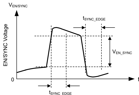
图 7-2. 应用于 EN/SYNC 的典型同步波形
