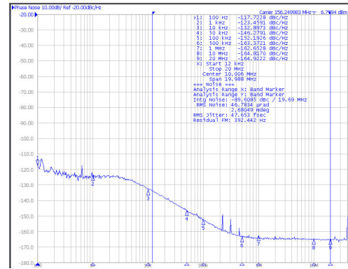
图 6-9. BAW APLL 的 156.25MHz HSDS 输出
