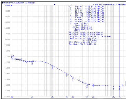
图 6-8. BAW APLL 的 312.5MHz HSDS 输出
