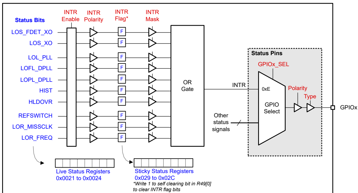
图 8-22. 状态和中断
