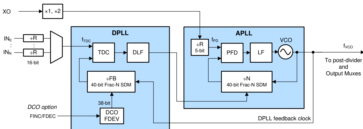
图 8-23. PLL 架构
