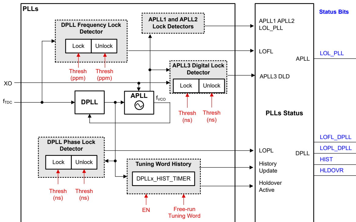
图 8-20. PLL 锁定检测器和历史记录监控器
