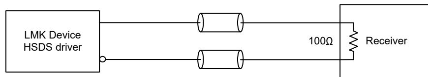
图 8-27. 直流耦合 HSDS/LVDS 输出终端
