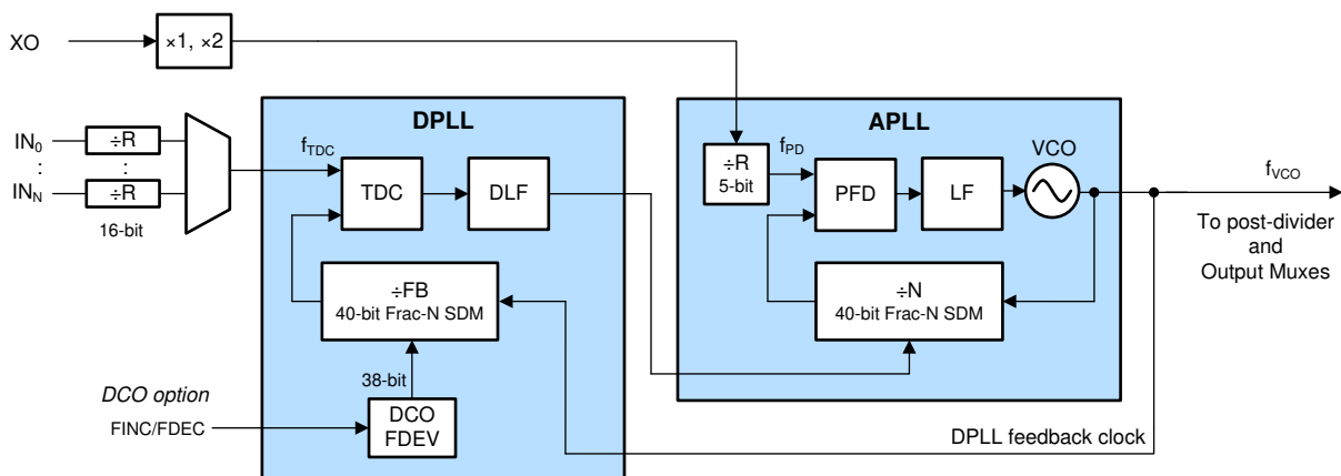
图 8-23. PLL 架构
