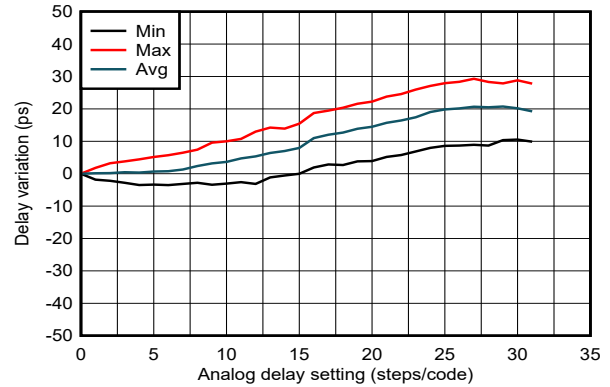
图 6-21. SYSREF/1PPS 延迟线性度与模拟延迟代码 2
