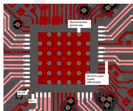
图 9-6. LMK5B33216 的 PCB 布局示例，顶层
