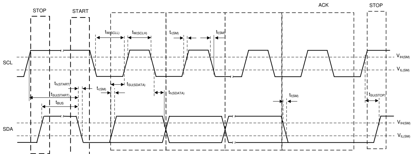
图 6-4. I²C 时序图
