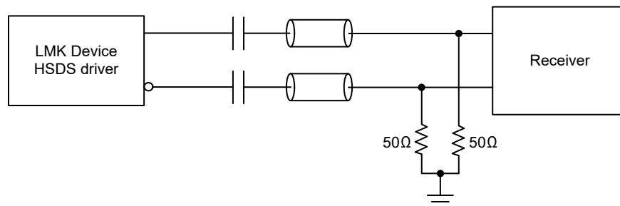
图 8-29. 交流耦合 HSDS 输出端接方法 2
