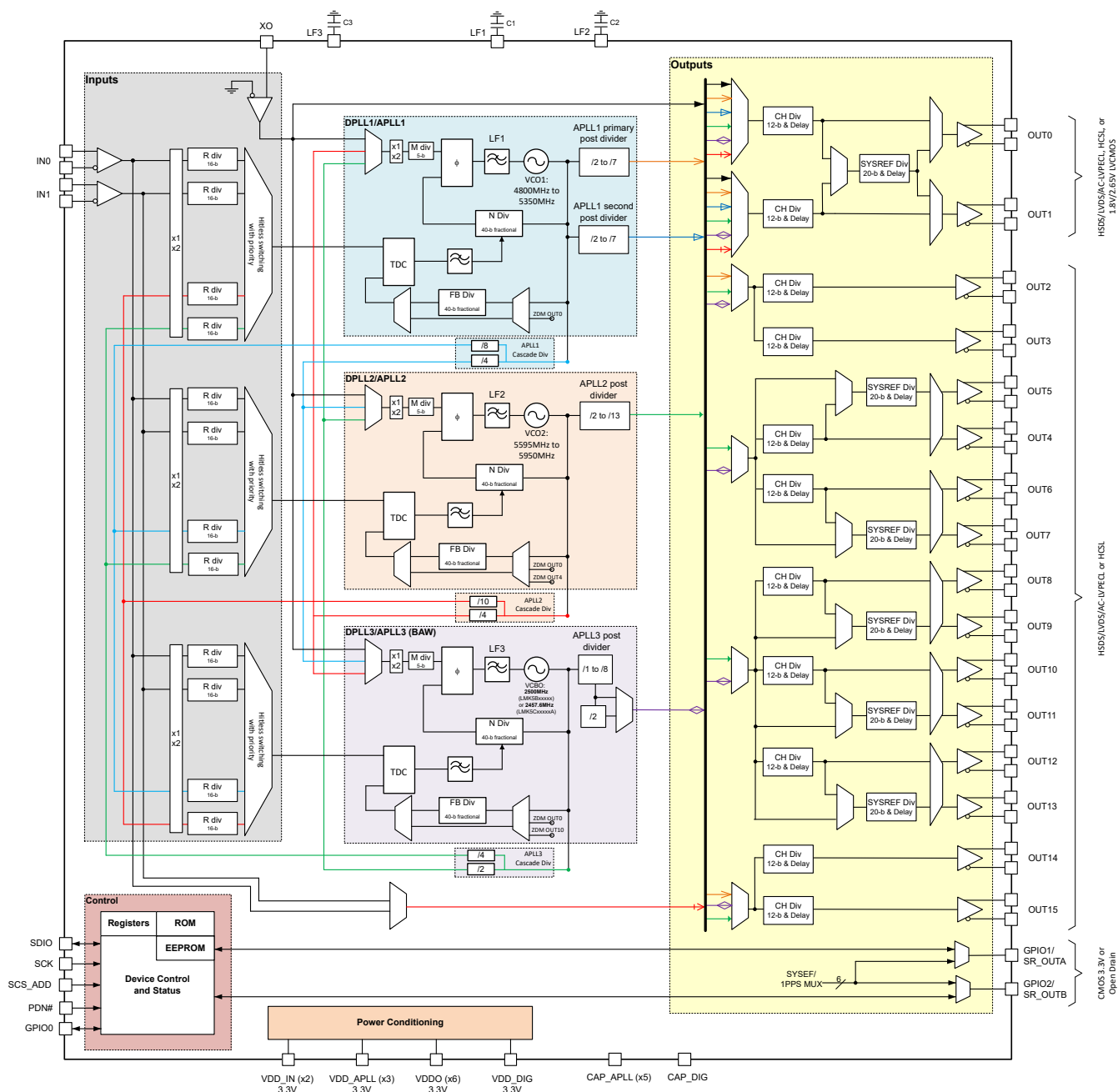
图 8-1. LMK5B33216 顶层方框图
