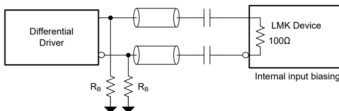
图 8-15. 交流耦合差分至基准 (INx)
