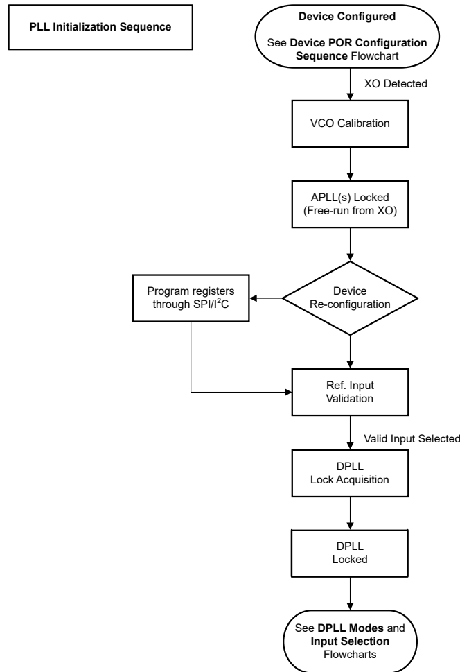
图 8-42. APLL 初始化序列
