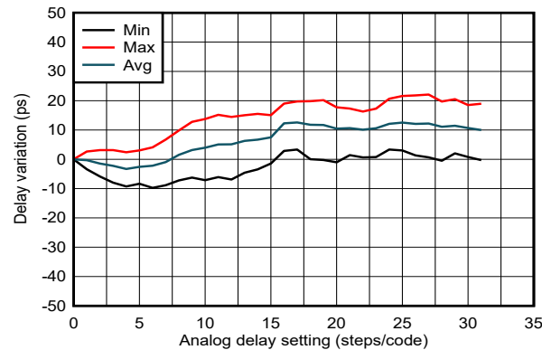
图 6-24. SYSREF/1PPS 延迟线性度与模拟延迟代码 5
