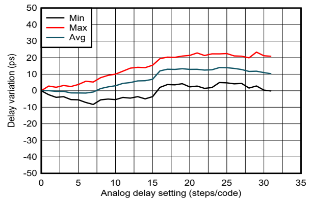
图 6-23. SYSREF/1PPS 延迟线性度与模拟延迟代码 4
