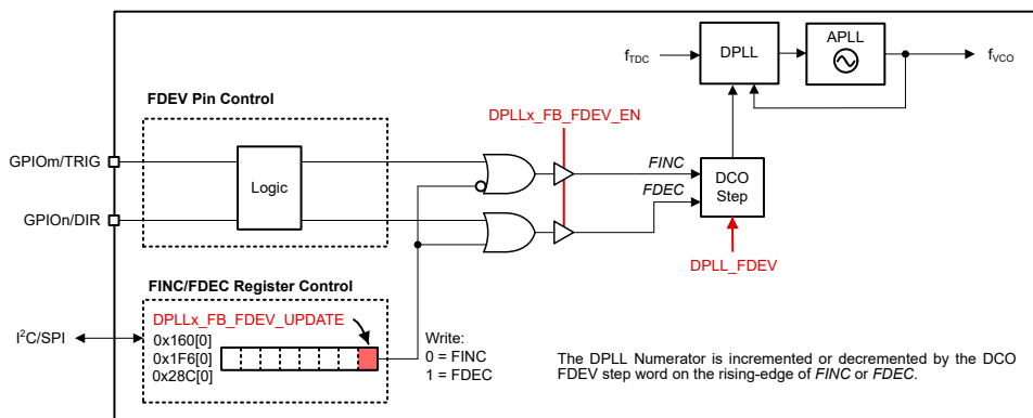
图 8-39. DCO 模式控制选项
