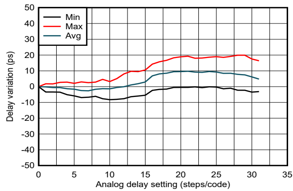
图 6-22. SYSREF/1PPS 延迟线性度与模拟延迟代码 3
