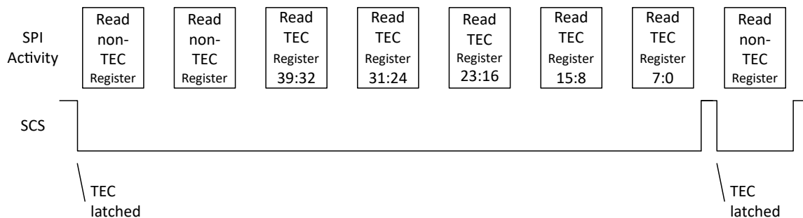
图 8-36. TEC 多字节读取
