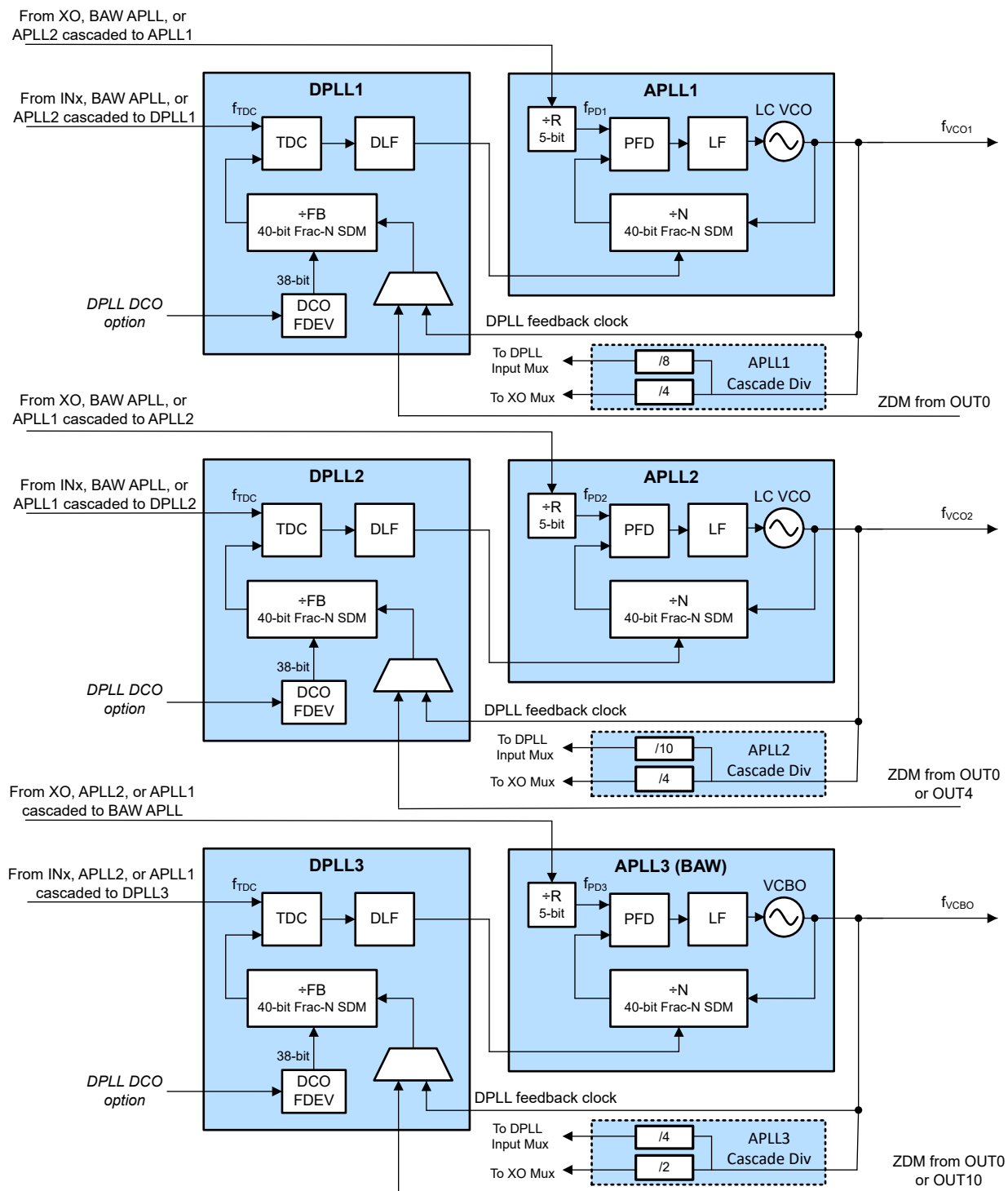
图 8-2. PLL 架构
