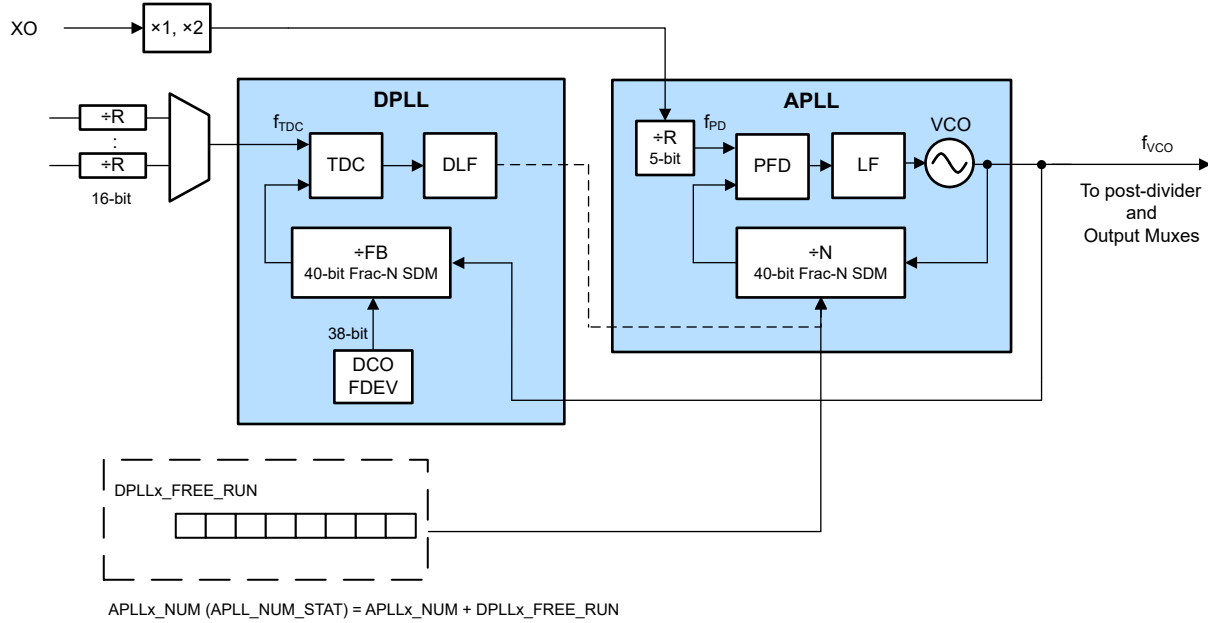
图 8-40. APLL DCO 模式
