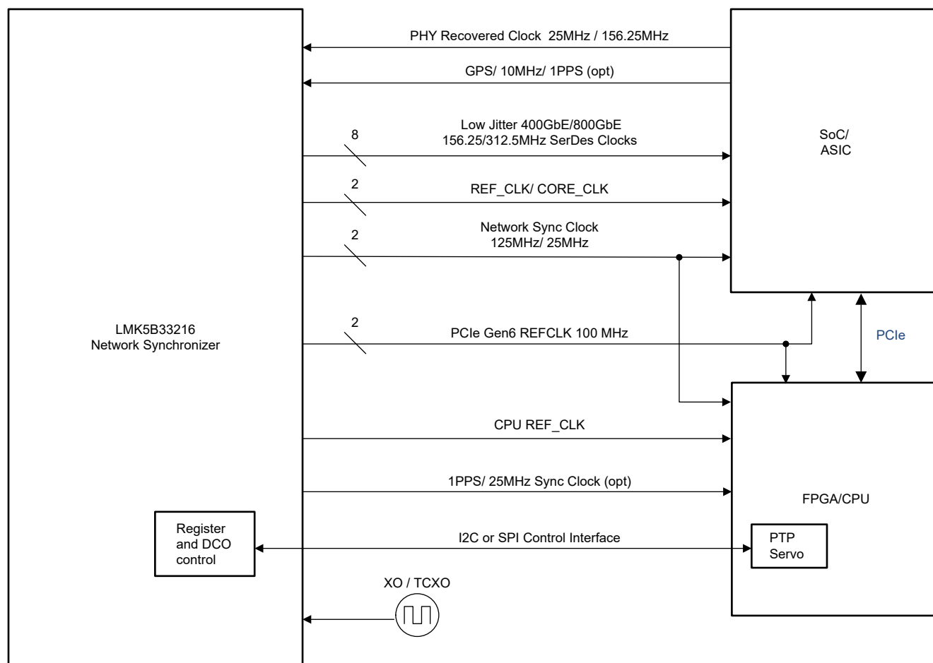
LMK5B33216 典型系统方框图
