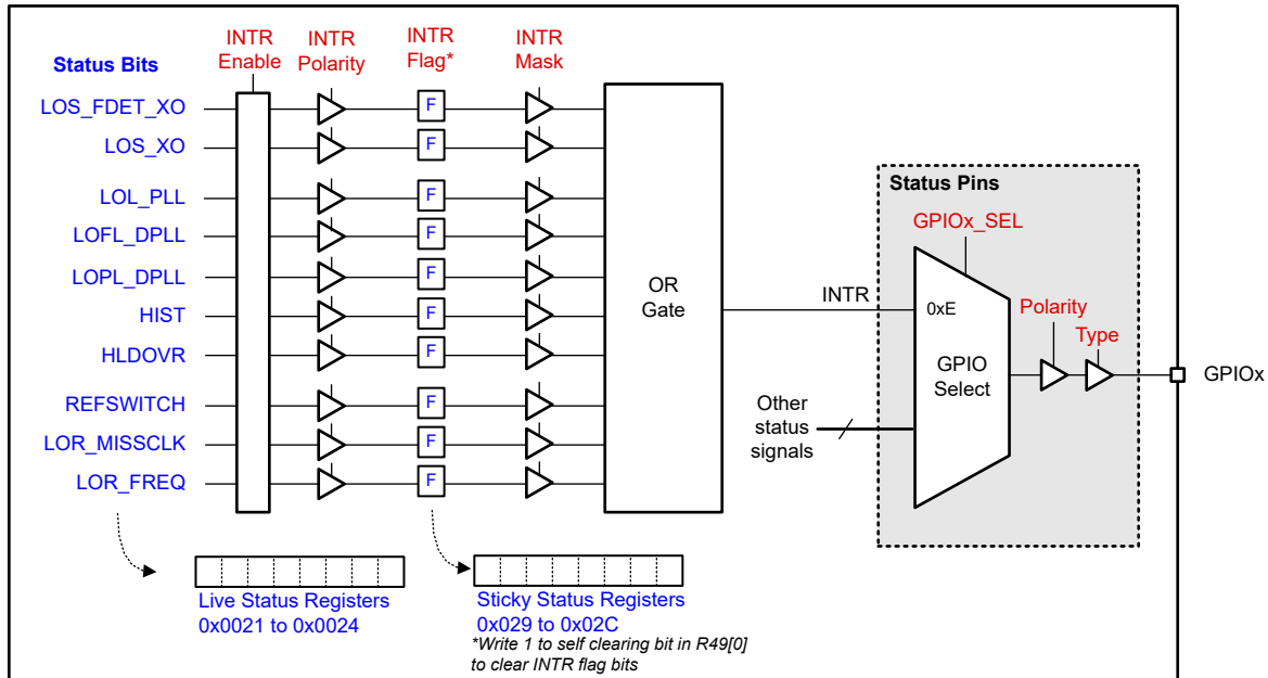
图 8-22. 状态和中断
