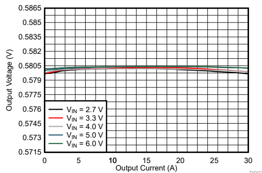
图 10-3. 输出电压与输出电流间的关系
