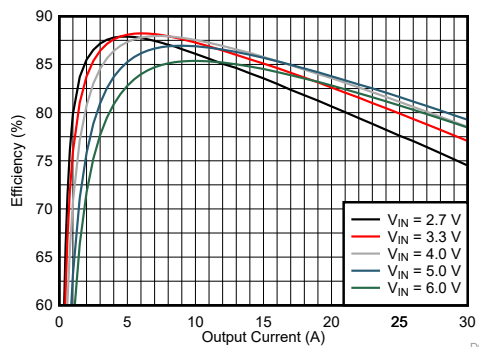
图 10-2. 效率与输出电流之间的关系
