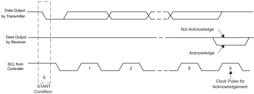
图 8-19. I 2 C 总线上的确认
