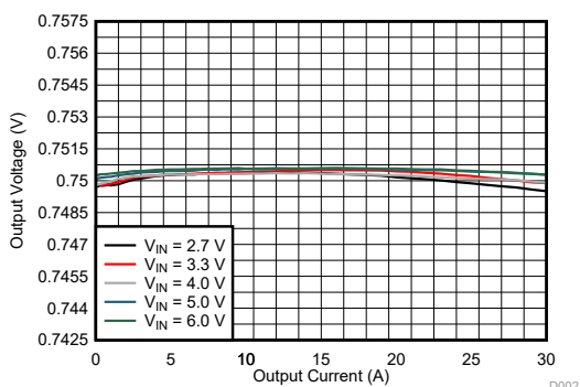
图 10-4. 输出电压与输出电流间的关系
