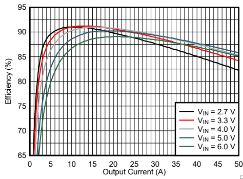
图 10-21. 效率与输出电流之间的关系
