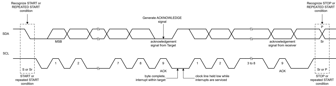
图 8-20. 总线协议
