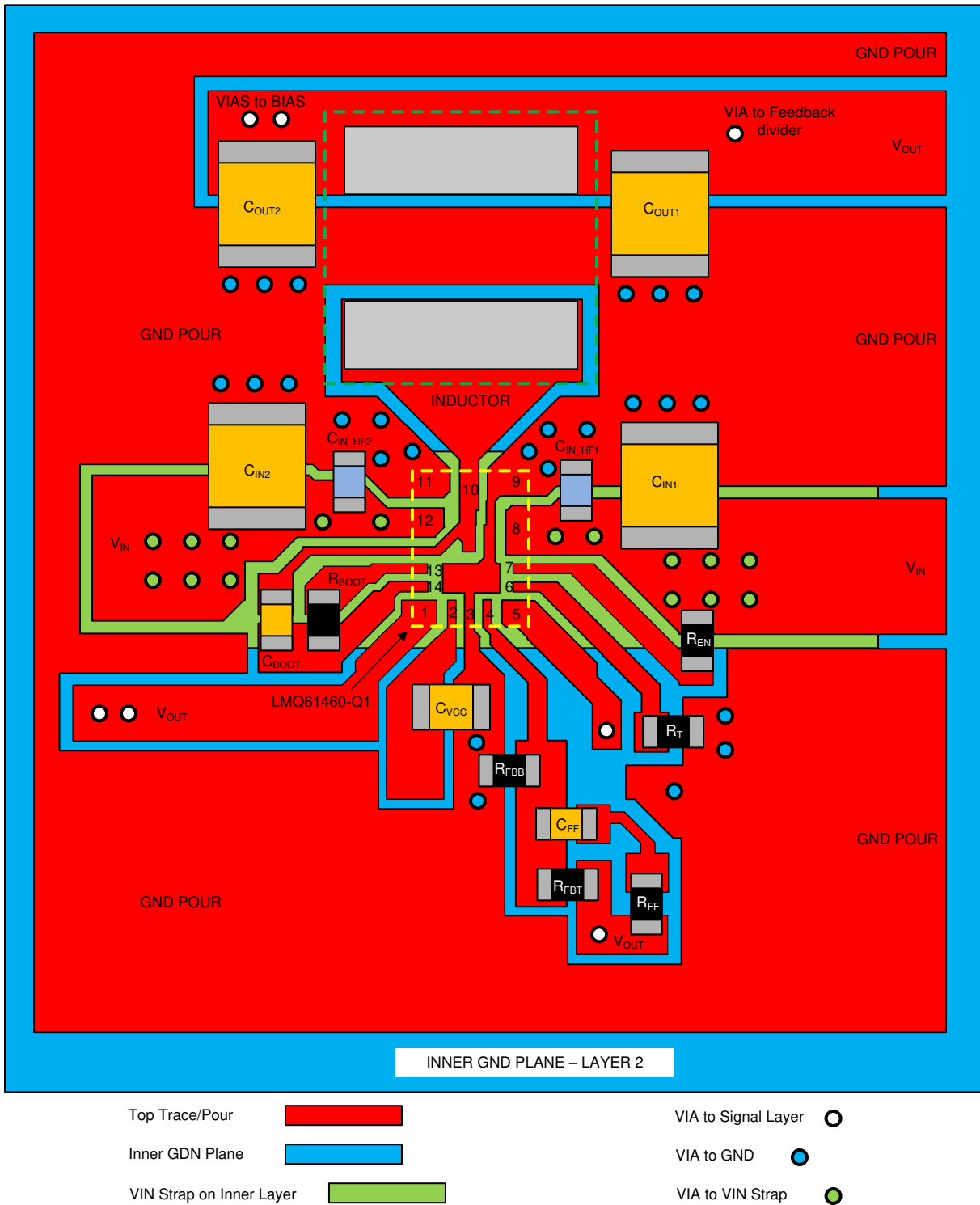
图 8-63. 布局示例
