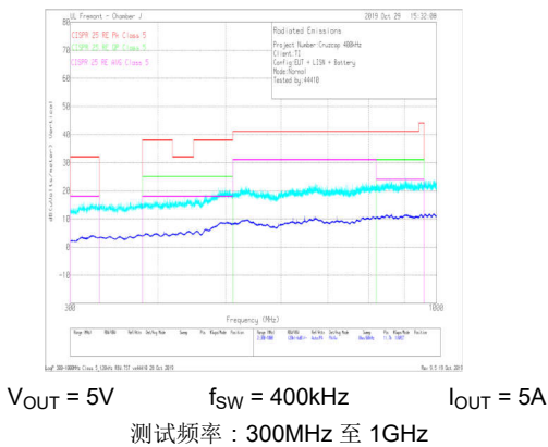
图 8-51. 辐射 EMI 对数垂直与 CISPR25 限值
