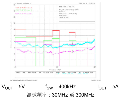
图 8-49. 辐射 EMI 双锥垂直与 CISPR25 限值
