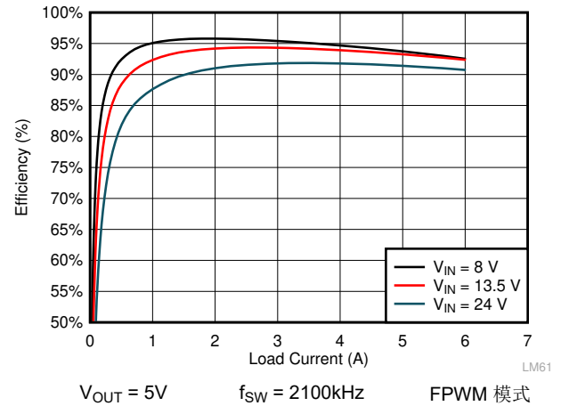
图 8-12. LMQ61460 效率
