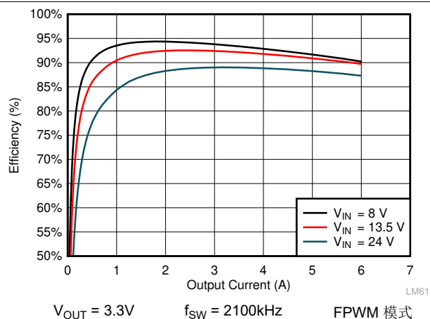
图 8-8. LMQ61460 效率
