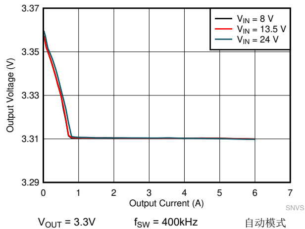
图 8-13. LMQ61460 负载和线性调整率
