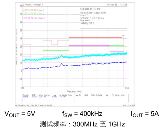
图 8-52. 辐射 EMI 对数水平与 CISPR25 限值
