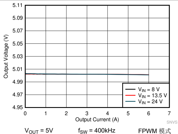
图 8-18. LMQ61460 负载和线性调整率
