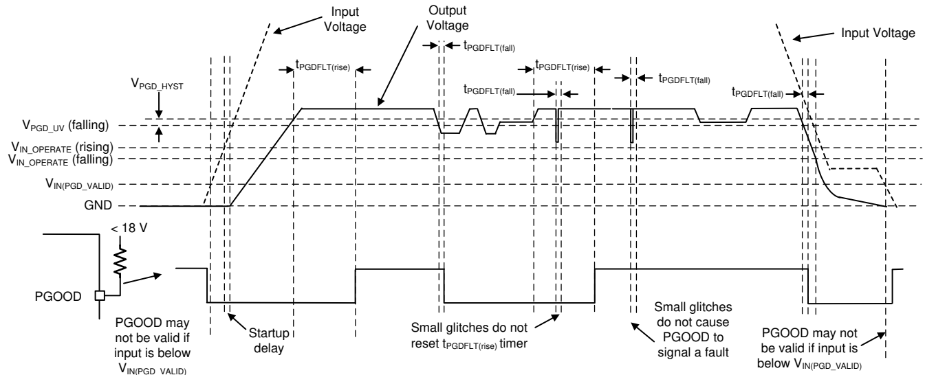
图 7-6. PGGOOD 时序图 (不包括 OV 事件)
