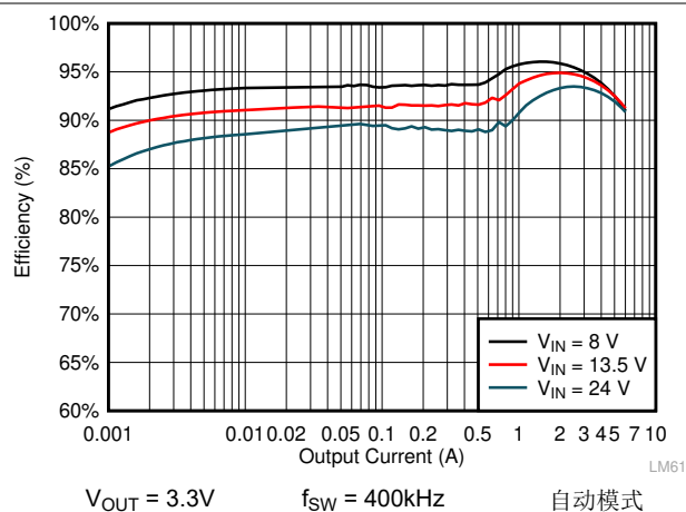
图 8-5. LMQ61460 效率
