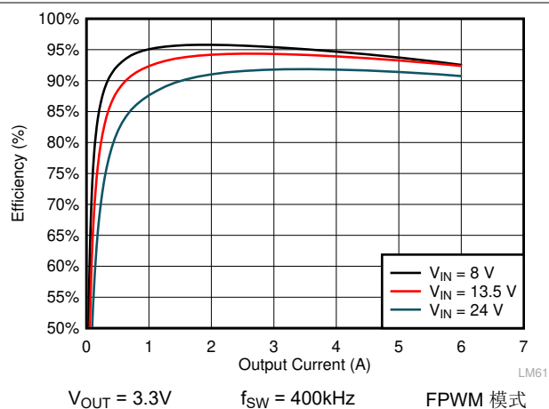
图 8-6. LMQ61460 效率
