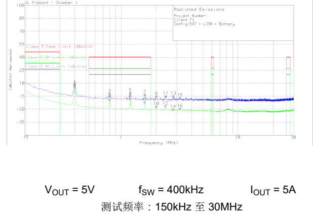
图 8-48. 辐射 EMI 杆状与 CISPR25 限值
