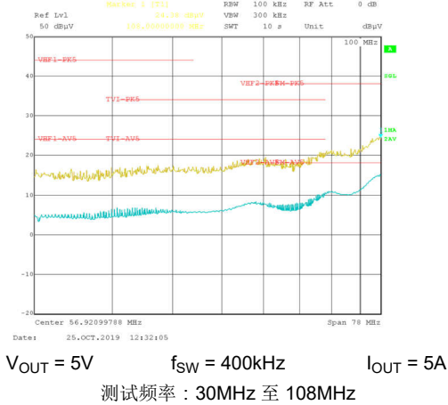
图 8-47. 传导 EMI 与 CISPR25 限值 (黄色：峰值信号，蓝色：平均信号)
