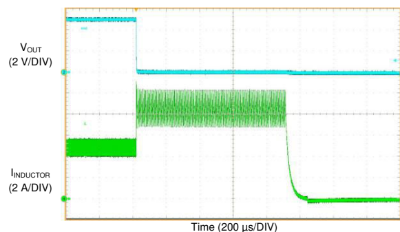
图 8-32. 在 50mA 负载下启动 LMQ61460
