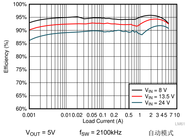
图 8-11. LMQ61460 效率
