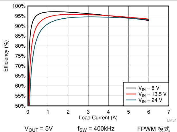
图 8-10. LMQ61460 效率
