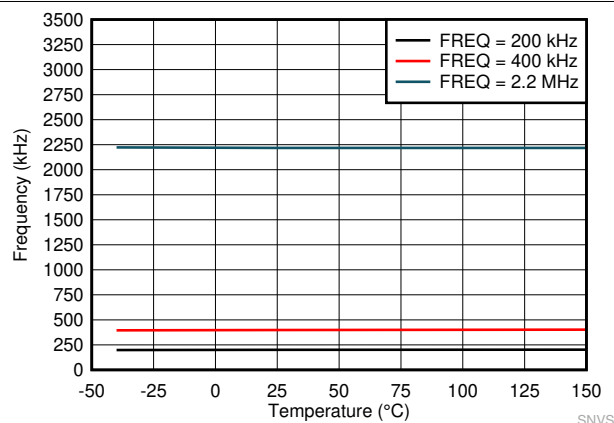
图 6-5. 开关频率
