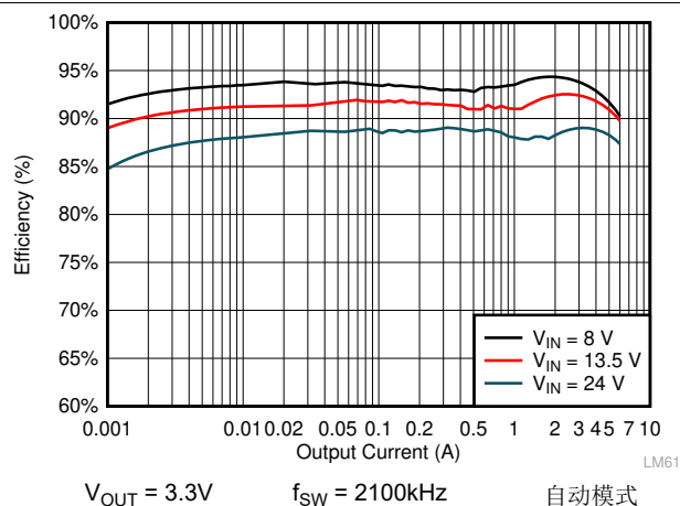
图 8-7. LMQ61460 效率
