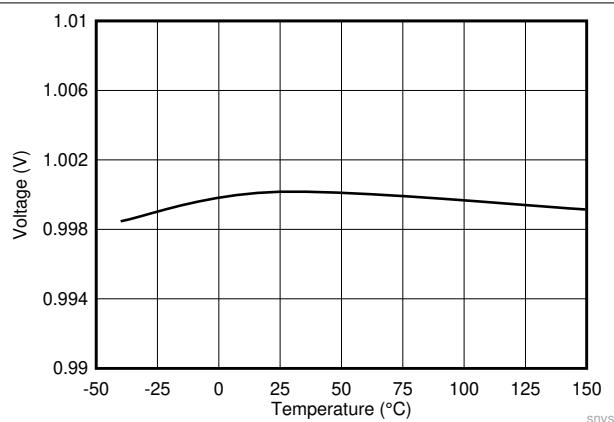
图 6-3. 反馈电压
