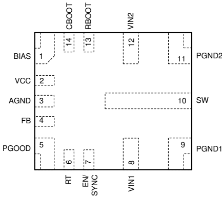
图 5-1. RJR 封装 14 引脚 VQFN-HR 顶视图
