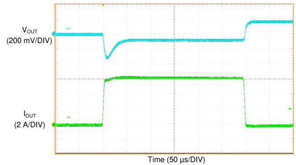
图 8-42. LMQ61460 负载瞬态
