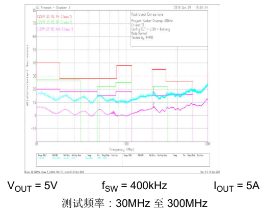
图 8-50. 辐射 EMI 双锥水平与 CISPR25 限值
