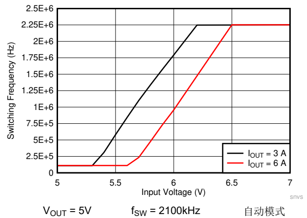
图 8-28. LMQ61460 压降曲线
