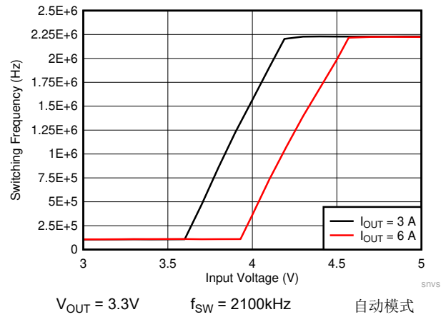
图 8-26. LMQ61460 压降曲线
