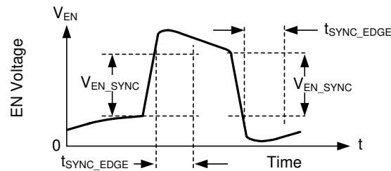
图 7-3. 典型 SYNC/EN 波形
