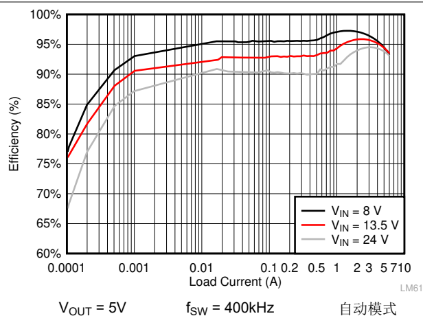
图 8-9. LMQ61460 效率
