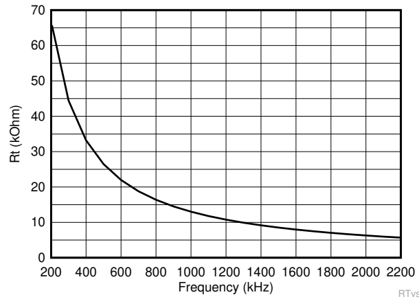
图 7-4. 设置时钟频率
