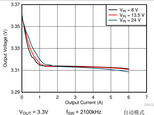
图 8-15. LMQ61460 负载和线性调整率
