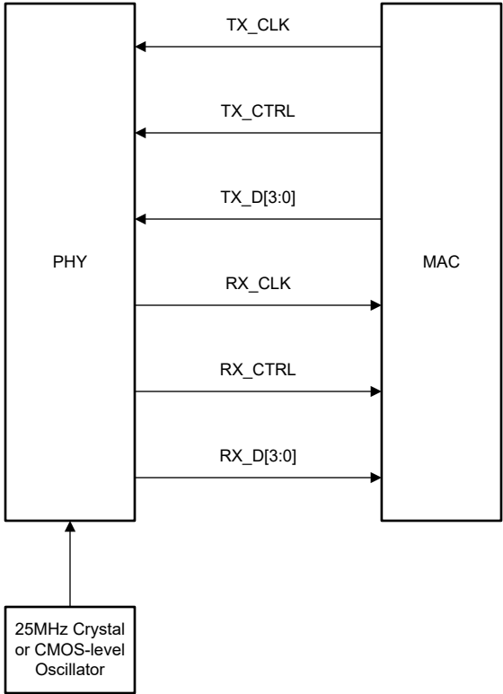
图 7-13. RGMII 连接
