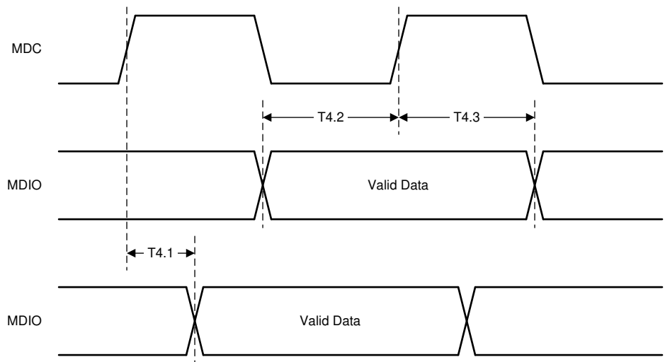
图 6-6. 串行管理时序
