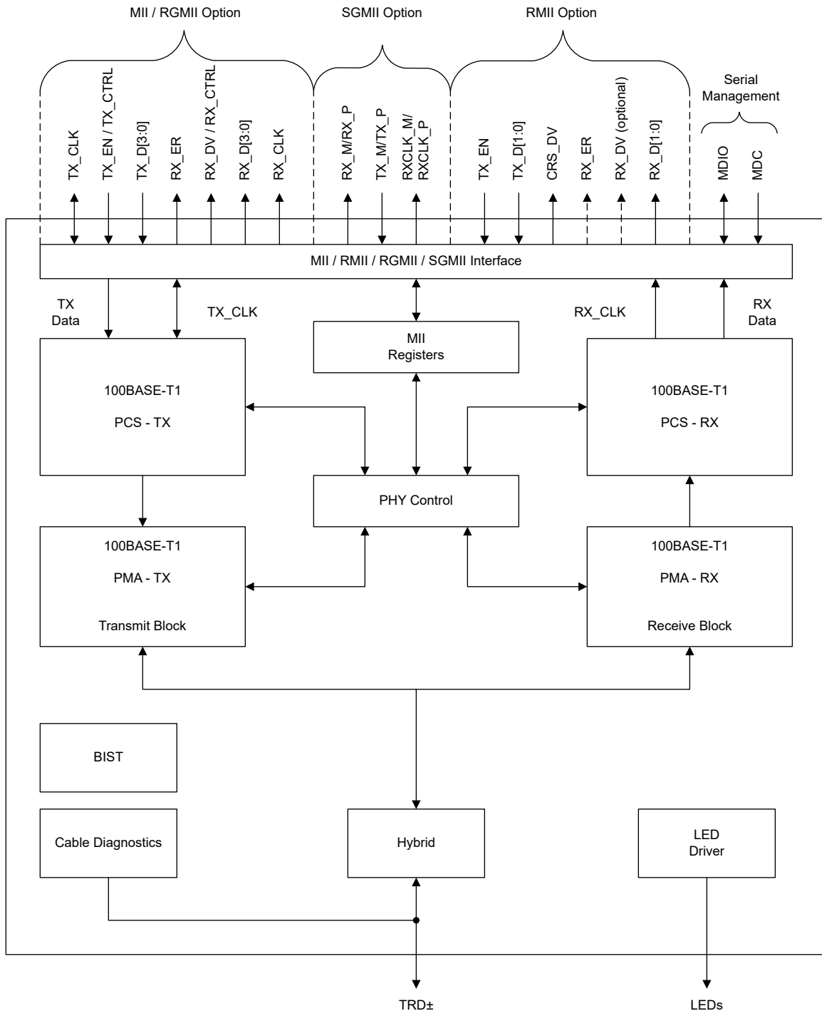
图 7-1. DP83TC814S-Q1
