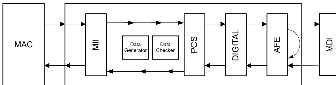
图 7-8. 不带数据生成器的模拟环回
