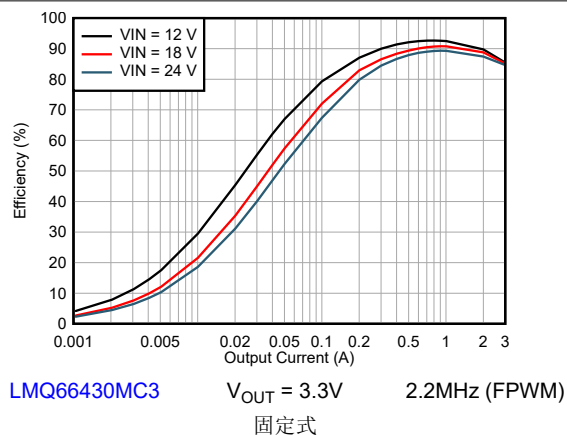
图 8-5. 效率
