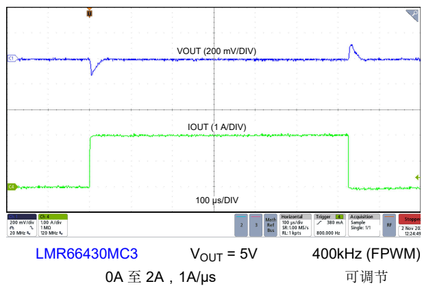
图 8-31. 负载瞬态
