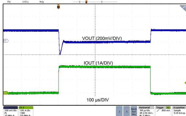
LMQ66430MC3 V_{OUT} = 3.3V 2.2MHz (自动) 0A 至 2A, 1A/μs 固定式
