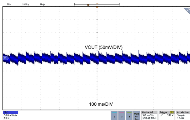
LMQ66430MC3 V_{OUT} = 3.3V 无负载 固定式
