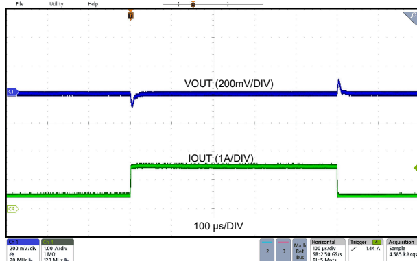
LMQ66430MC3 V_{OUT} = 3.3V 2.2MHz (自动) 0.5A 至 1.5A, 1A/μs 固定式
