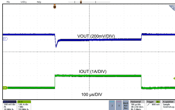
LMQ66430MC3 V_{OUT} = 3.3V 2.2MHz (自动) 0A 至 1A, 1A/μs 固定式
