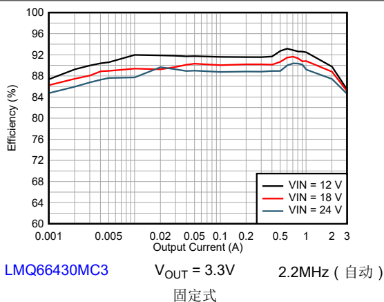
图 8-4. 效率
