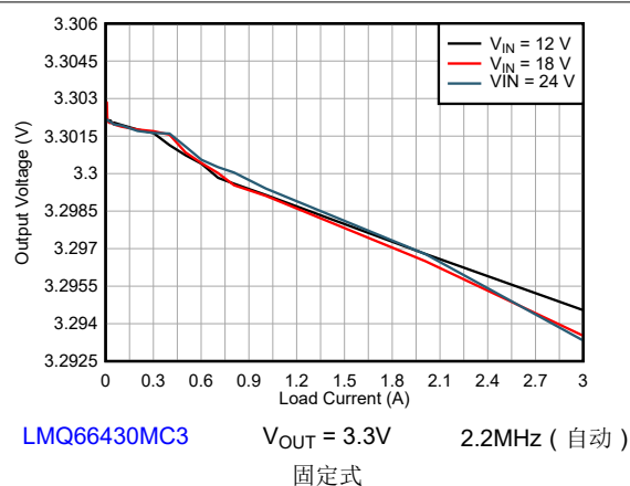
图 8-7. 线性 and 负载调整率
