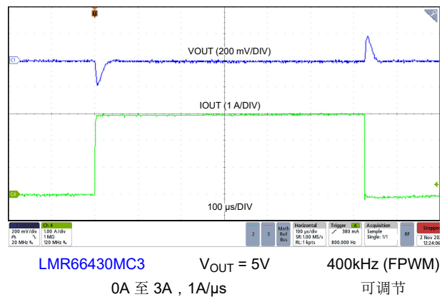
图 8-30. 负载瞬态
