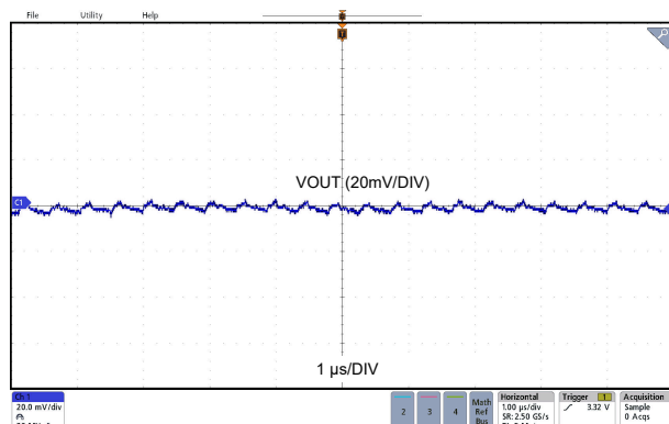
LMQ66430MC3 V_{OUT} = 3.3V 2A 负载 固定式
