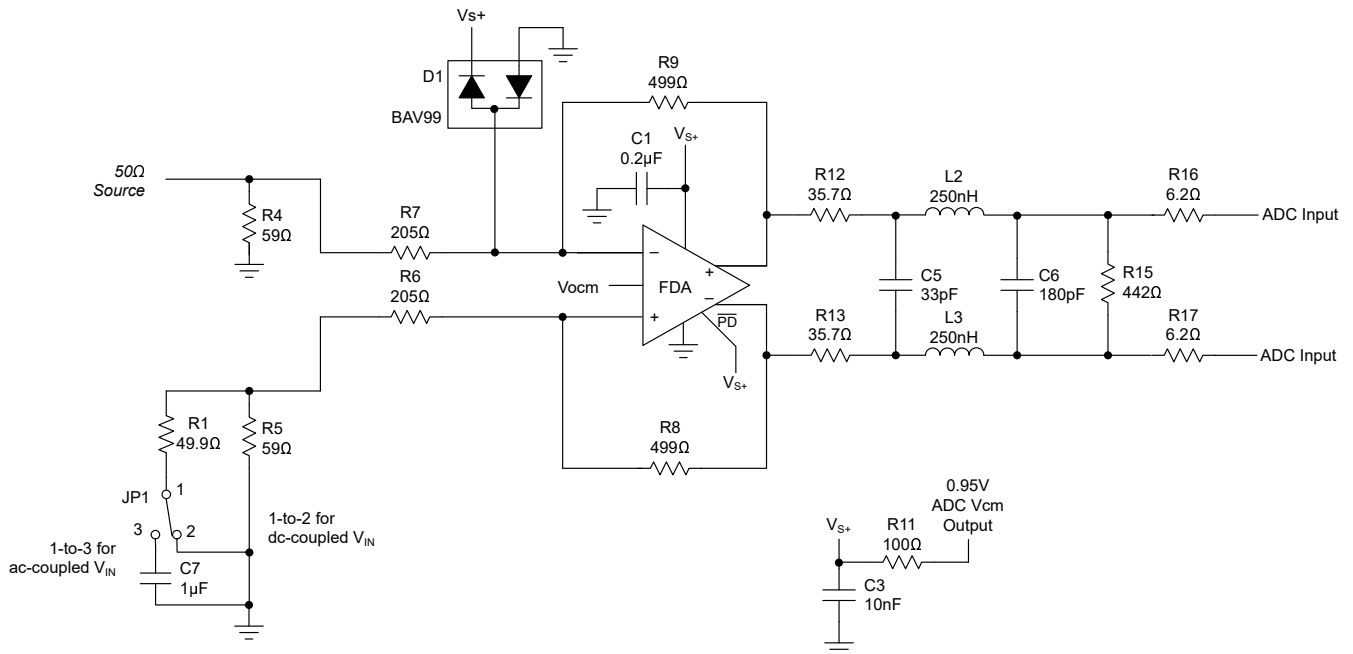
图 9-1. 用于连接 ADC 的直流耦合、双极输入、2V/V 增益单端至差分接口
