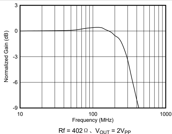
图 6-6. 大信号频率响应
