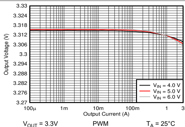
图 9-11. 输出电压与输出电流间的关系
