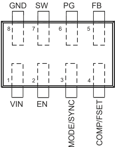
图 5-2. TPS62850x-Q1 的 8 引脚 SOT583 DYC 封装 (俯视图)
