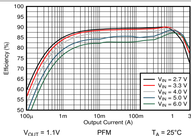
图 9-6. 效率与输出电流之间的关系
