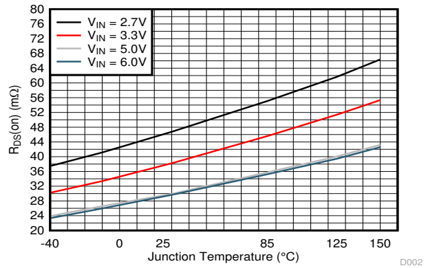
图 6-2. 低侧开关的 R_{DS(ON)}
