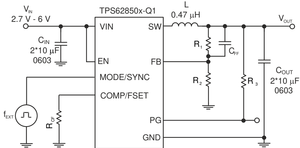
图 9-58. 使用外部同步的原理图
