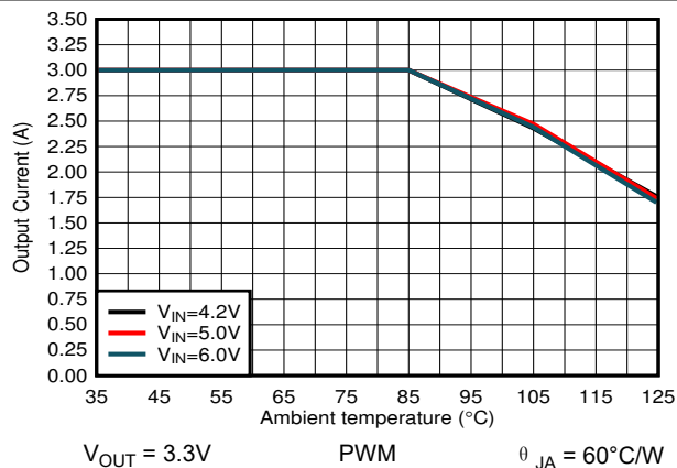
图 9-21. 输出电流与环境温度间的关系
