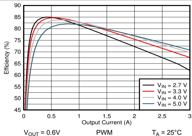
图 9-9. 效率与输出电流之间的关系
