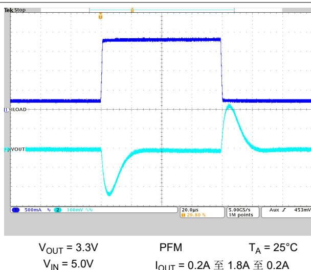
图 9-22. 负载瞬态响应
