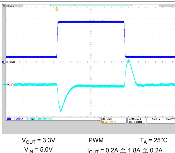
图 9-23. 负载瞬态响应
