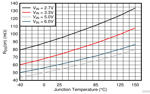
图 6-1. 高侧开关的 R_{DS(ON)}
