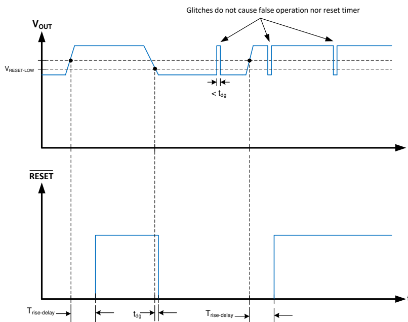
图 7-5. RESET 时序行为
