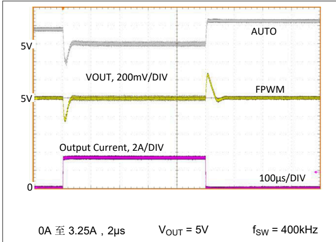
图 8-20. 负载瞬态
