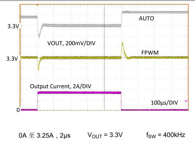
图 8-21. 负载瞬态
