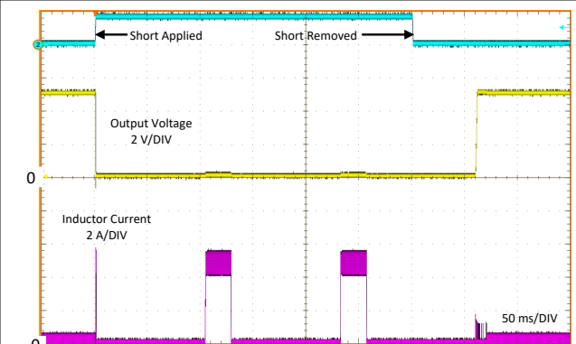
图 7-13. 短路瞬态和恢复
