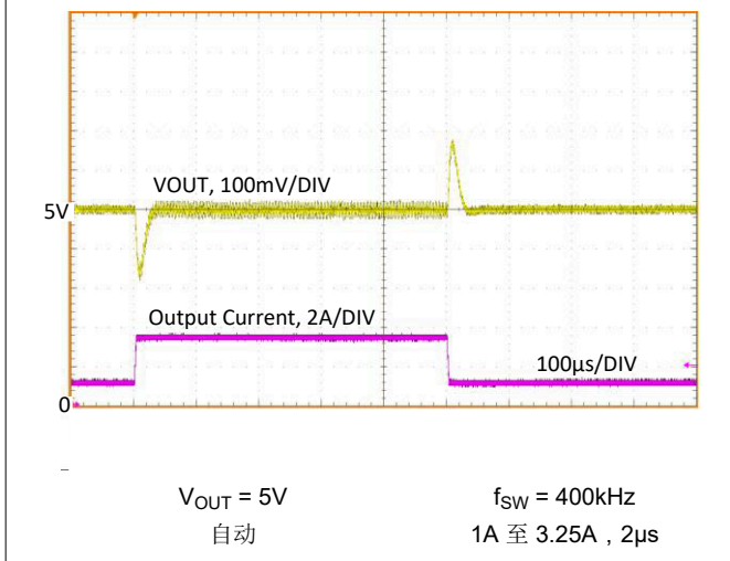
图 8-24. 负载瞬态
