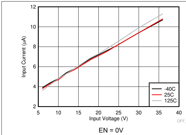
图 6-1. 关断模式下的输入电源电流
