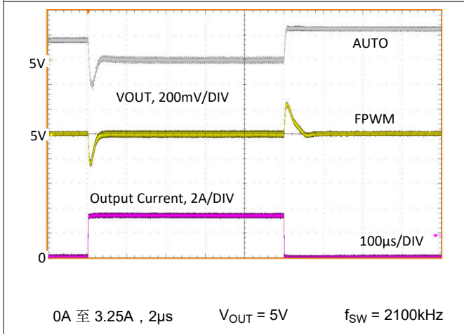
图 8-22. 负载瞬态
