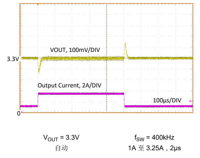
图 8-25. 负载瞬态
