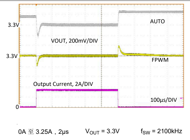
图 8-23. 负载瞬态
