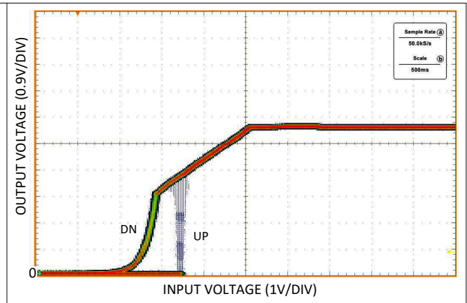
图 6-2. UVLO 阈值
