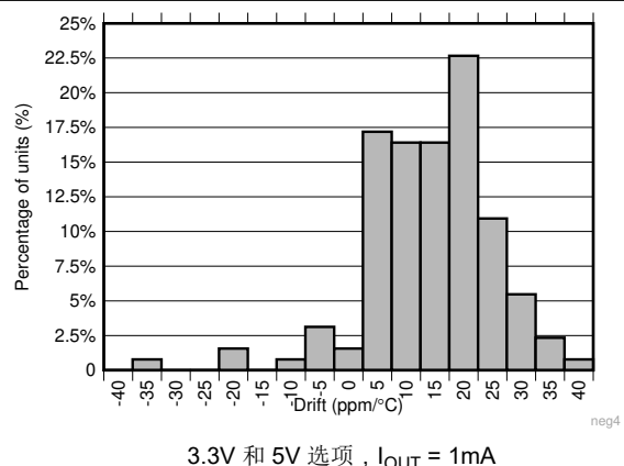
图 5-10. 温漂直方图 (-40°C 至 +25°C)
