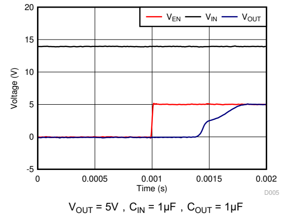
图 5-18. 通过使能启动
