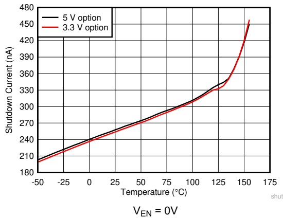
图 5-1. 关断电流与环境温度间的关系
