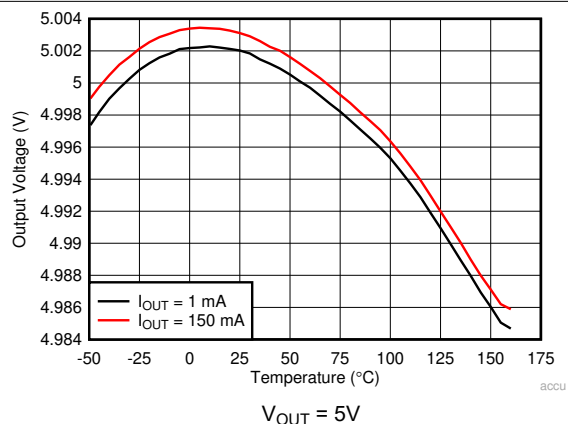
图 5-8. 输出电压与环境温度间的关系
