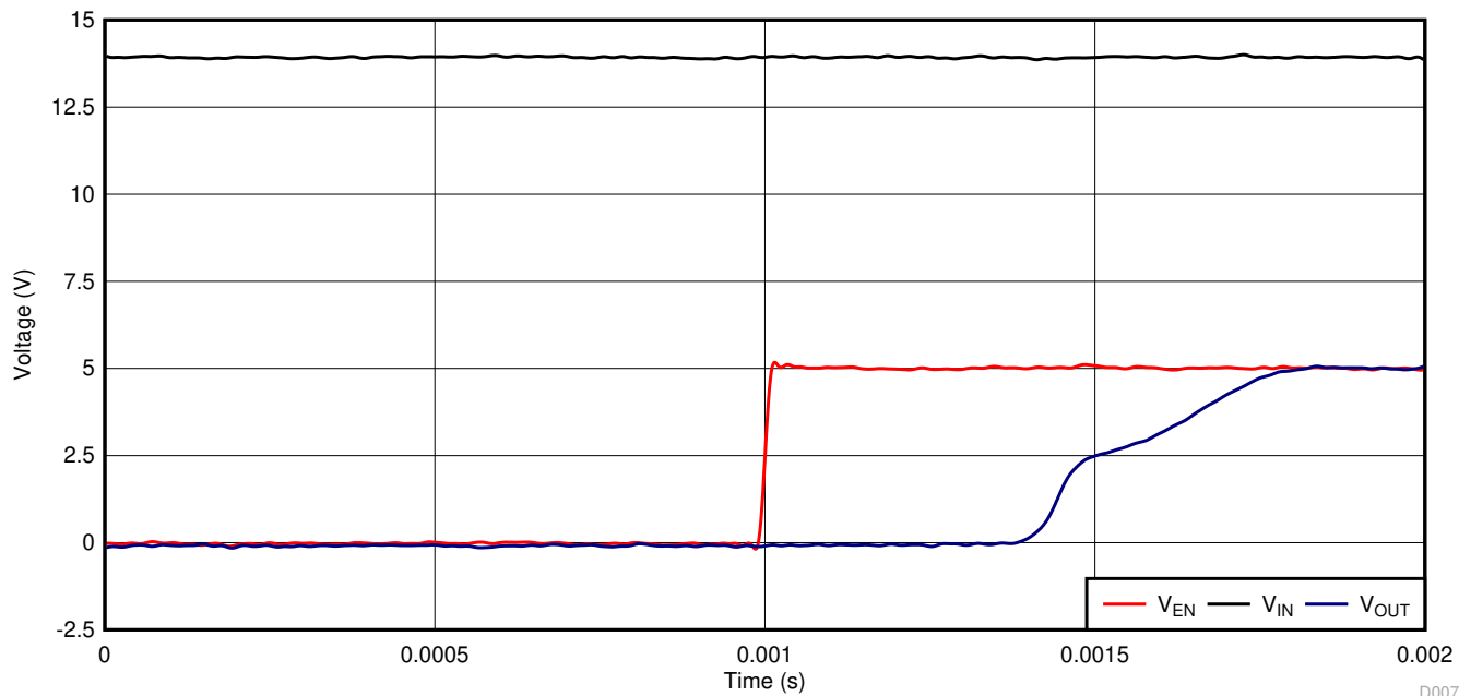
图 7-8. TPS7B81-Q1 加电波形 (5V)
