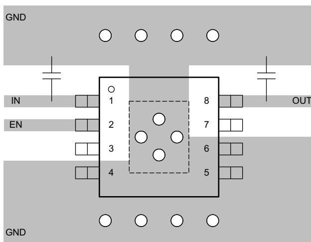
图 7-9. TPSB81-Q1 示例布局图
