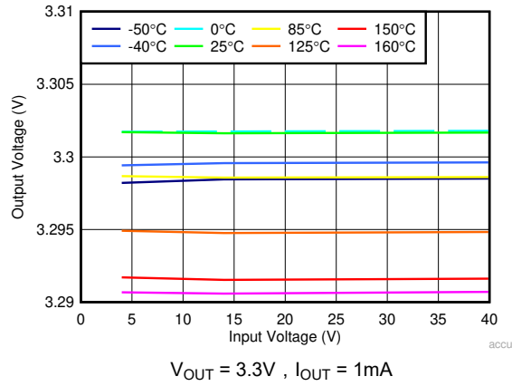
图 5-13. 输出电压与输入电压间的关系
