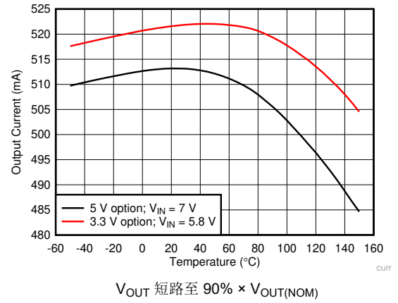
图 5-14. 输出电流限制与环境温度
