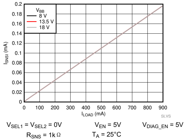
图 6-17. V_{BB} 上的电流感应输出电流 ( I_{SNSI} ) 与负载电流 ( I_{OUT} ) 间的关系
