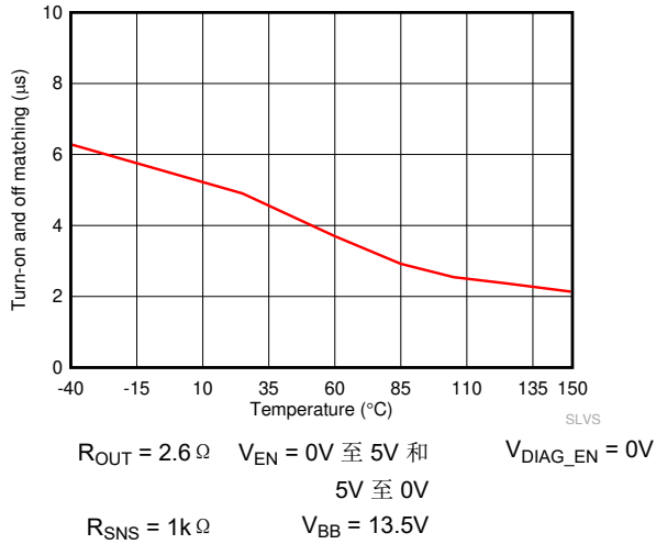
图 6-15. 导通和关断匹配 ( t_{ON} - t_{OFF} ) 与温度间的关系
