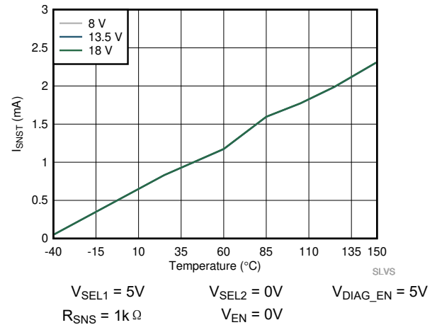
图 6-18. 温度感应输出电流 ( I_{SNST} ) 与温度间的关系
