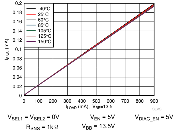
图 6-16. 整个温度范围内电流感应输出电流 ( I_{SNSI} ) 与负载电流 ( I_{OUT} ) 间的关系
