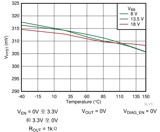
图 6-26. V_{IHYS} 与温度间的关系
