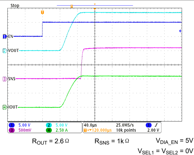
图 6-29. 导通时间 ( t_{ON} )
