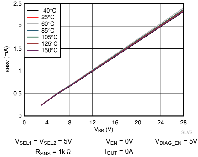
图 6-19. 电压感应输出电流 ( I_{SNSV} ) 与 V_{BB} 间的关系
