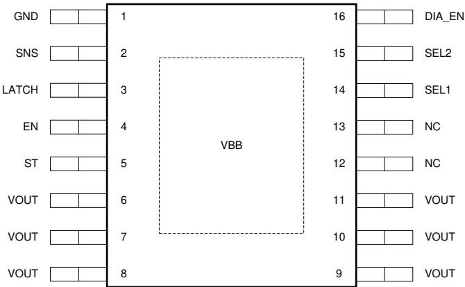
图 5-1. PWP 封装 16 引脚 HTSSOP 顶视图
