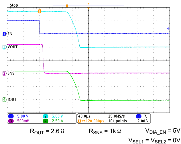
图 6-30. 关断时间 ( t_{OFF} ) 和感应趋稳时间 ( t_{SNSION2} )
