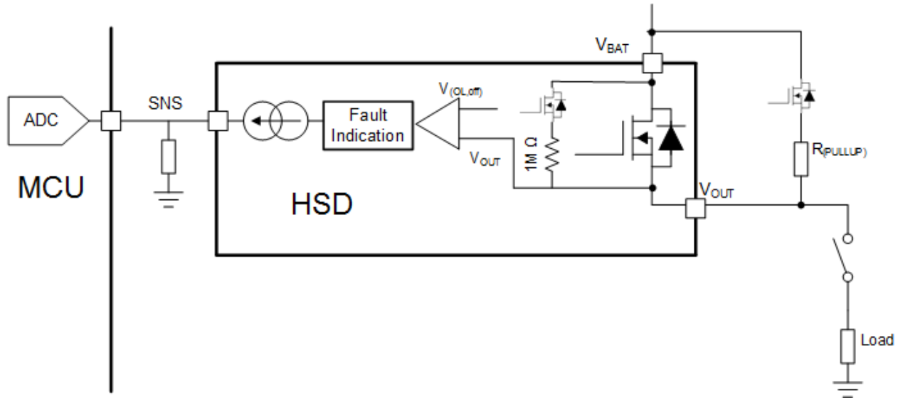
图 8-10. 电池短路和开路负载检测
