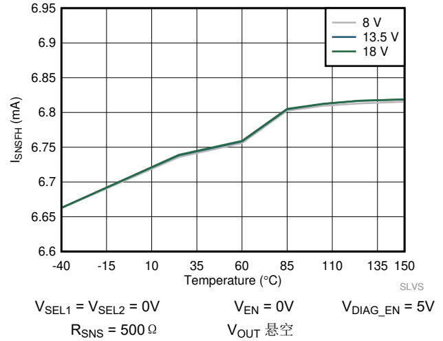
图 6-20. 故障高电平输出电流 ( I_{SNSFH} ) 与温度间的关系
