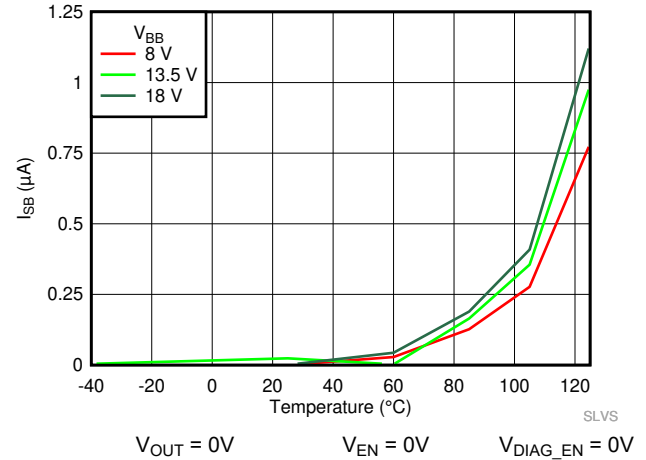
图 6-4. 待机电流 ( I_{SB} ) 与温度间的关系
