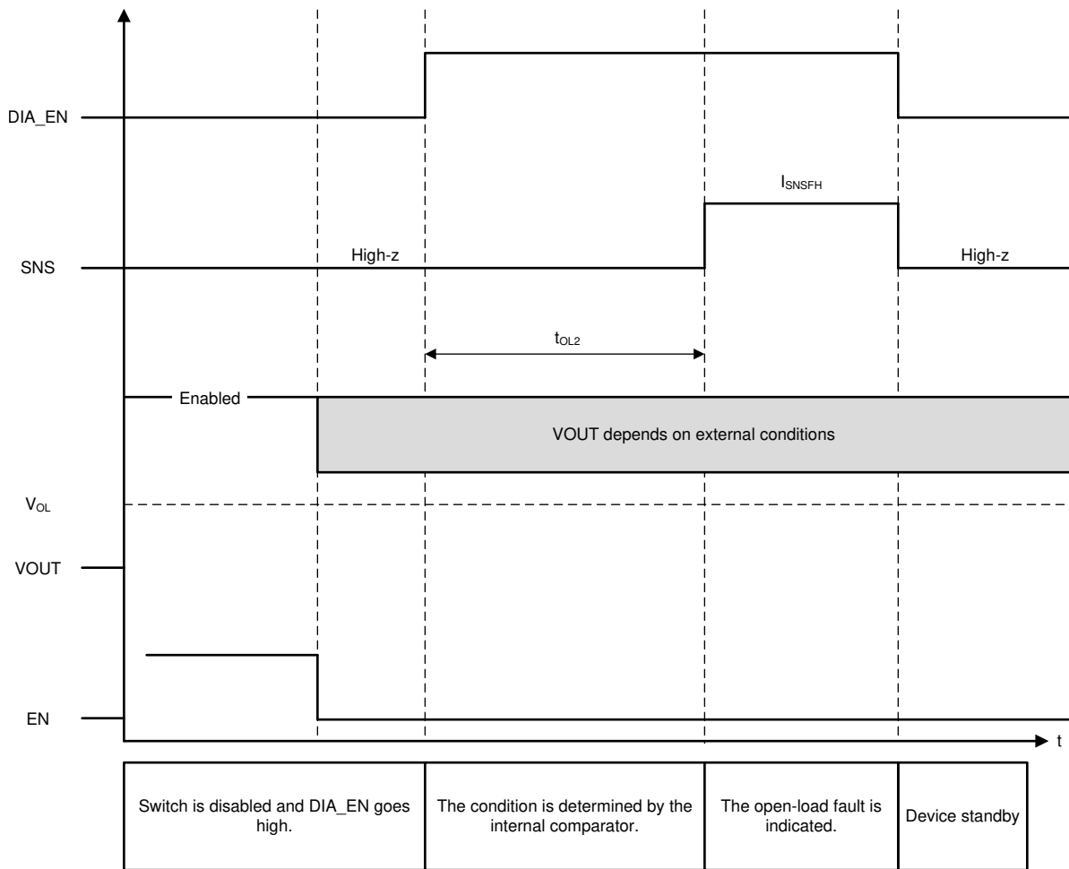
图 8-11. 开路负载
