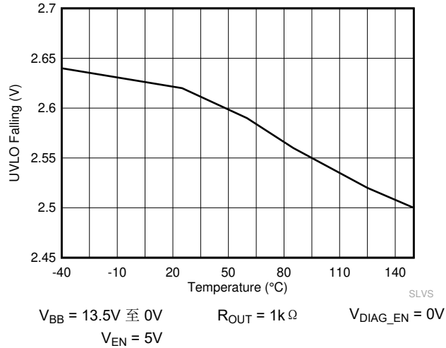
图 6-3. 下降欠压锁定 ( V_{UVLOF} ) 与温度间的关系
