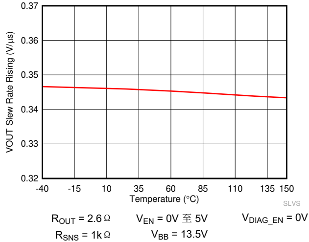
图 6-11. V_{OUT} 转换率上升 ( SR_R ) 与温度间的关系
