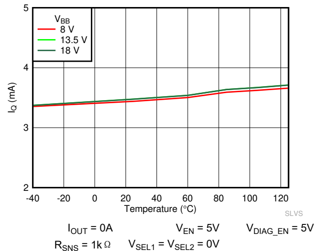
图 6-6. 静态电流 ( I_Q ) 与温度间的关系
