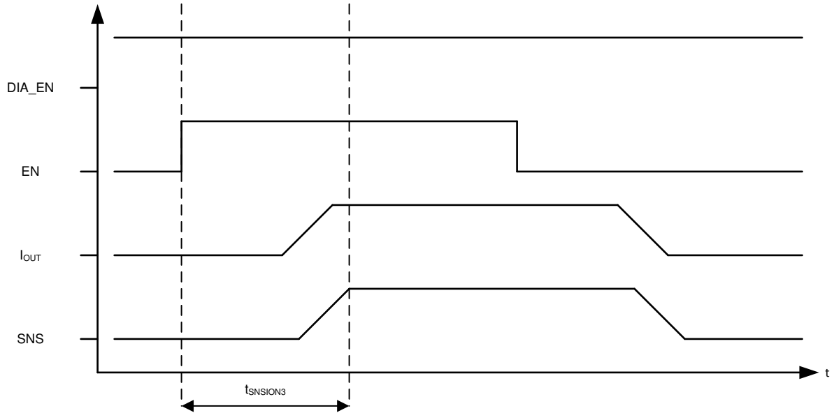
图 8-13. 低占空比应用中的电流检测
