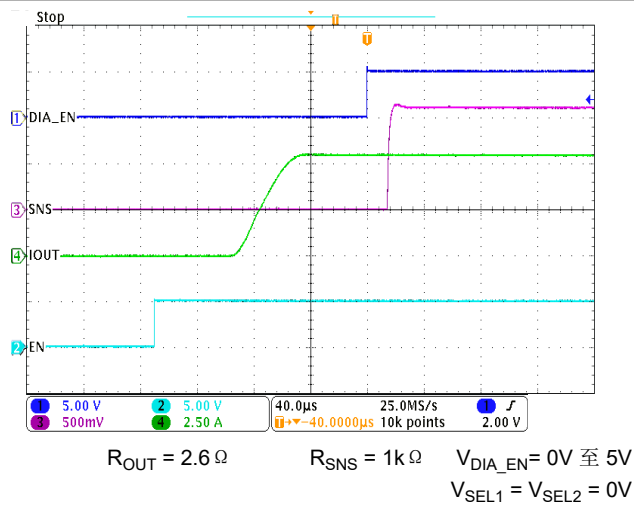
图 6-31. DIA_EN 切换时的 I_{SNS} 趋稳时间 ( t_{SNSION1} )
