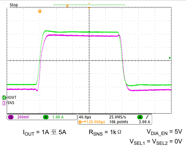
图 6-32. 上升负载阶跃上的 I_{SNS} 趋稳时间 ( t_{SETTLEH} )
