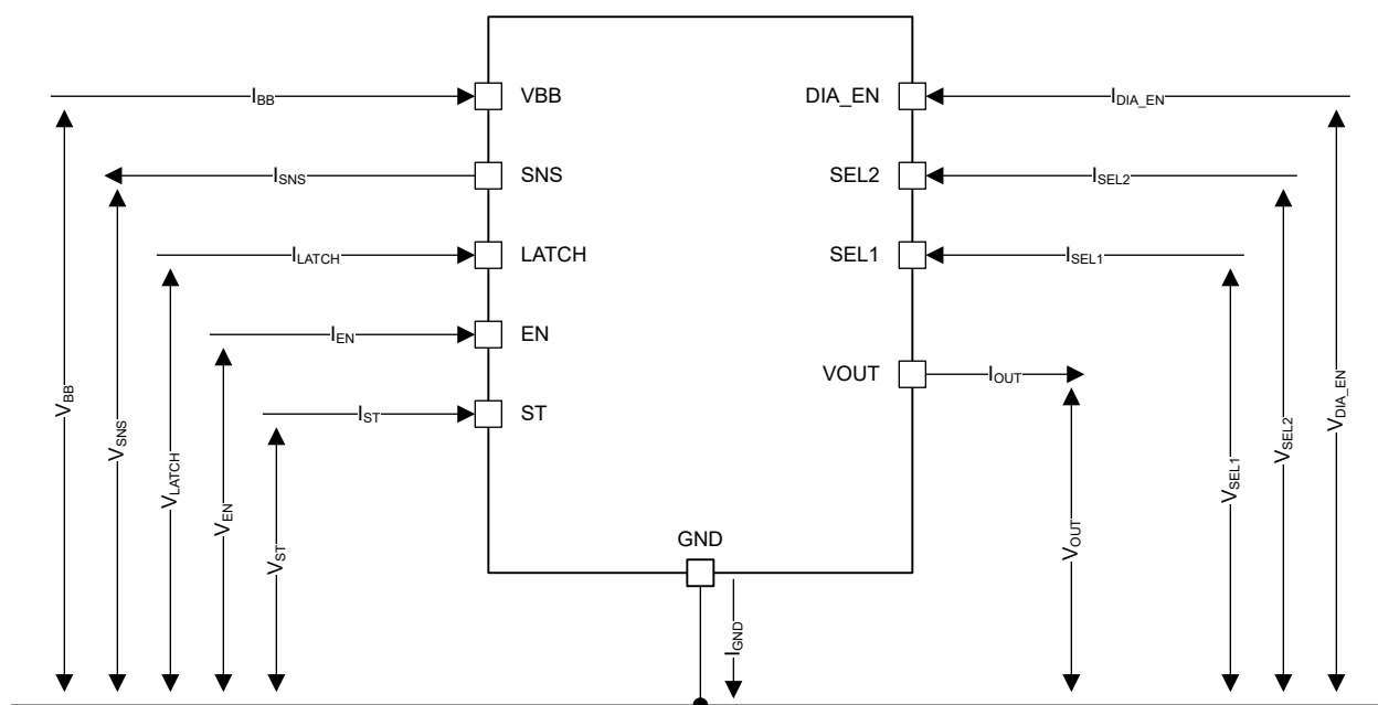
图 7-1. 参数定义
