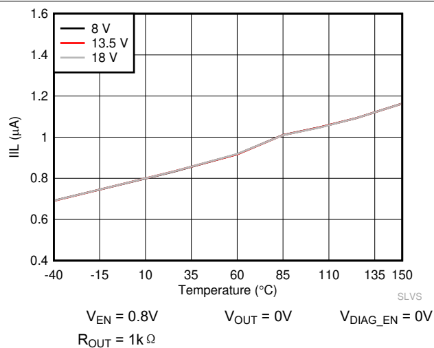
图 6-27. I_{IL} 与温度间的关系
