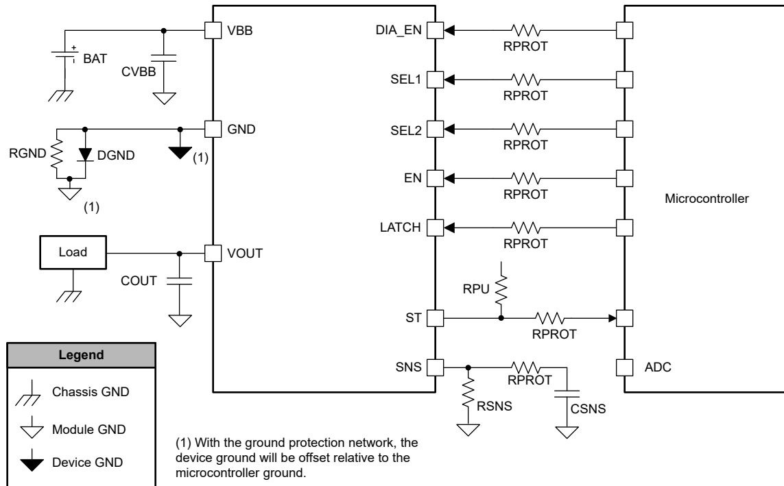
图 9-1. 系统图
