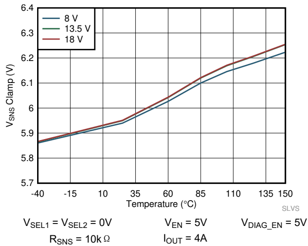
图 6-21. 感应引脚钳位电压 ( V_{SNSCLAMP} ) 与温度间的关系
