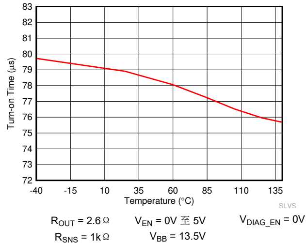
图 6-13. 导通时间 ( t_{ON} ) 与温度间的关系
