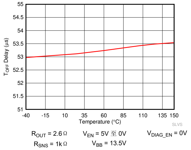
图 6-10. 关断延迟时间 ( t_{DF} ) 与温度间的关系
