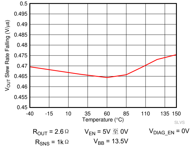
图 6-12. V_{OUT} 转换率下降 ( SR_F ) 与温度间的关系
