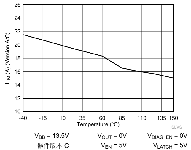
图 6-22. 电流限制 ( I_{CL} ) 与温度间的关系
