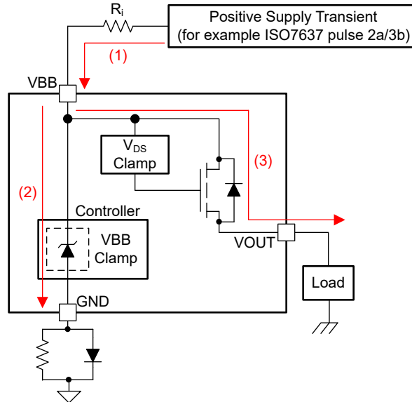
图 8-2. 电源电压瞬变期间的电流路径
