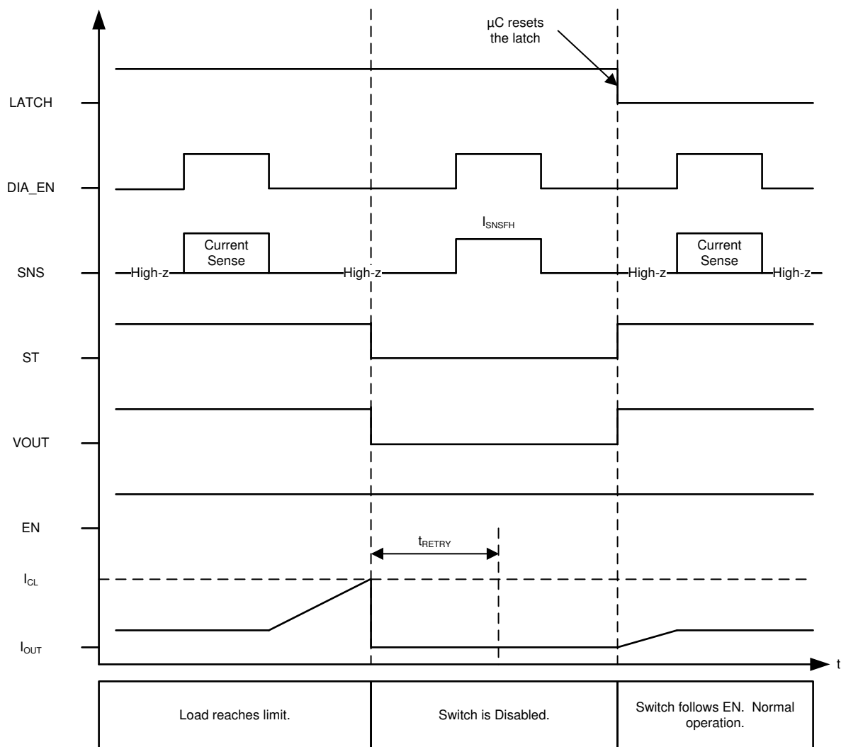
图 8-5. 电流限制 - 版本 A、B、E - 锁存行为
