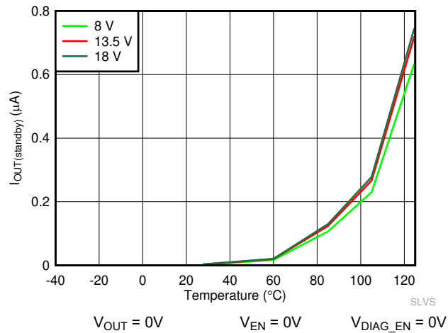
图 6-5. 输出泄漏电流 ( I_{OUT(standby)} ) 与温度间的关系
