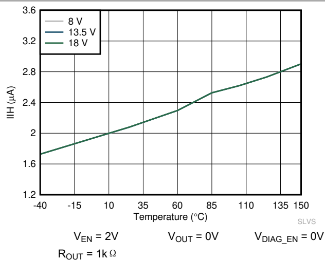
图 6-28. I_{IH} 与温度间的关系
