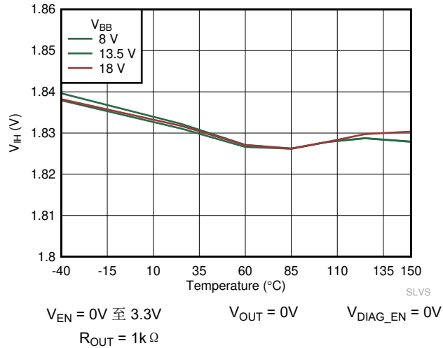
图 6-25. V_{IH} 与温度间的关系
