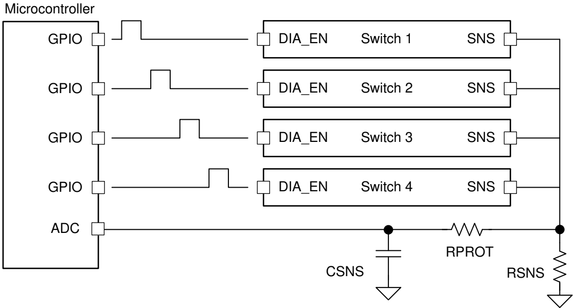
图 8-12. 在多个器件之间共享 R_{SNS}
