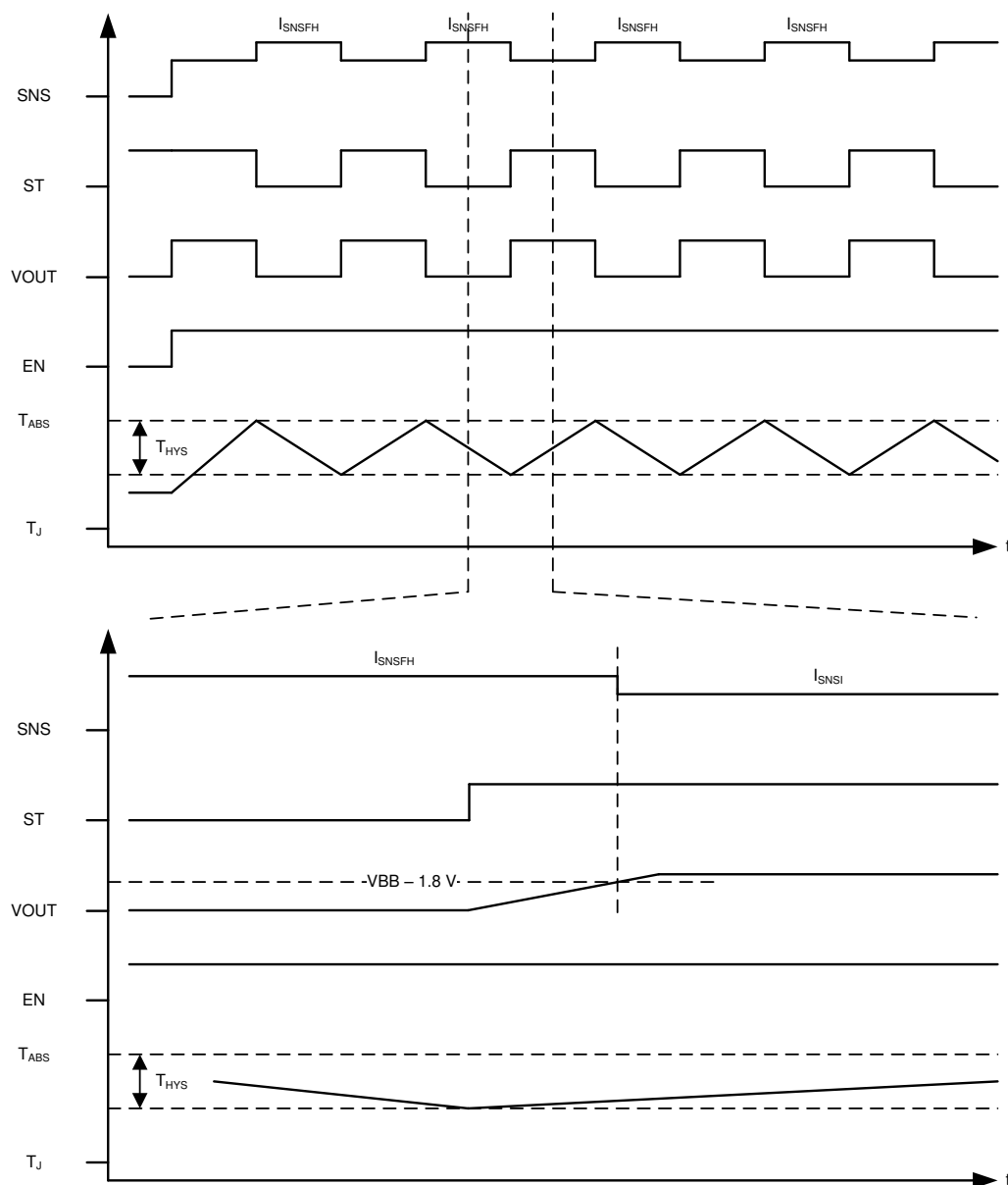
图 8-9. 重试期间的故障指示
