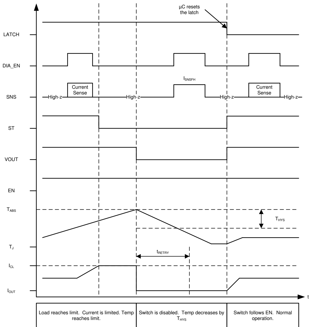
图 8-7. 电流限制 - 版本 C、D - 锁存行为
