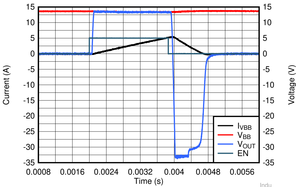
图 8-3. 感性放电 ( 5mH , 5A )
