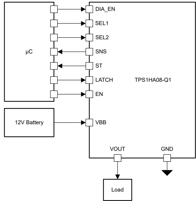
图 9-3. 为加热器负载供电的方框图
