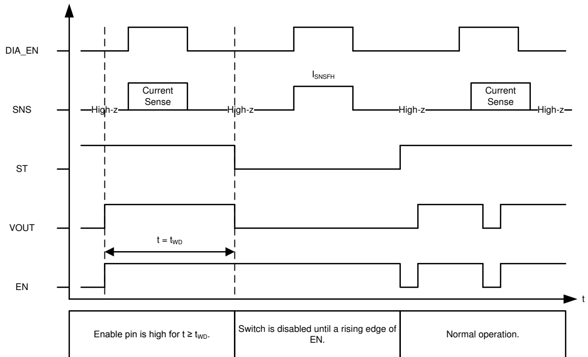
图 8-15. 使能看门狗时序图
