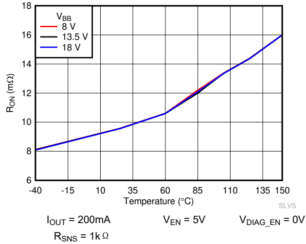
图 6-7. 导通电阻 ( R_{ON} ) 与温度间的关系
