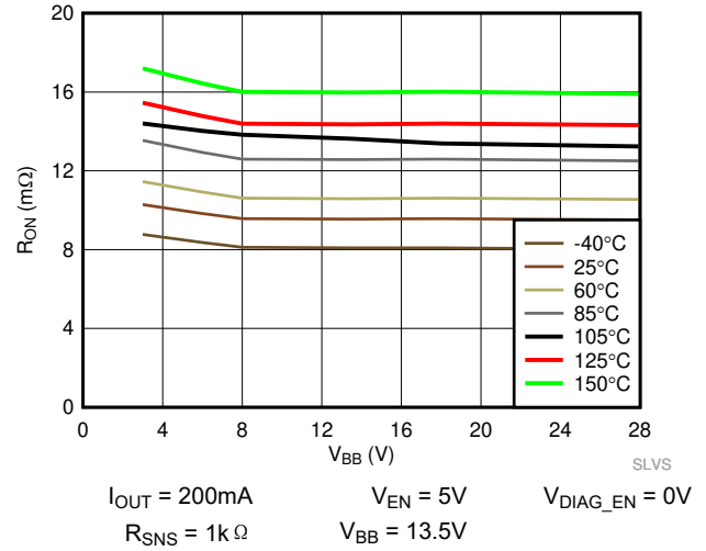
图 6-8. 导通电阻 ( R_{ON} ) 与 V_{BB} 间的关系
