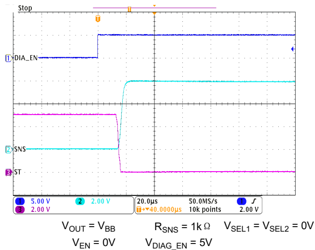
图 6-33. DIAG_EN 上升沿时的开路负载检测时间 ( t_{OL2} )
