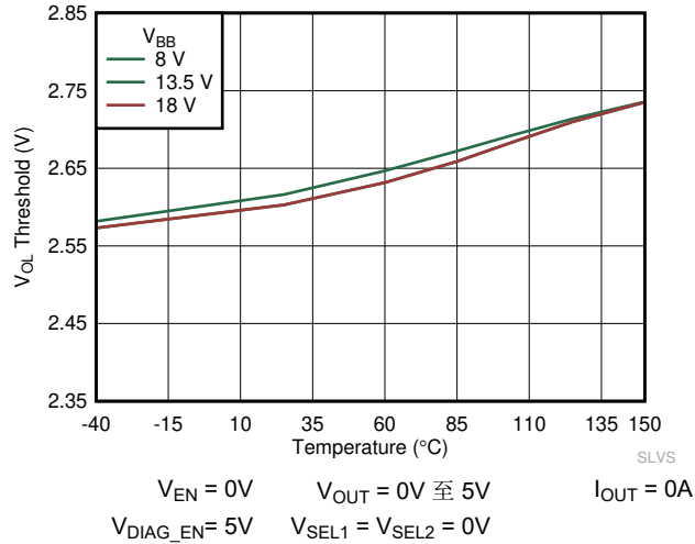
图 6-23. 开路负载检测电压 ( V_{OL} ) 与温度间的关系
