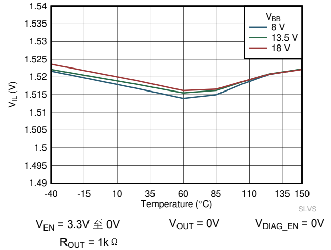
图 6-24. V_{IL} 与温度间的关系
