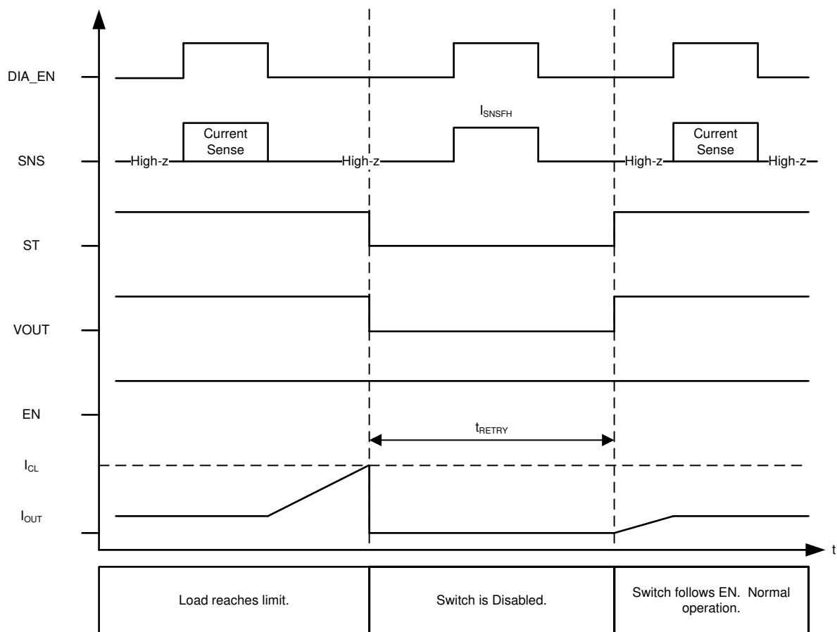
图 8-6. 电流限制 - 版本 A、B、E - LATCH = 0
