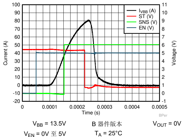
图 6-34. B 器件版本的短路行为
