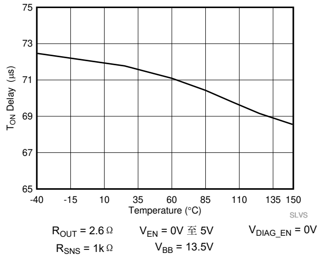
图 6-9. 导通延迟时间 ( t_{DR} ) 与温度间的关系
