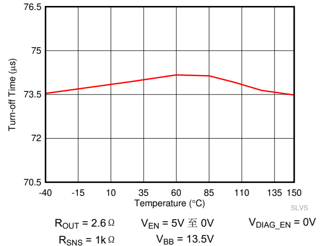
图 6-14. 关断时间 ( t_{OFF} ) 与温度间的关系
