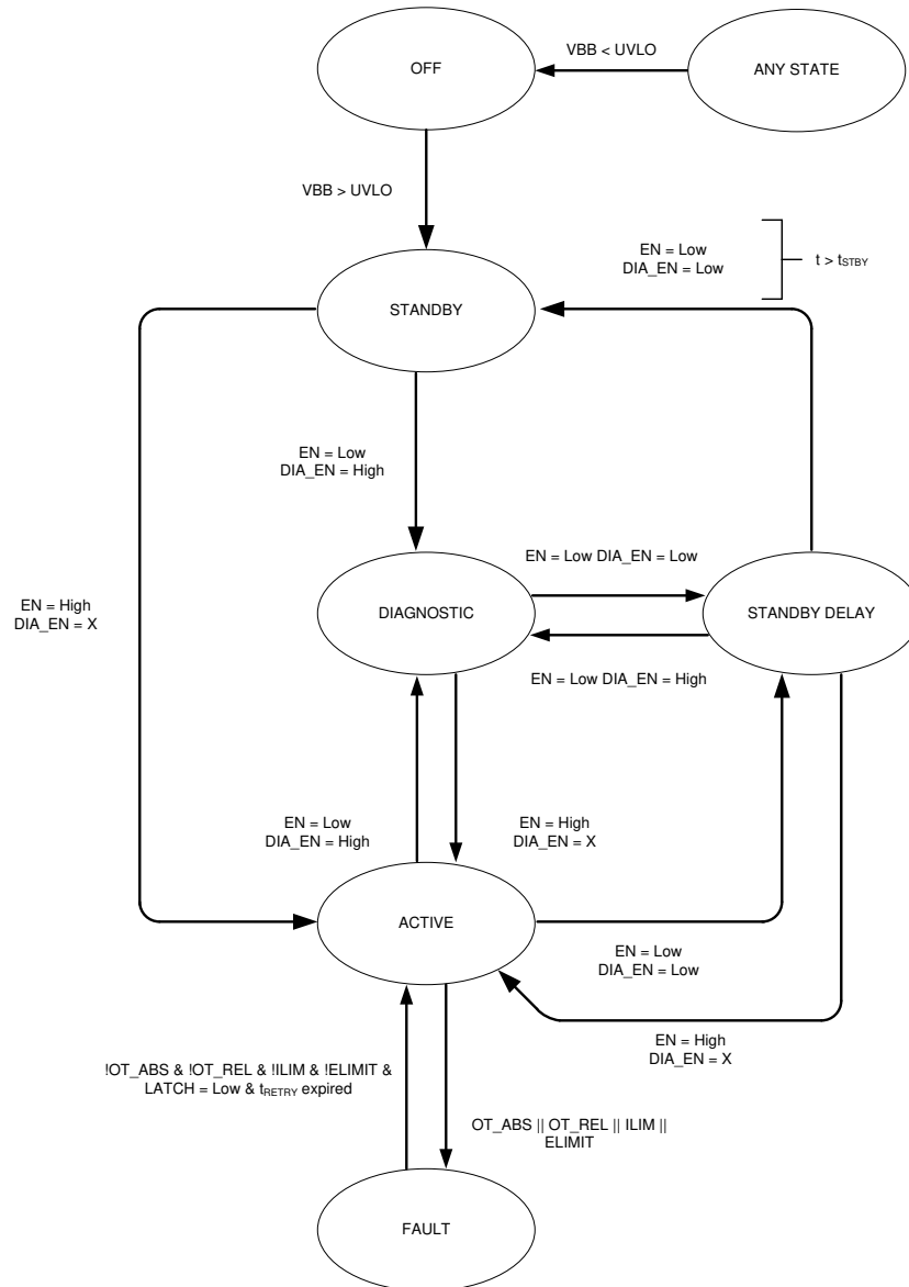
图 8-16. 状态图
