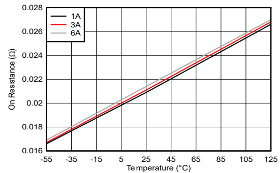
图 6-4. VIN = 1.5V 时 HTSSOP 封装不同负载下导通电阻与温度间的关系
