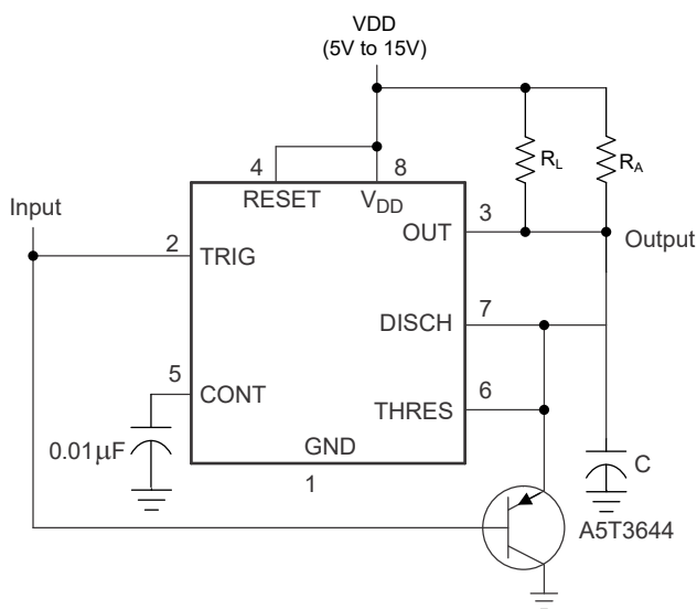
图 7-1. 漏脉冲检测器电路
