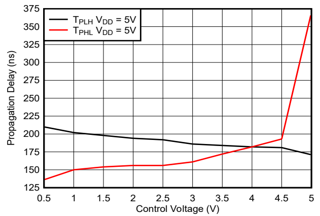
图 5-8. 传播延迟与控制电压间的关系
