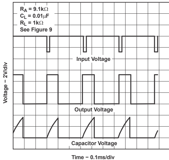
图 6-3. 典型单稳态波形
