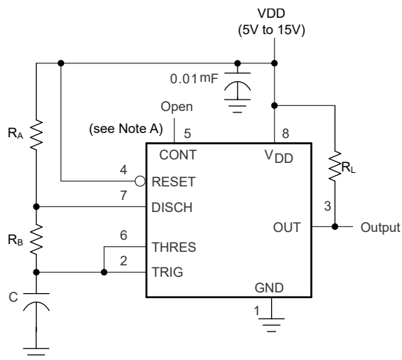
图 6-5. 非稳态工作模式电路
