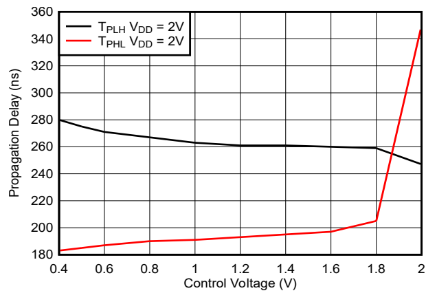
图 5-7. 传播延迟与控制电压间的关系
