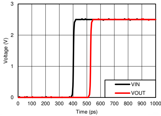
图 8-2. V_{CC} = 2.5V 时的传播延迟 ( t_{pd} ) 仿真结果。
