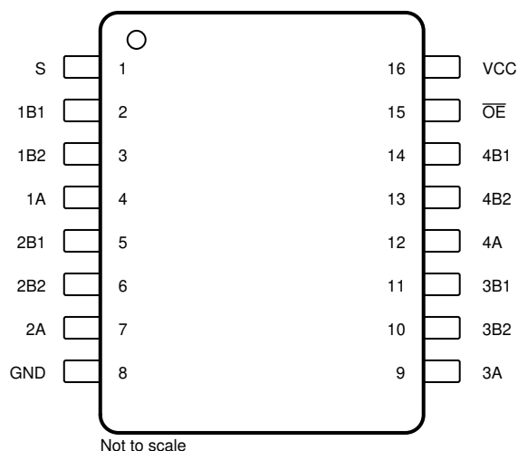
图 4-1. DYY、DGV、DBQ 或 PW 封装 16 引脚 SOT-23 THN、TVSOP、SSOP 或 TSSOP (顶视图)
