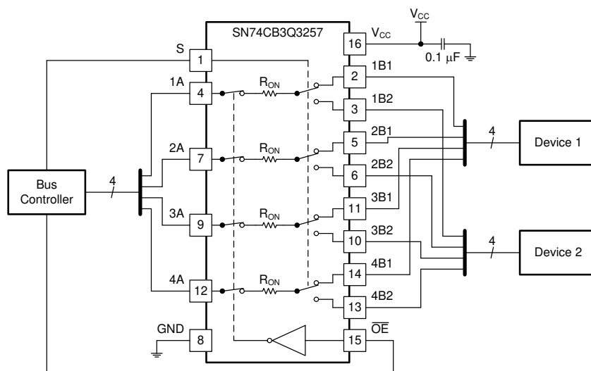
图 8-1. SN74CB3Q3257 典型应用
