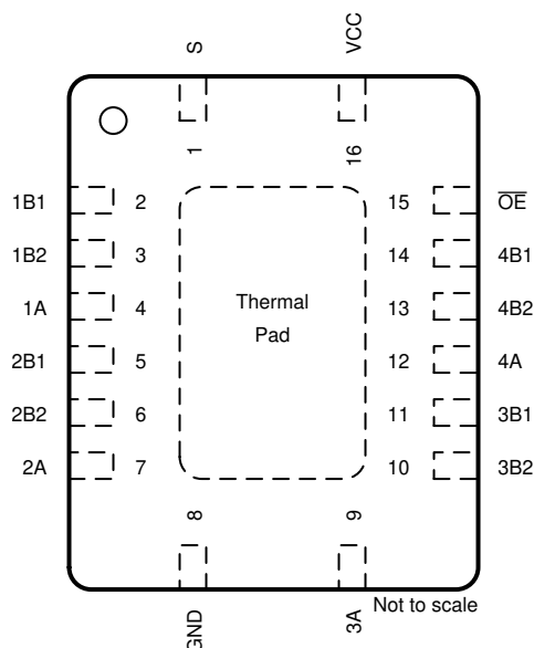
图 4-2. RGY 封装, 16 引脚 VQFN (顶视图)
