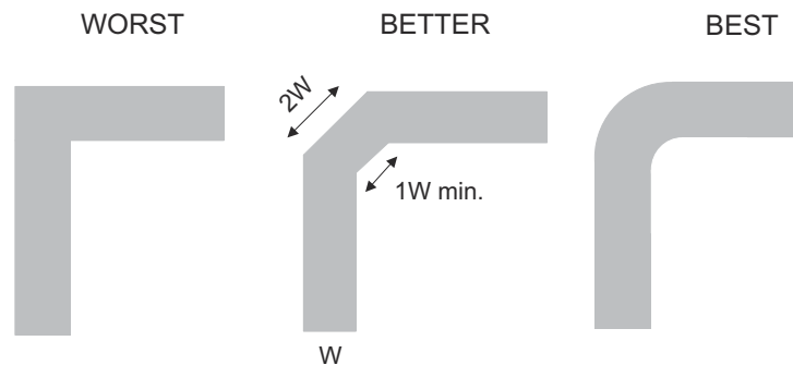
图 8-3. 布线示例
