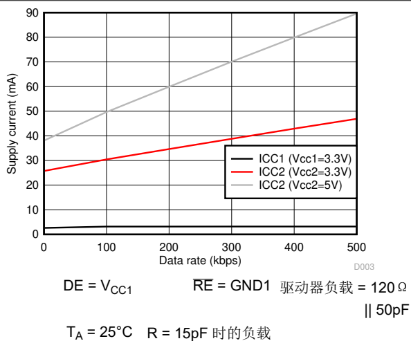
图 6-5. ISO141x 电源电流与数据速率间的关系 - 具有 120\Omega||50\text{pF} 负载
