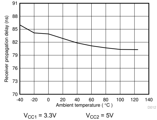
图 6-24. ISO141x 接收器传播延迟 (ns) 与温度 (c) 间的关系
