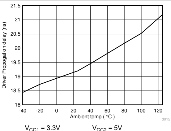
图 6-21. ISO145x 驱动器传播延迟 (ns) 与温度 (C) 间的关系
