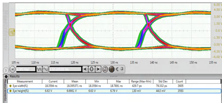
图 9-5. 眼图：50Mbps 时钟、 V_{CC2} = 5\text{V} 、 25^\circ\text{C}
