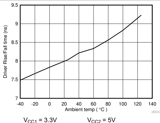
图 6-17. ISO143x 驱动器上升/下降时间 (ns) 与温度 (C) 间的关系
