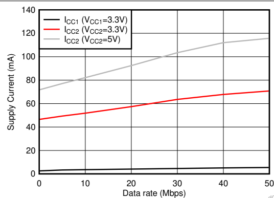
图 6-8. ISO143x 电源电流与数据速率间的关系 - 54\ \Omega || 50\text{pF} 负载
