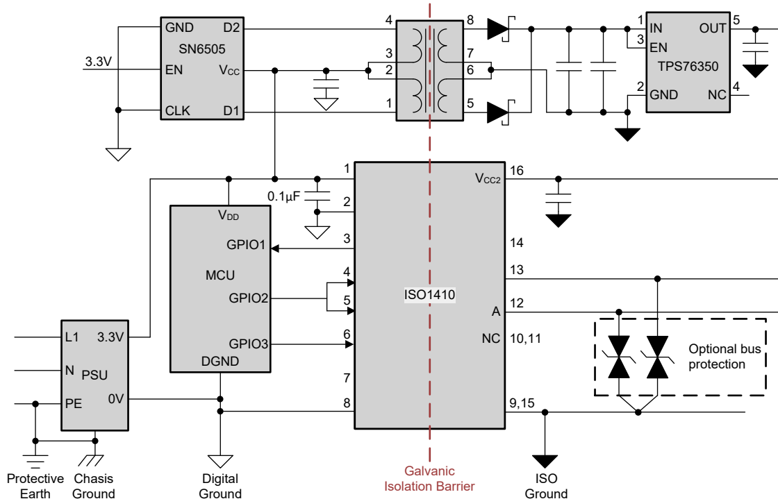
图 9-3. ISO1410 的应用电路
