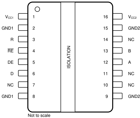
图 5-2. DW 封装 16 引脚 SOIC 半双工器件顶视图
