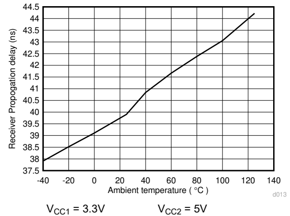
图 6-26. ISO145x 接收器传播延迟 (ns) 与温度 (C) 间的关系
