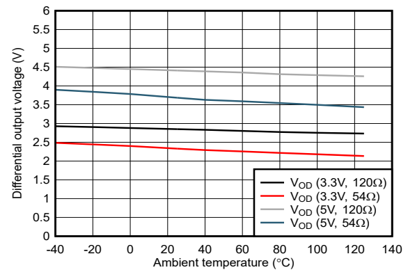
图 6-14. 驱动器差分输出电压与温度间的关系
