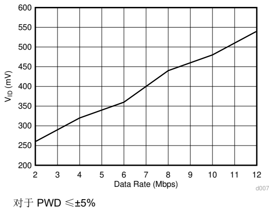
图 6-27. ISO143x 接收器 V_{ID} 与信令速率间的关系
