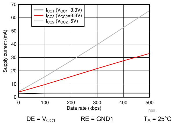
图 6-3. ISO141x 电源电流与数据速率间的关系 - 无负载
