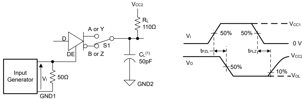
图 7-7. 驱动器启用和禁用时间
