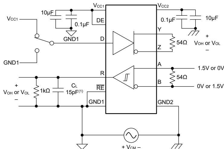
图 7-4. 共模瞬态抗扰度 (CMTI)—全双工
