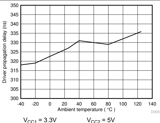
图 6-19. ISO141x 驱动器传播延迟 (ns) 与温度 (c) 间的关系
