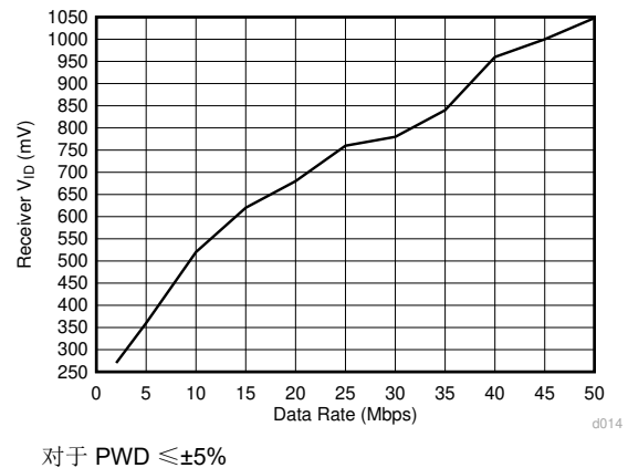
图 6-28. ISO145x 接收器 V_{ID} 与信令速率间的关系
