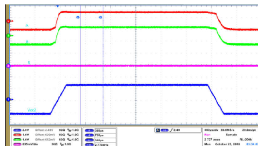
图 6-34. V_{CC2} 加电/断电 - 无毛刺脉冲行为
