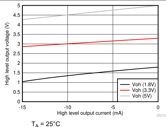
图 6-22. 接收器缓冲器高电平输出电压与高电平输出电流间的关系
