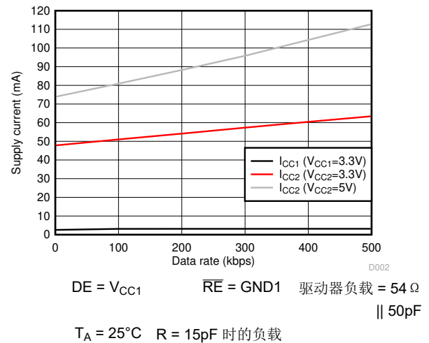
图 6-4. ISO141x 电源电流与数据速率间的关系 - 具有 54\Omega||50\text{pF} 负载
