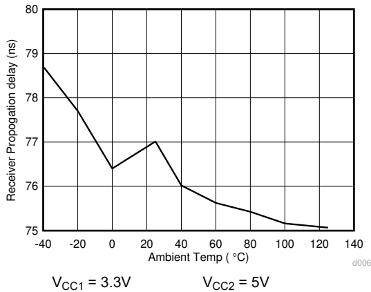
图 6-25. ISO143x 接收器传播延迟 (ns) 与温度 (C) 间的关系
