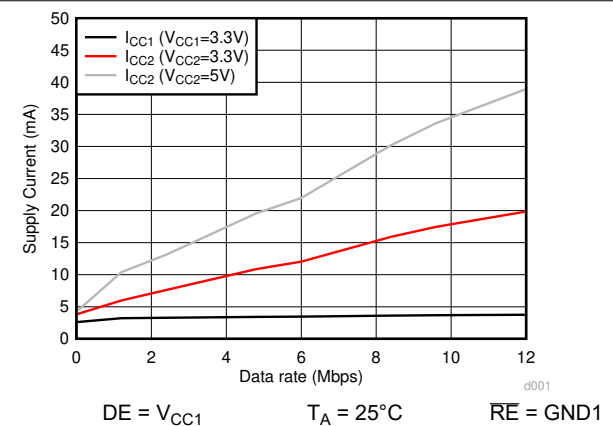
图 6-6. ISO143x 电源电流与数据速率间的关系 - 无负载
