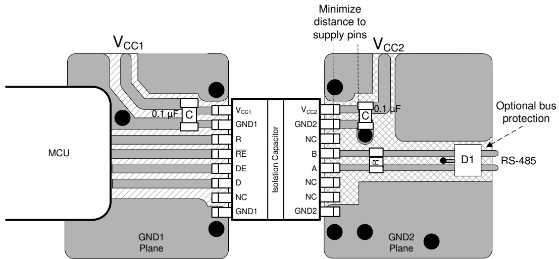
图 9-9. 布局示例
