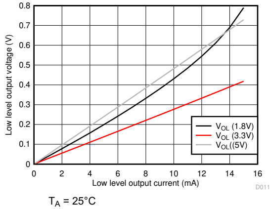
图 6-23. 接收器缓冲器低电平输出电压与低电平输出电流间的关系
