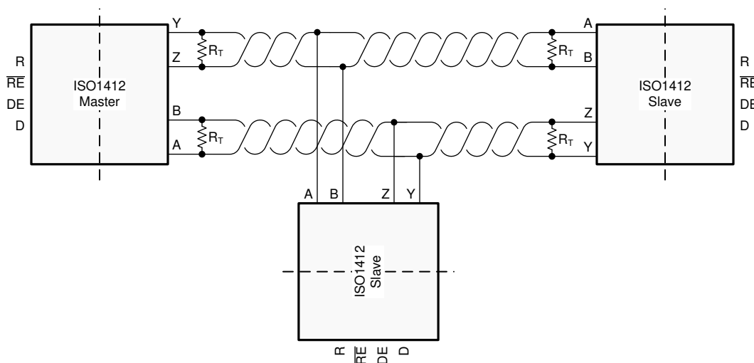
图 9-1. 具有全双工隔离式收发器的典型 RS-485 网络
