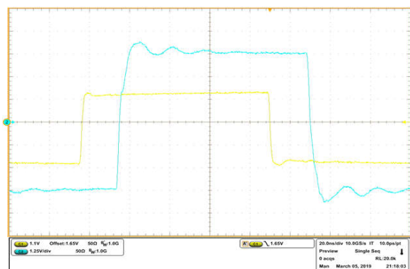
图 6-29. ISO141x 驱动器传播延迟
