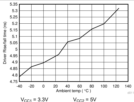
图 6-18. ISO145x 驱动器上升/下降时间 (ns) 与温度 (C) 间的关系
