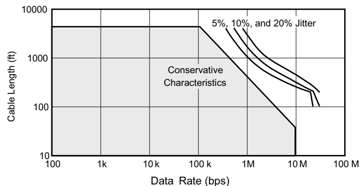
图 9-4. 电缆长度与数据速率特性间的关系
