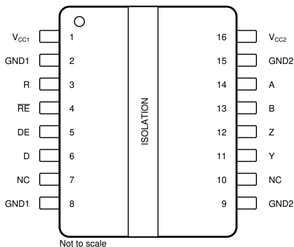
图 5-1. DW 封装 16 引脚 SOIC 全双工器件顶视图
