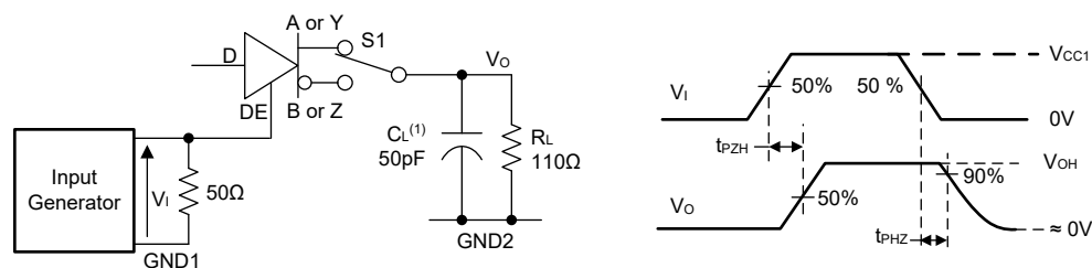
图 7-5. 共模瞬态抗扰度 (CMTI)—半双工
