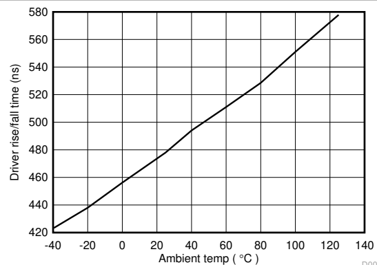
图 6-16. ISO141x 驱动器上升/下降时间 (ns) 与温度 (c) 间的关系
