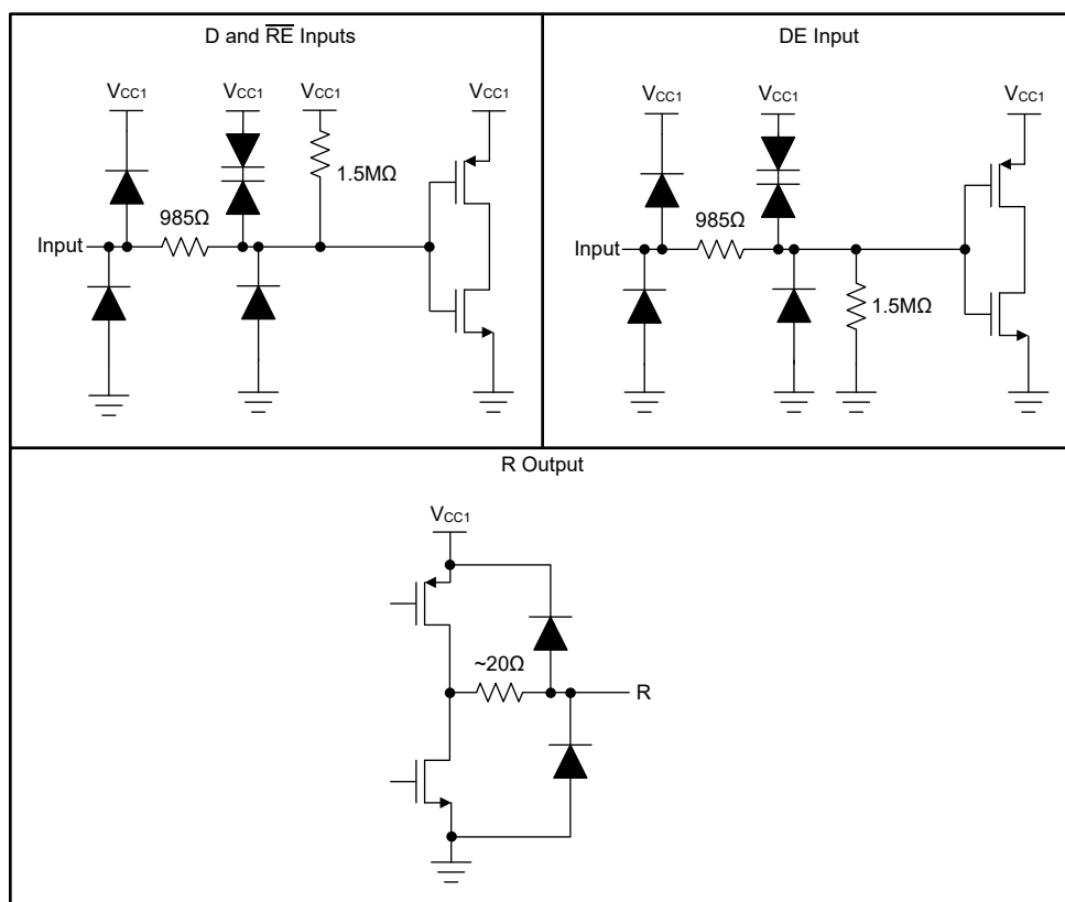
图 8-4. 器件 I/O 原理图
