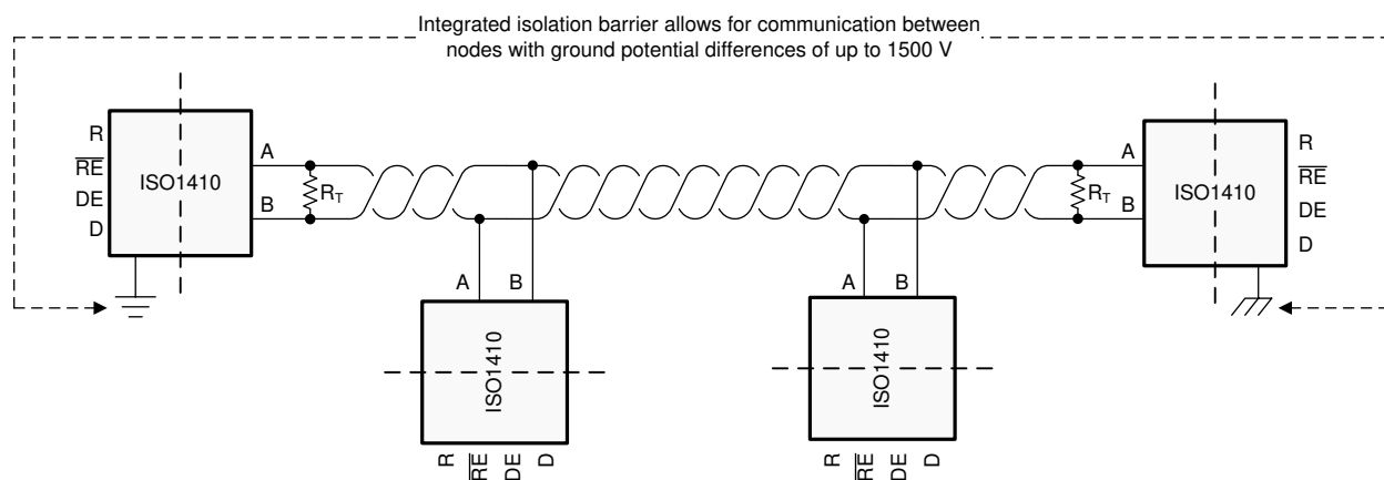
图 9-2. 具有半双工隔离式收发器的典型 RS-485 网络
