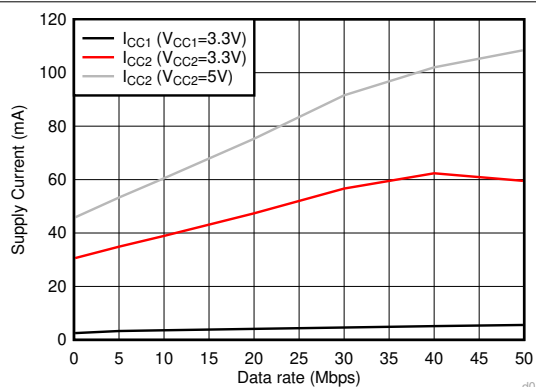
图 6-7. ISO143x 电源电流与数据速率间的关系 - 120\ \Omega || 50\text{pF} 负载
