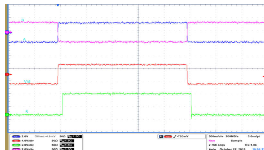
图 6-30. ISO143x 驱动器传播延迟
