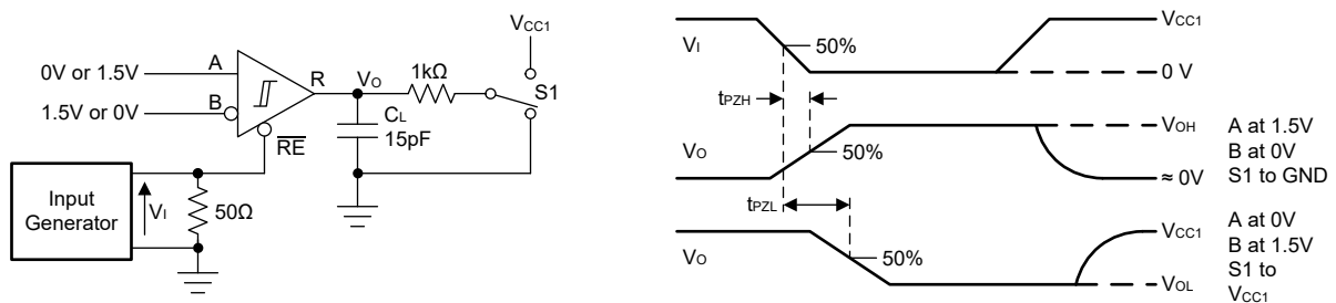
图 7-10. 接收器启用和禁用时间
