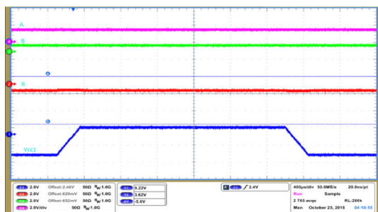
图 6-33. V_{CC1} 加电/断电 - 无毛刺脉冲行为
