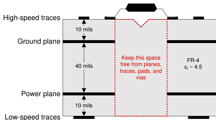
图 9-8. 建议的层堆叠
