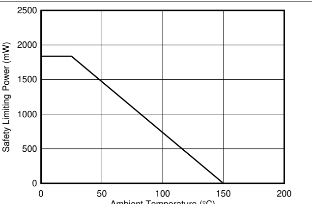
图 6-2. 根据 VDE 标准限制功率的热降额曲线
