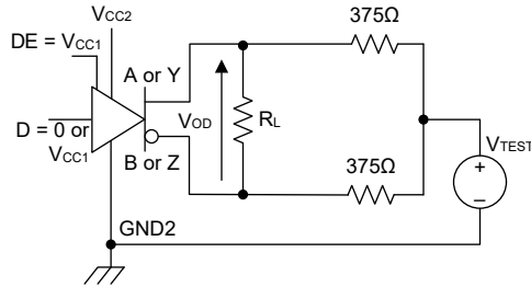
图 7-1. 驱动器电压
