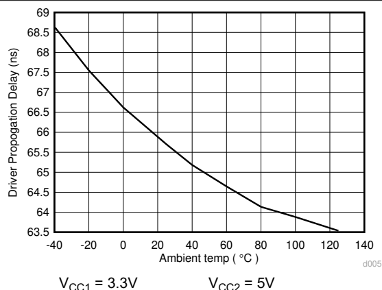
图 6-20. ISO143x 驱动器传播延迟 (ns) 与温度 (C) 间的关系
