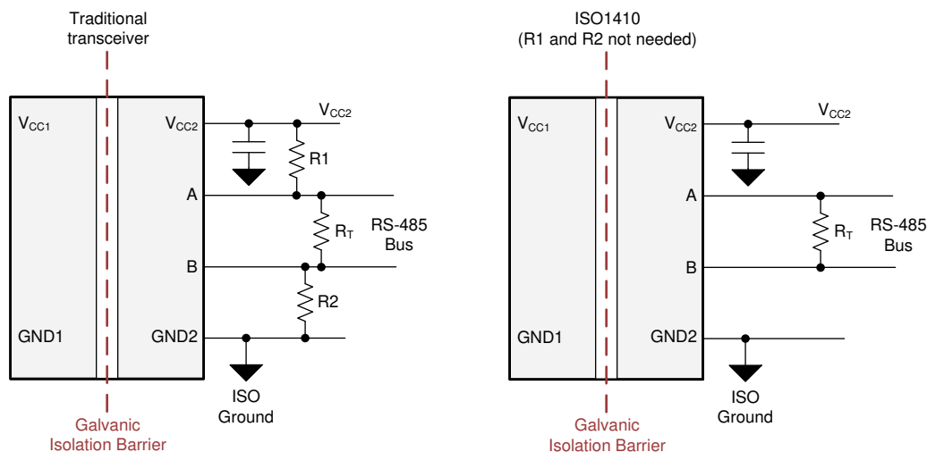
图 8-3. 失效防护收发器
