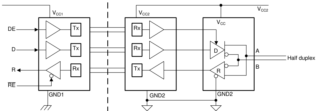
图 8-2. 半双工方框图
