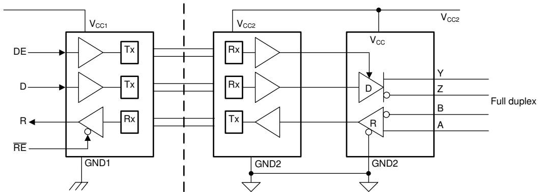
图 8-1. 全双工方框图
