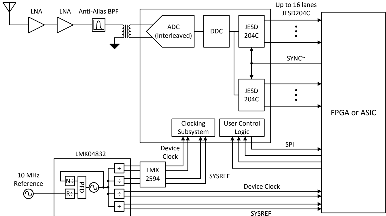
图 8-1. 宽带射频采样的典型配置
