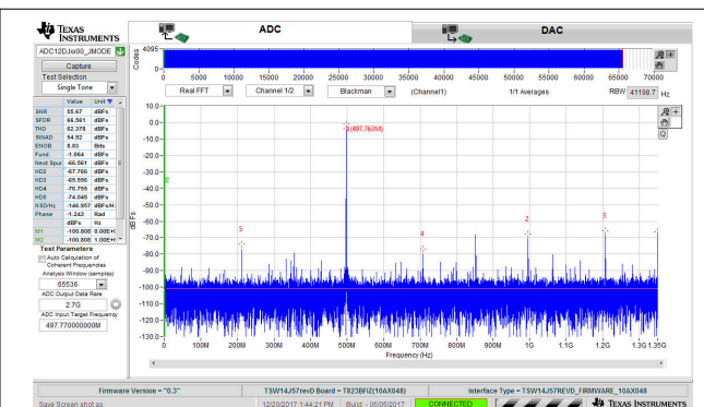
图 8-3. 针对 497.77MHz 输入信号的 FFT，2.7GSPS，JMODE2
