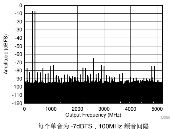
图 6-11. DES 模式：347MHz 时的双音 FFT
