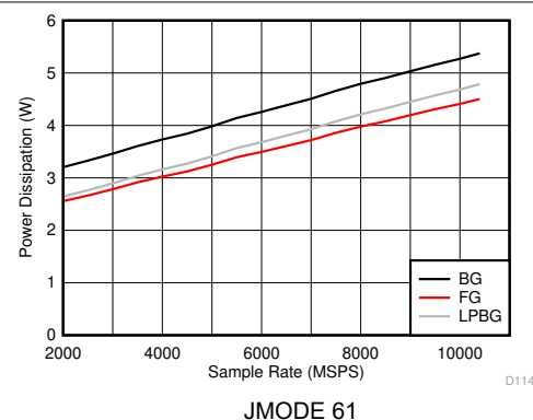
图 6-144. DES 模式：功耗与采样率间的关系
