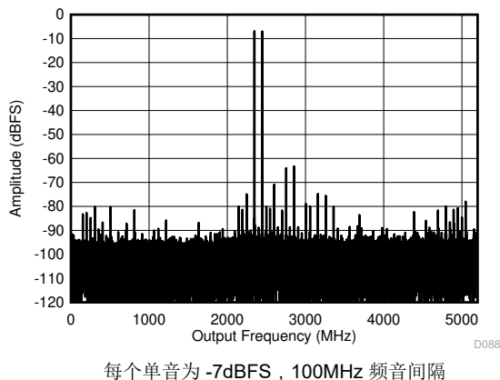
图 6-13. DES 模式：2397MHz 时的双音 FFT
