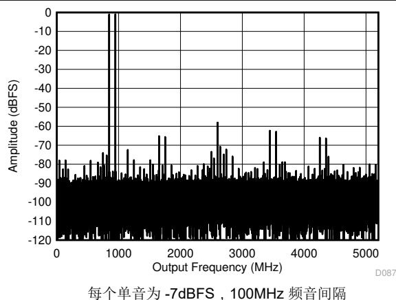
图 6-12. DES 模式：897MHz 时的双音 FFT
