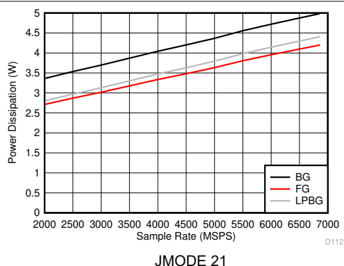
图 6-142. DES 模式：功耗与采样率间的关系
