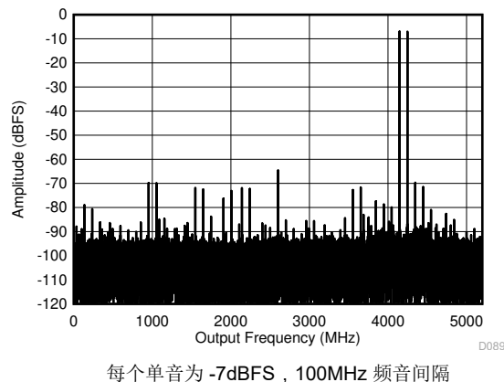
图 6-14. DES 模式：4197MHz 时的双音 FFT
