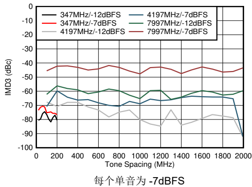
图 6-101. DES 模式：IMD3 与频音间隔间的关系
