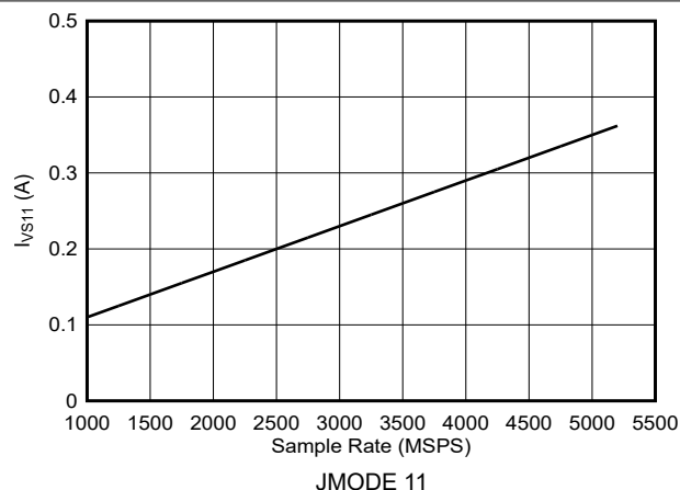
图 6-152. 双通道模式： I_{VD11} 与采样率间的关系 (ADC12DJ5210RF)
