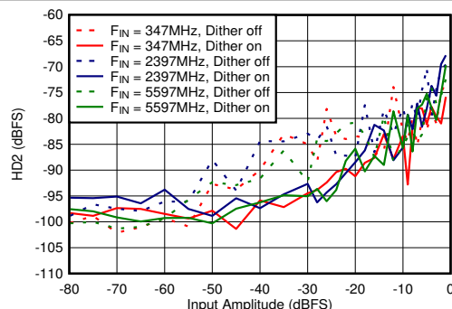
图 6-62. DES 模式：HD2 与输入振幅和抖动间的关系
