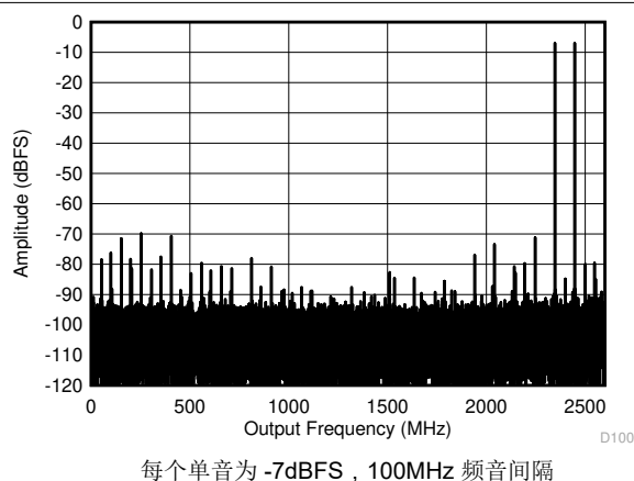
图 6-25. 双通道模式：2397MHz 时的双音 FFT
