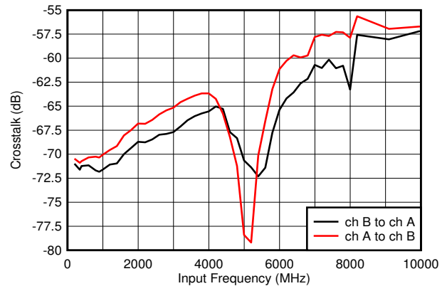
图 6-2. 串扰与输入频率间的关系
