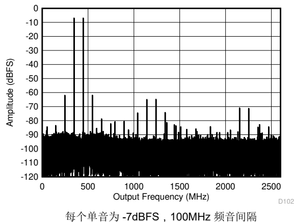
图 6-27. 双通道模式：5597MHz 时的双音 FFT
