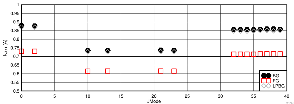
图 6-121. 具有较低最大 F_S 的其他模式： I_{VA19} 与 \text{JMODE} 间的关系
