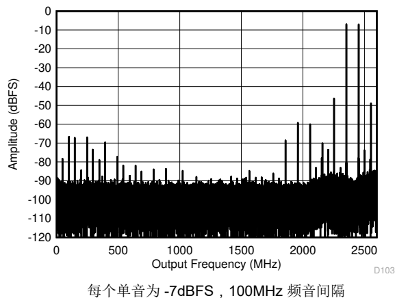
图 6-28. 双通道模式：7997MHz 时的双音 FFT
