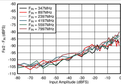
图 6-79. 双通道模式：Fs/2 - F_IN 与输入振幅和频率间的关系
