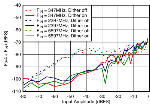
图 6-66. DES 模式: F_s/2 + F_{\text{IN}} 与输入振幅和抖动间的关系
