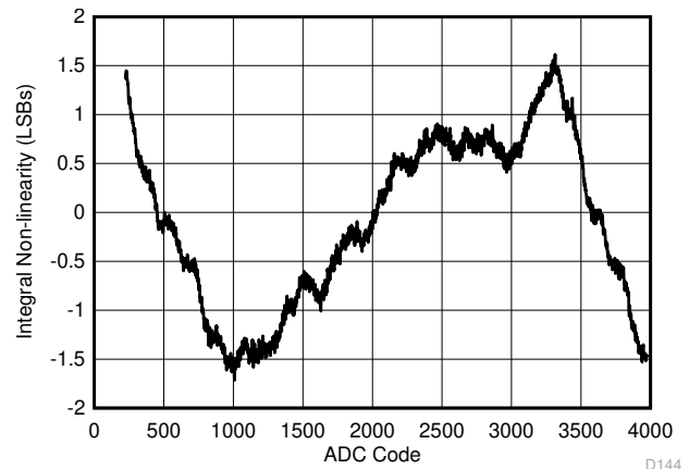
图 6-4. INL 与 ADC 代码间的关系
