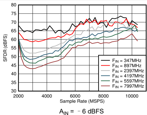
图 6-33. DES 模式：SFDR 与采样率和输入频率间的关系
