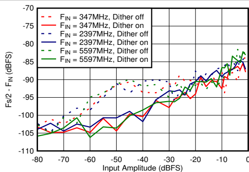
图 6-80. 双通道模式：Fs/2 - F_IN 与输入振幅和抖动间的关系
