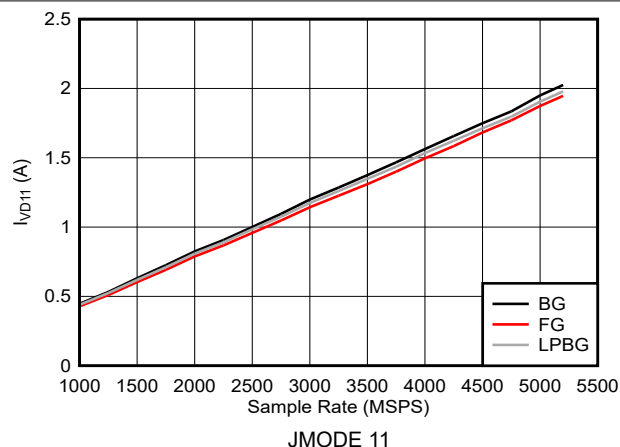
图 6-151. 双通道模式： I_{VD11} 与采样率间的关系 (ADC12DJ5210RF)
