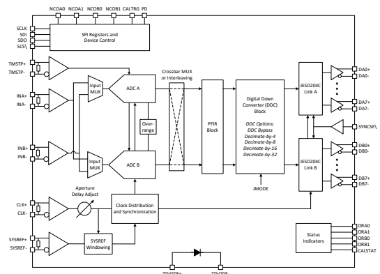
ADC12DJ52x0RF 方框图
