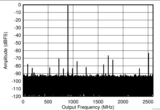
图 6-18. 双通道模式：897MHz 时的单音 FFT
