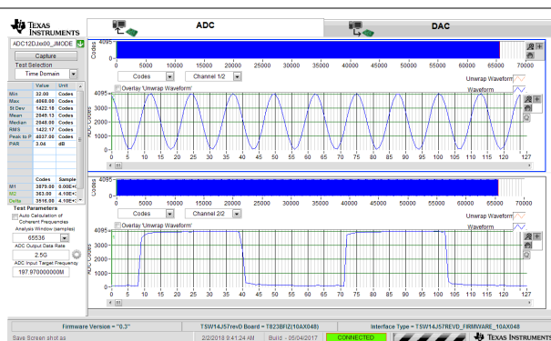
图 8-11. 5GSPS 单通道示波器的 200MHz 正弦波 (通道 A) 和 40MHz 方波 (通道 B) 时域
