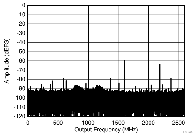
图 6-20. 双通道模式：4197MHz 时的单音 FFT
