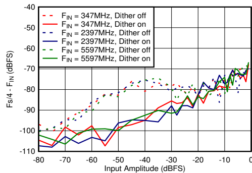
图 6-70. DES 模式: F_s/4 - F_{\text{IN}} 与输入振幅和抖动间的关系
