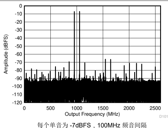
图 6-26. 双通道模式：4197MHz 时的双音 FFT
