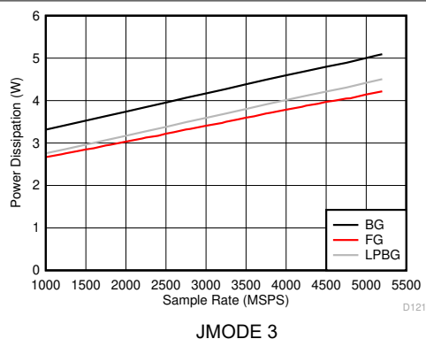
图 6-159. 双通道模式：功耗与采样率间的关系
