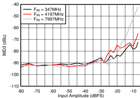
图 6-105. 双通道模式：IMD3 与输入幅度间的关系
