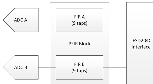
图 7-4. 双通道均衡 PFIR 方框图
