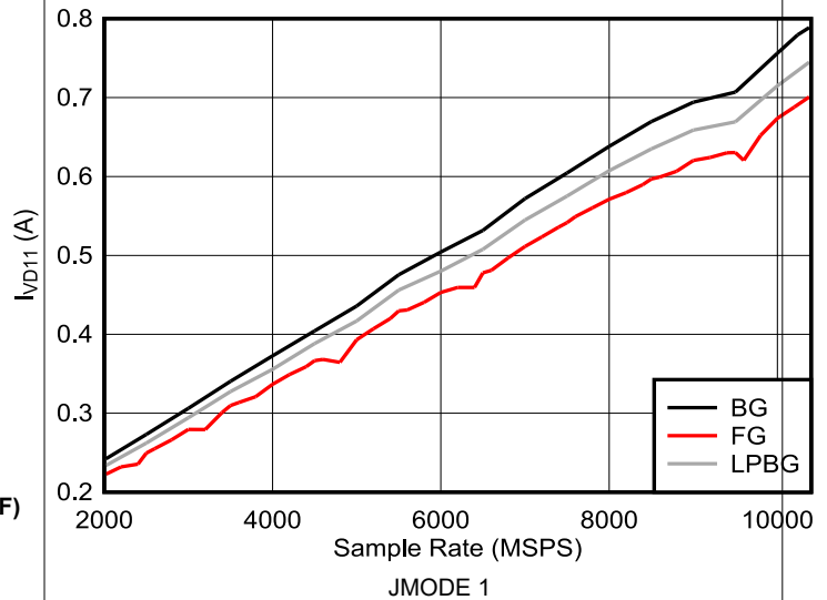
图 6-130. DES 模式: I_{VD11} 与采样率间的关系 (ADC12DJ5210RF)
