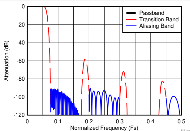
图 7-13. 8 倍抽取复合响应
