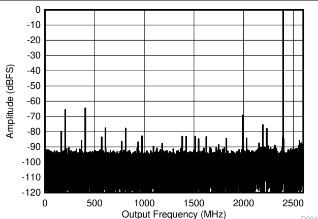
图 6-19. 双通道模式：2397MHz 时的单音 FFT
