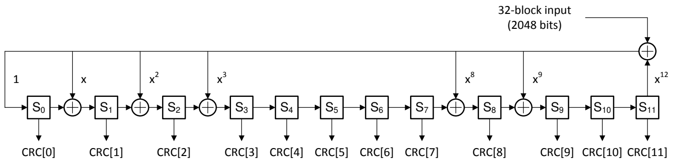
图 7-21. CRC-12 奇偶校验位发生器
