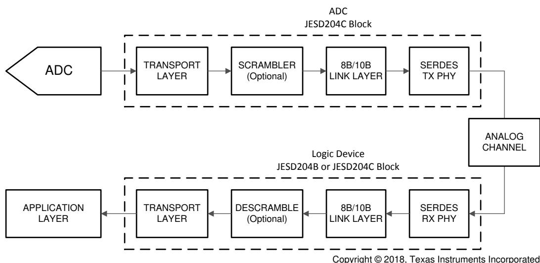
图 7-19. 8B/10B 编码的 JESD204C 简化接口图
