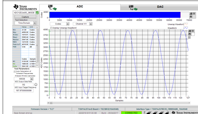
图 8-8. 5GSPS 单通道示波器的 200MHz 正弦波时域
