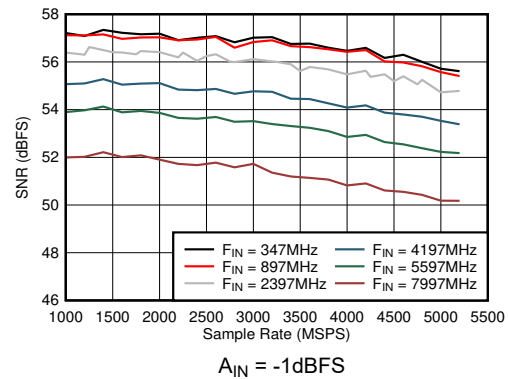
图 6-44. 双通道模式：SNR 与采样率和输入频率间的关系
