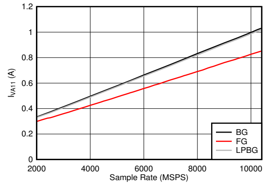
图 6-128. DES 模式: I_{VA11} 与采样率间的关系
