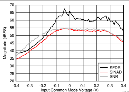
图 6-97. SNR、SFDR 和 SINAD 与输入共模电压间的关系
