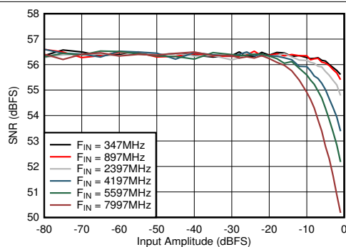
图 6-71. 双通道模式：SNR 与输入振幅和频率间的关系
