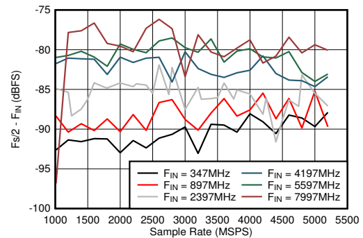
图 6-56. 双通道模式：Fs/2 - F_{\text{IN}} 与采样率和输入频率间的关系
