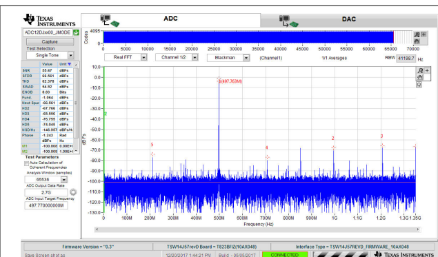
图 8-3. 针对 497.77MHz 输入信号的 FFT，2.7GSPS，JMODE2
