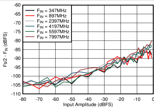
图 6-79. 双通道模式：Fs/2 - f_{\text{IN}} 与输入振幅和频率间的关系
