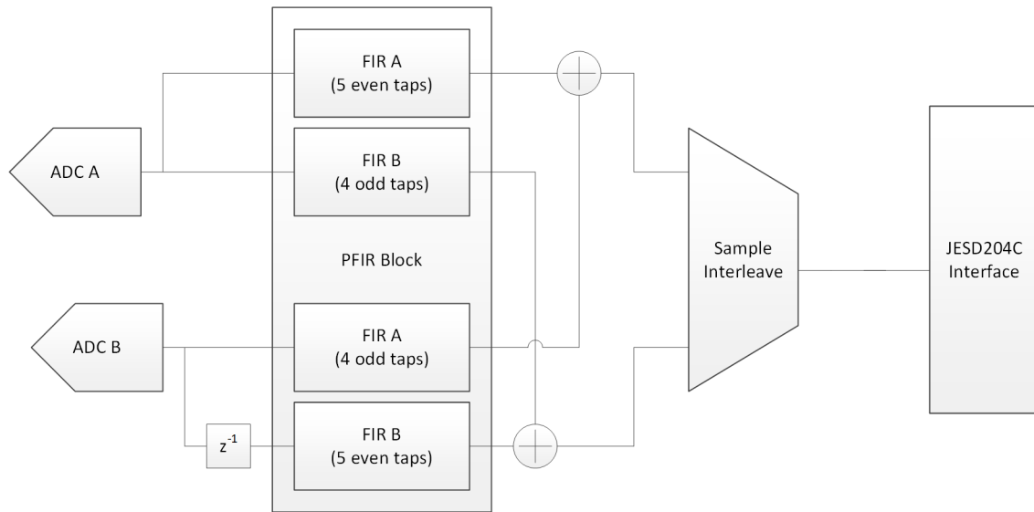
图 7-7. 备选 I/Q 校正型滤波器方框图
