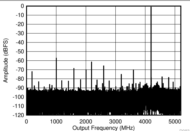
图 6-8. DES 模式：4197MHz 时的单音 FFT
