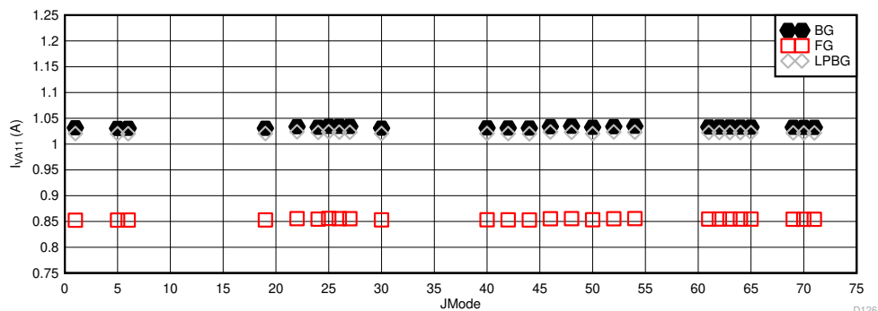
图 6-109. DES 模式：在 10.4GSPS 时的 I_{VA19} 与 JMODE
