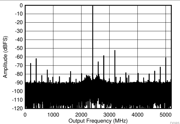
图 6-10. DES 模式：7997MHz 时的单音 FFT
