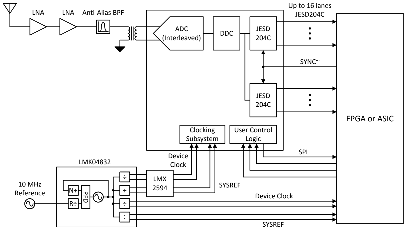
图 8-1. 宽带射频采样的典型配置
