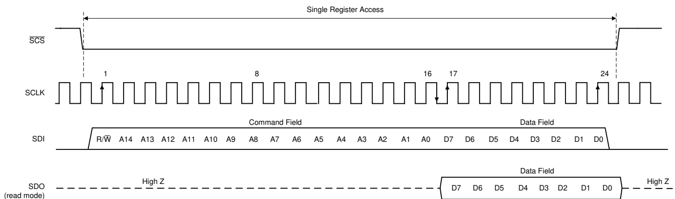
图 7-27. 串行接口协议：单读取/写入
