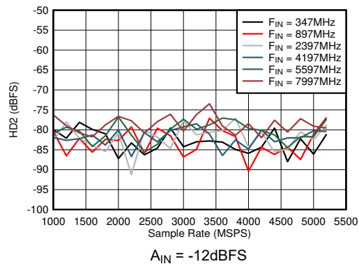
图 6-52. 双通道模式：HD2 与采样率和输入频率间的关系
