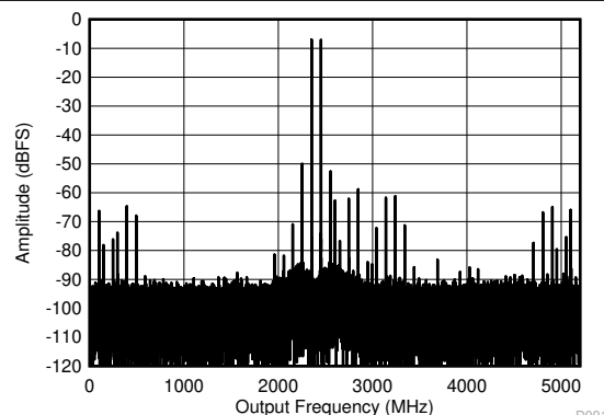
图 6-16. DES 模式：7997MHz 时的双音 FFT
