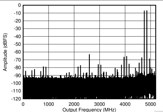
图 6-15. DES 模式：5597MHz 时的双音 FFT
