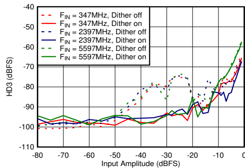
图 6-64. DES 模式：HD3 与输入振幅和抖动间的关系
