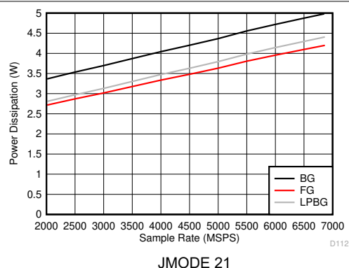
图 6-142. DES 模式：功耗与采样率间的关系
