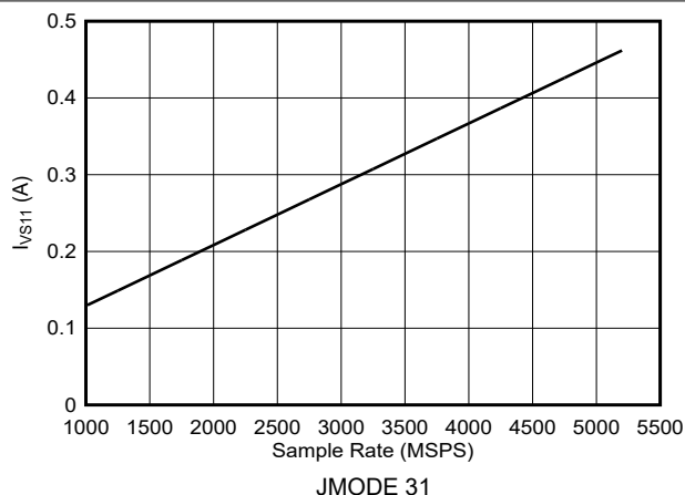
图 6-155. 双通道模式: I_{VS11} 与采样率间的关系 (ADC12DJ5210RF)
