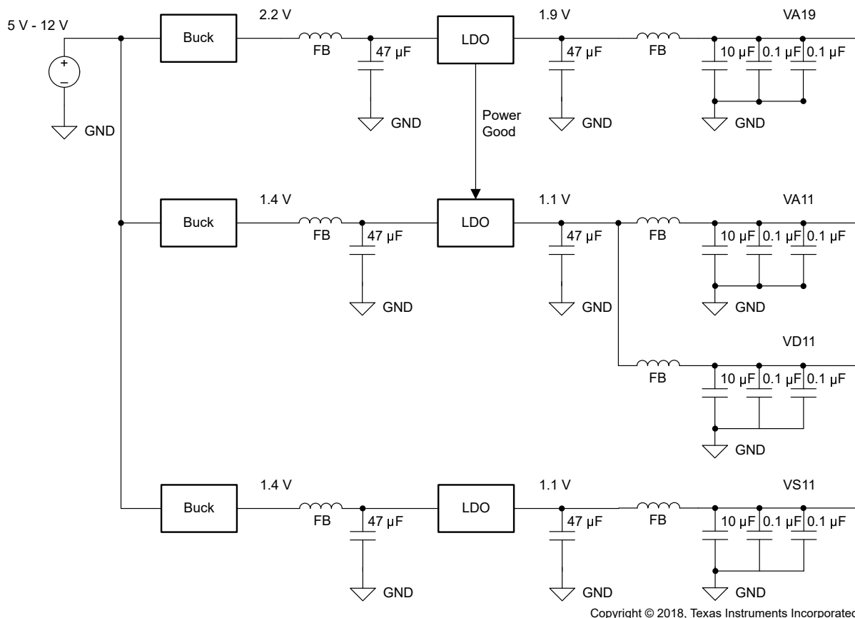
图 8-15. LDO 线性稳压器方法示例 (ADC12DJ5210RF)
