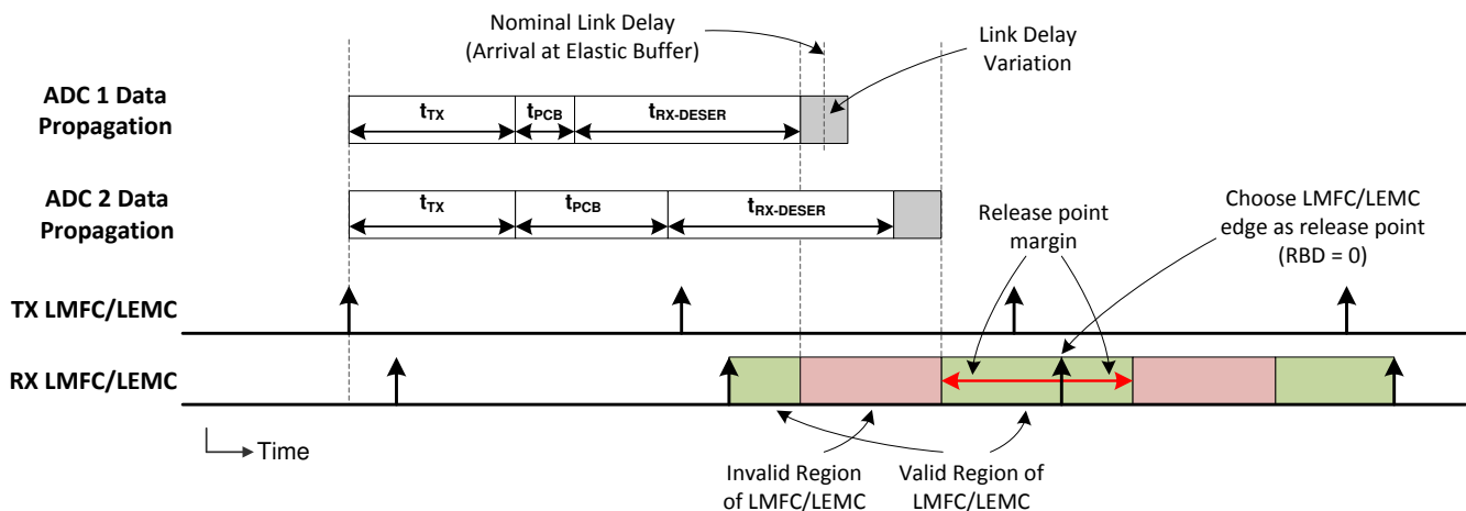
图 7-23. 用于弹性缓冲器释放点选择的 LMFC/LEMC 有效区域定义
