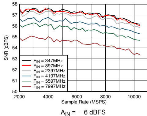
图 6-30. DES 模式：SNR 与采样率和输入频率间的关系
