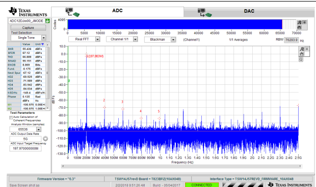
图 8-9. 5GSPS 单通道示波器的 200MHz 正弦波频域 (FFT)
