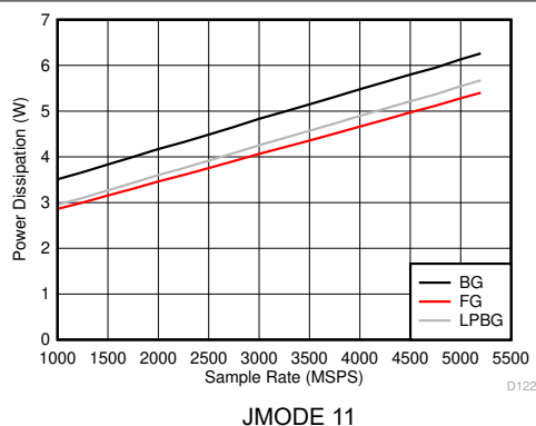
图 6-160. 双通道模式：功耗与采样率间的关系
