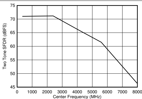
图 6-107. 双通道模式：双音 SFDR 与输入频率间的关系
