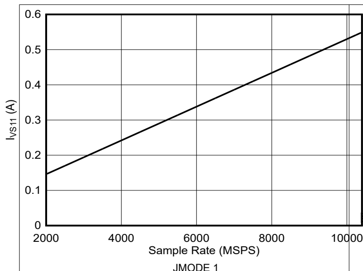
图 6-131. DES 模式： I_{VS11} 与采样率间的关系 (ADC12DJ5210RF)
