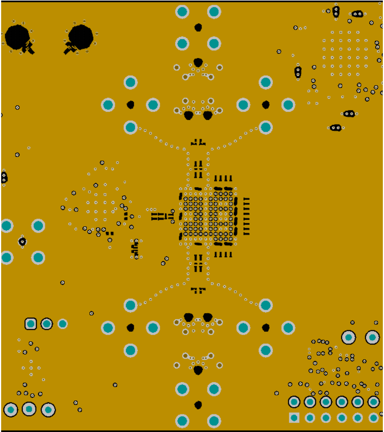
图 8-18. GND1 开孔可优化元件焊盘的阻抗
