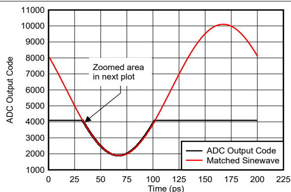
图 6-170. 正弦波过驱恢复
