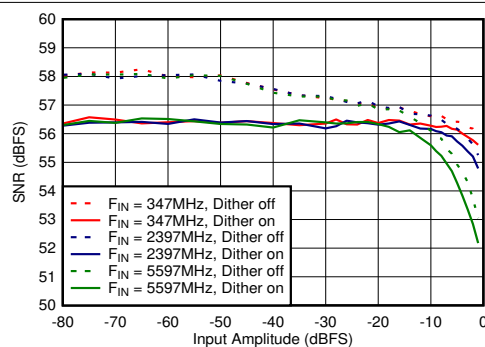
图 6-72. 双通道模式：SNR 与输入振幅和抖动间的关系
