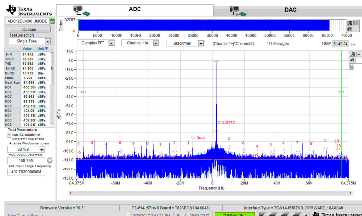
图 8-4. 针对 497.77MHz 输入信号的 FFT，2.7GSPS，16 倍抽取， f_{NCO} = 500\text{MHz} ，JMODE16
