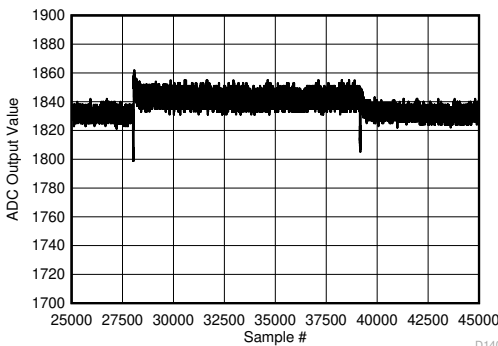
图 6-167. 后台校准内核转换 (放大直流信号)
