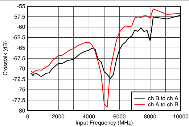
图 6-2. 串扰与输入频率间的关系
