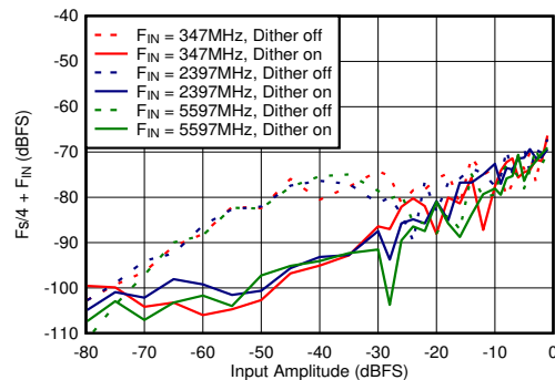
图 6-68. DES 模式： F_s/4 + F_{\text{IN}} 与输入振幅和抖动间的关系
