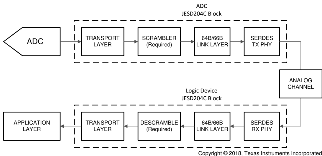
图 7-20. 64B/66B 编码的 JESD204C 简化接口图
