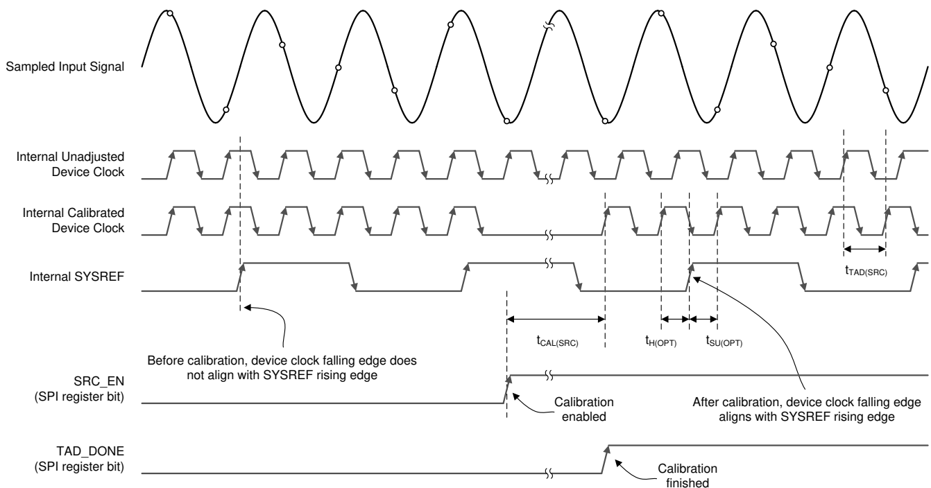
图 7-3. SYSREF 校准时序图
