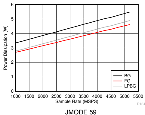
图 6-162. 双通道模式：功耗与采样率间的关系
