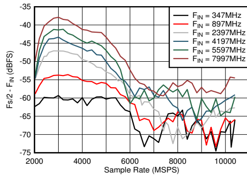
图 6-41. DES 模式：Fs/2 - F_{IN} 与采样率和输入频率间的关系
