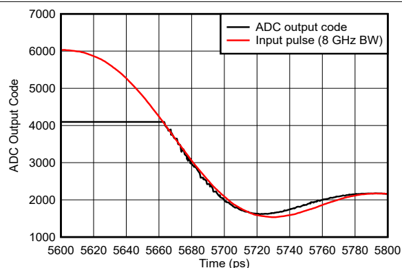
图 6-169. 脉冲过驱恢复 (放大)
