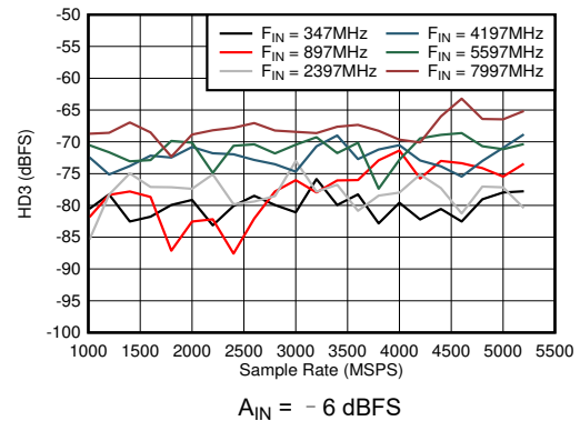
图 6-54. 双通道模式：HD3 与采样率和输入频率间的关系
