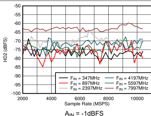
图 6-35. DES 模式：HD2 与采样率和输入频率间的关系
