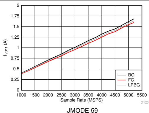
图 6-156. 双通道模式: I_{VD11} 与采样率间的关系 (ADC12DJ5200RF)
