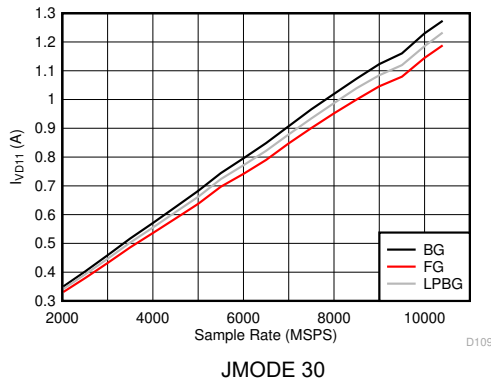
图 6-135. DES 模式： I_{VD11} 与采样率间的关系 (ADC12DJ5200RF)
