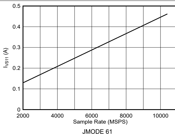
图 6-140. DES 模式： I_{VS11} 与采样率间的关系 (ADC12DJ5210RF)
