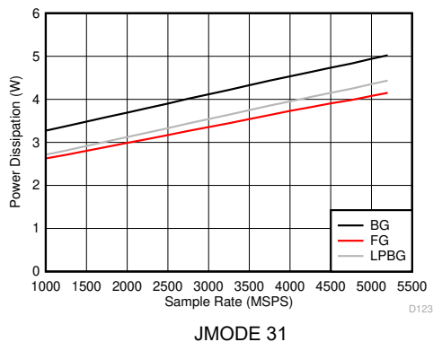
图 6-161. 双通道模式：功耗与采样率间的关系
