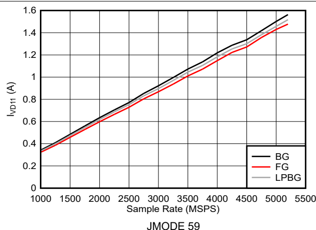
图 6-157. 双通道模式： I_{VD11} 与采样率间的关系 (ADC12DJ5210RF)
