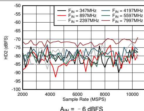
图 6-36. DES 模式：HD2 与采样率和输入频率间的关系
