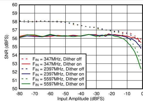
图 6-58. DES 模式：SNR 与输入振幅和抖动间的关系
