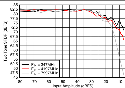
图 6-108. 双通道模式：双音 SFDR 与输入振幅间的关系
