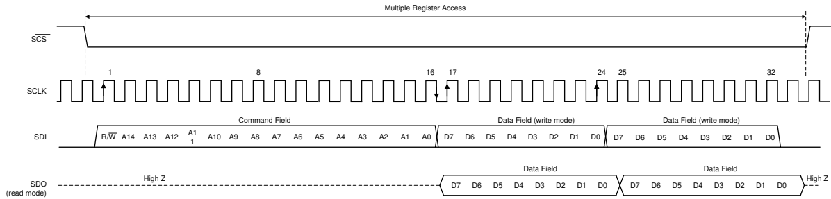
图 7-28. 串行接口协议：流式读取/写入
