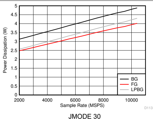
图 6-143. DES 模式：功耗与采样率间的关系
