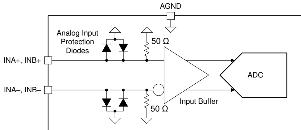
图 7-1. ADC12DJ52x0RF 模拟输入内部端接和保护图
