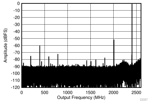
图 6-22. 双通道模式：7997MHz 时的单音 FFT
