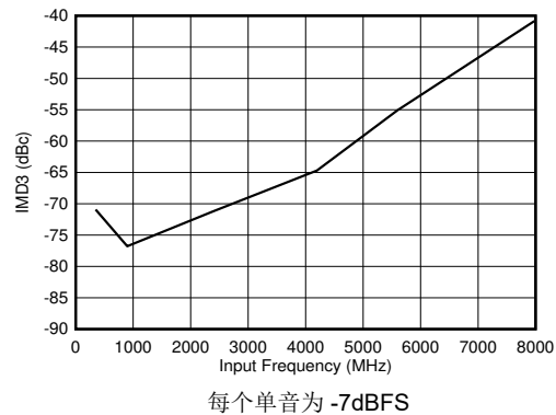
图 6-104. 双通道模式：IMD3 与输入频率间的关系
