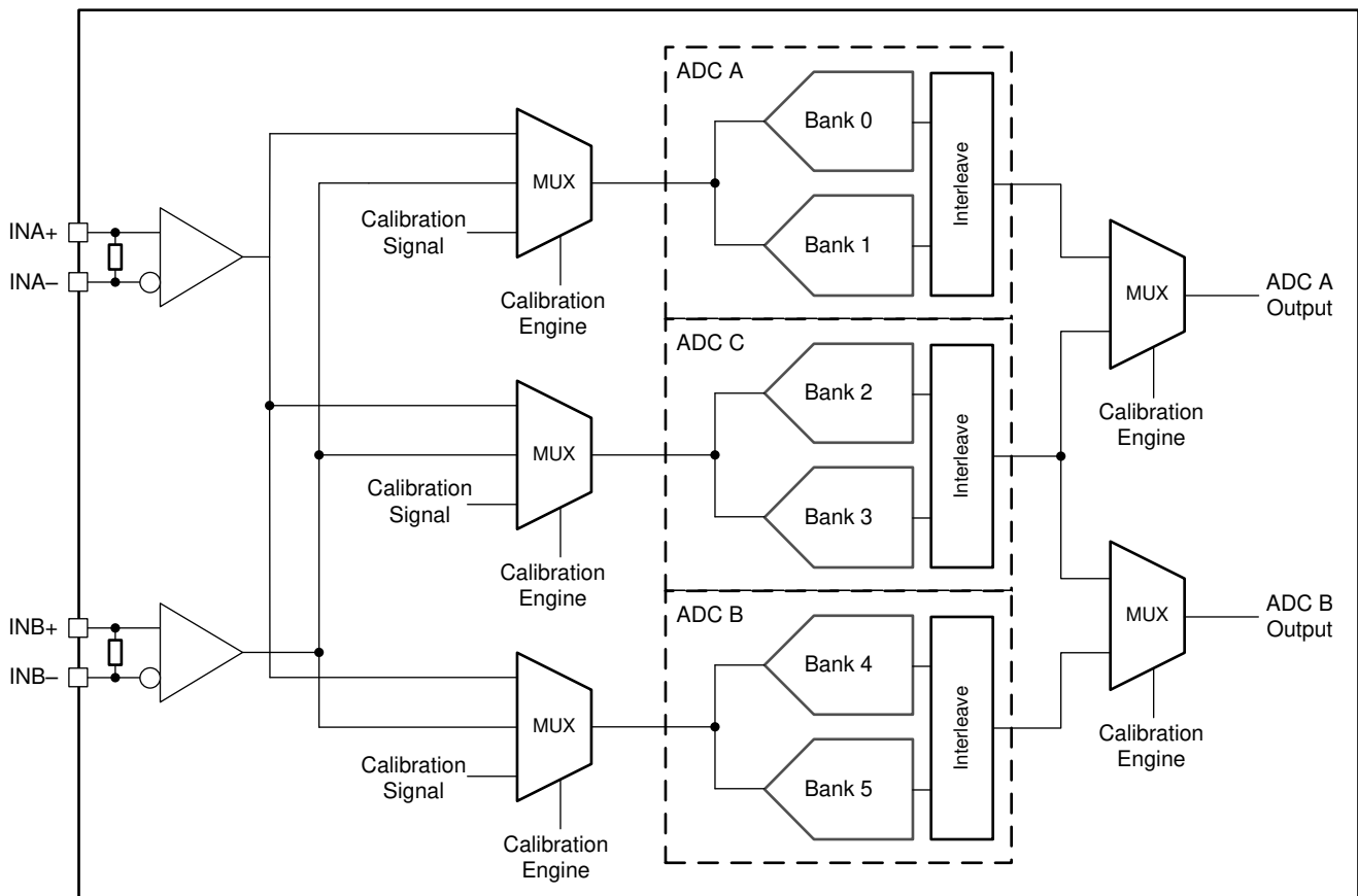
图 7-26. ADC12DJ52x0RF 校准系统方框图
