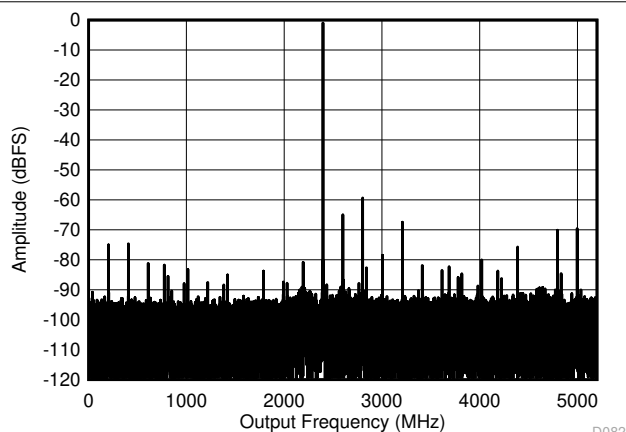
图 6-7. DES 模式：2397MHz 时的单音 FFT
