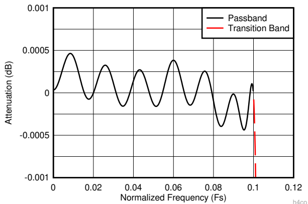
图 7-12. 4 倍抽取复合放大通带响应
