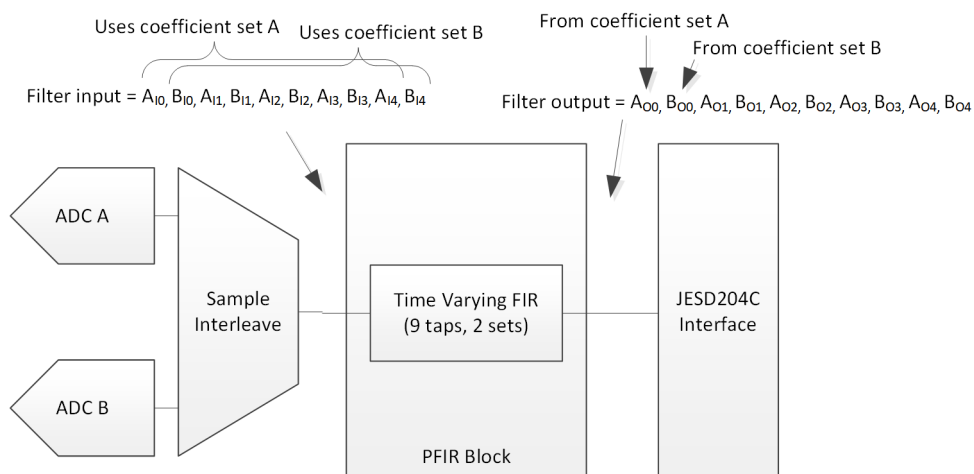
图 7-6. 时变滤波器 PFIR 方框图
