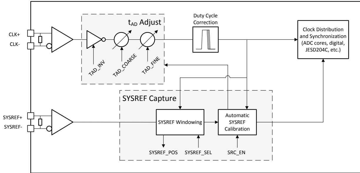
图 7-2. 时钟子系统
