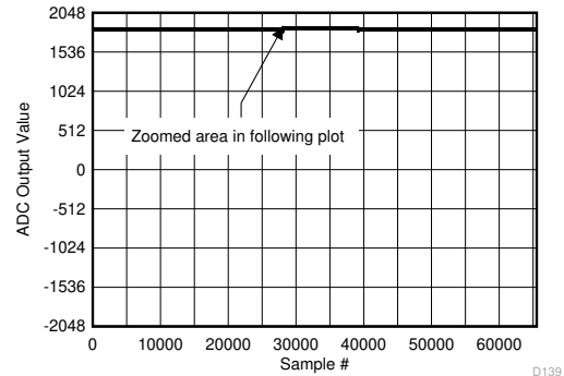
图 6-166. 后台校准内核转换 (直流信号)
