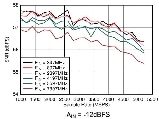
图 6-46. 双通道模式：SNR 与采样率和输入频率间的关系
