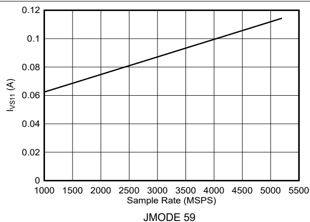
图 6-158. 双通道模式： I_{VS11} 与采样率间的关系 (ADC12DJ5210RF)
