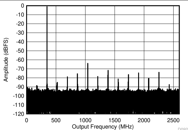
图 6-17. 双通道模式：347MHz 时的单音 FFT
