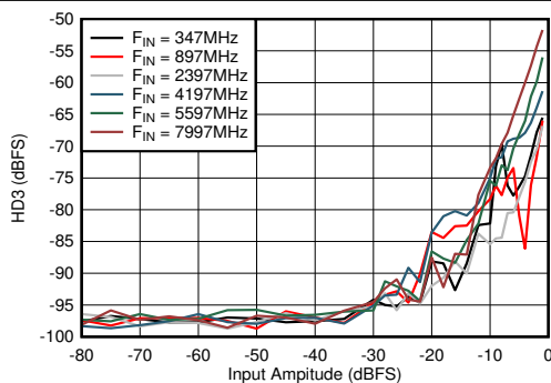
图 6-77. 双通道模式：HD3 与输入振幅和频率间的关系
