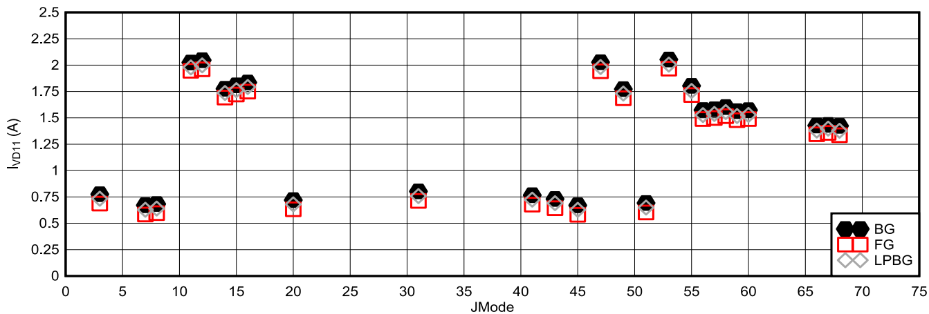
图 6-117. 双通道模式：在 5.2GSPS 时的 I_{VD11} 与 JMODE 间的关系(ADC12DJ5200RF)
