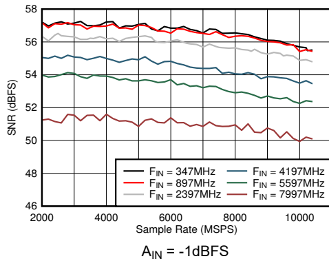
图 6-29. DES 模式：SNR 与采样率和输入频率间的关系
