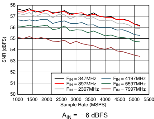
图 6-45. 双通道模式：SNR 与采样率和输入频率间的关系
