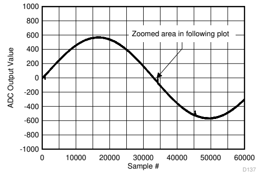
图 6-164. 后台校准内核转换 (交流信号)
