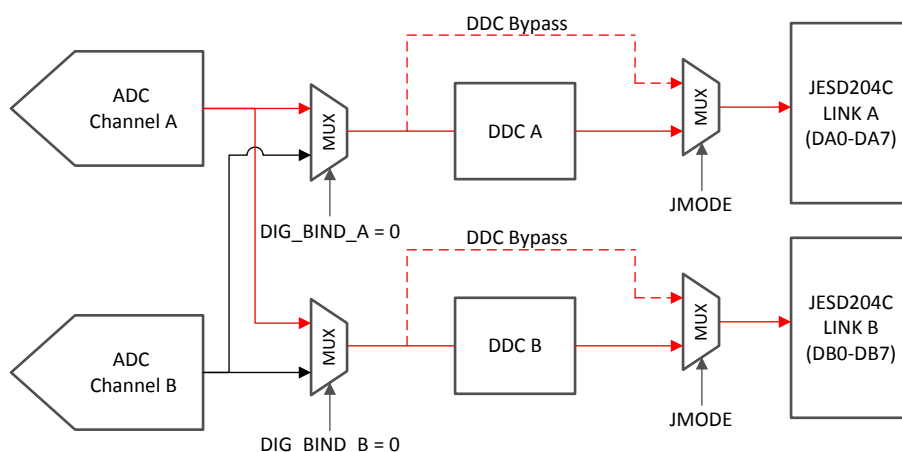
图 7-24. 通道 A 的双 DDC 模式或冗余数据模式
