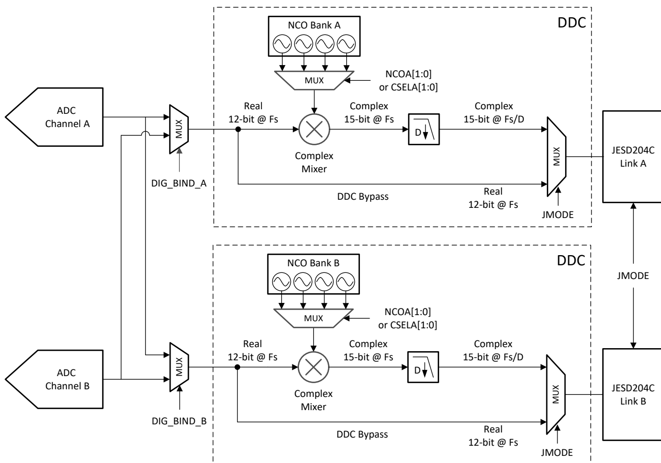
图 7-8. 双通道模式下的数字下变频块
