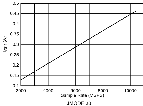
图 6-137. DES 模式： I_{VS11} 与采样率间的关系 (ADC12DJ5210RF)
