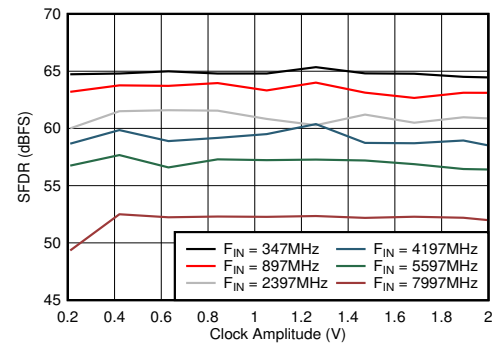
图 6-82. DES 模式：SFDR 与时钟振幅间的关系
