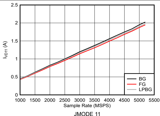
图 6-151. 双通道模式： I_{VD11} 与采样率间的关系 (ADC12DJ5210RF)
