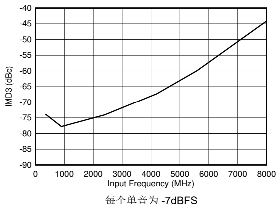
图 6-99. DES 模式：IMD3 与输入频率间的关系
