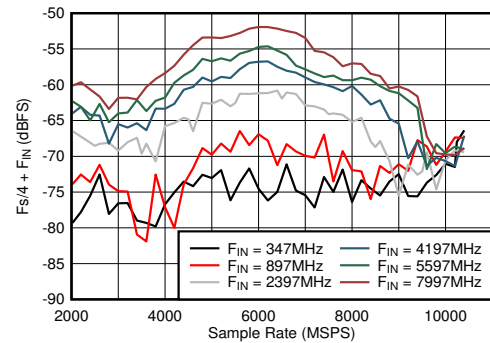
图 6-42. DES 模式：Fs/4 + F_{IN} 与采样率和输入频率间的关系
