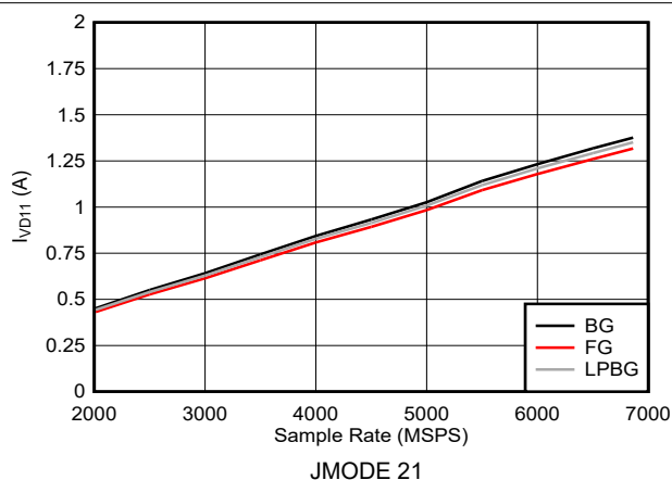
图 6-133. DES 模式： I_{VD11} 与采样率间的关系 (ADC12DJ5210RF)
