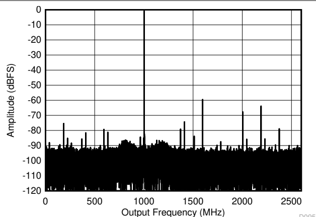
图 6-20. 双通道模式：4197MHz 时的单音 FFT
