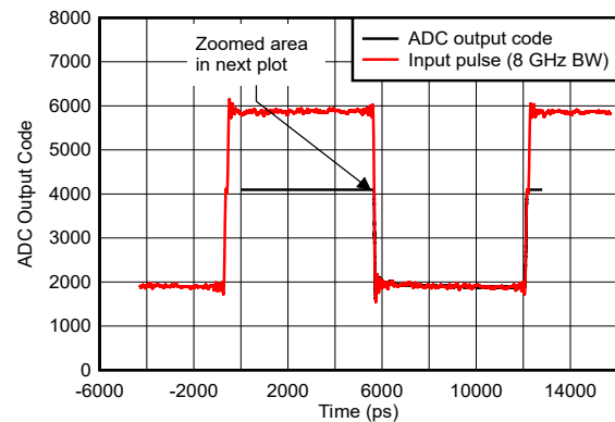
图 6-168. 脉冲过驱动恢复
