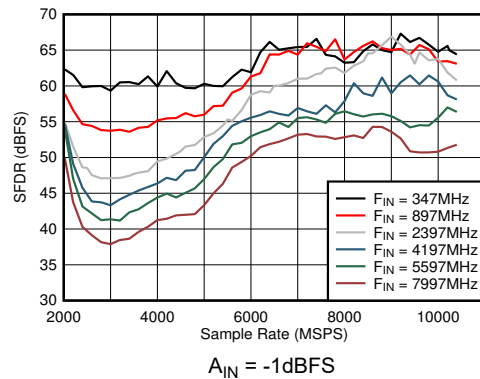
图 6-32. DES 模式：SFDR 与采样率和输入频率间的关系
