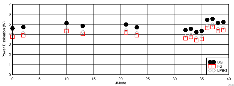
图 6-125. 具有较低最大 F_S 的其他模式： I_{VS11} 与 JMODE 间的关系 (ADC12DJ5210RF)
