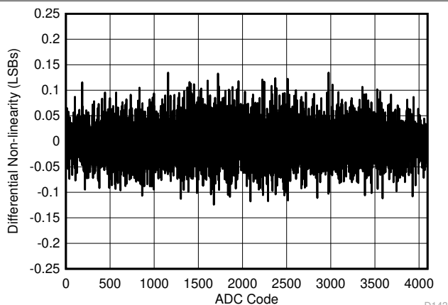
图 6-3. DNL 与 ADC 代码间的关系
