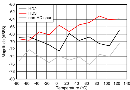
图 6-87. DES 模式：HD2、HD3 和最差非 HD 杂散与温度间的关系
