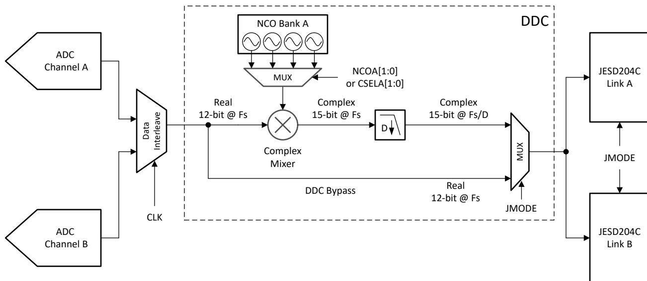
图 7-9. 单通道模式下的数字下变频块
