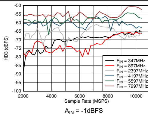
图 6-38. DES 模式：HD3 与采样率和输入频率间的关系
