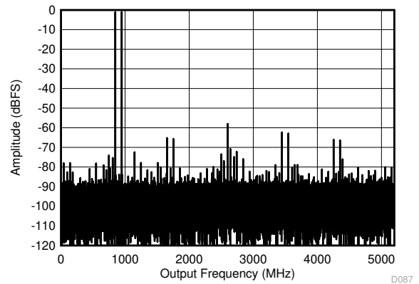
图 6-12. DES 模式：897MHz 时的双音 FFT
