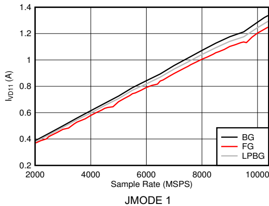
图 6-129. DES 模式: I_{VD11} 与采样率间的关系 (ADC12DJ5200RF)
