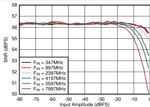
图 6-57. DES 模式：SNR 与输入振幅和频率间的关系
