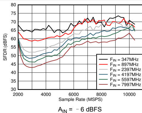
图 6-33. DES 模式：SFDR 与采样率和输入频率间的关系
