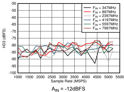
图 6-55. 双通道模式：HD3 与采样率和输入频率间的关系
