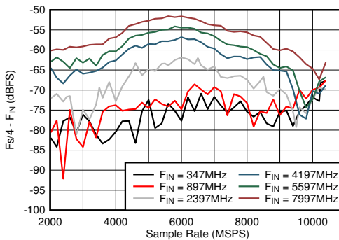
图 6-43. DES 模式：Fs/4 - F_{IN} 与采样率和输入频率间的关系
