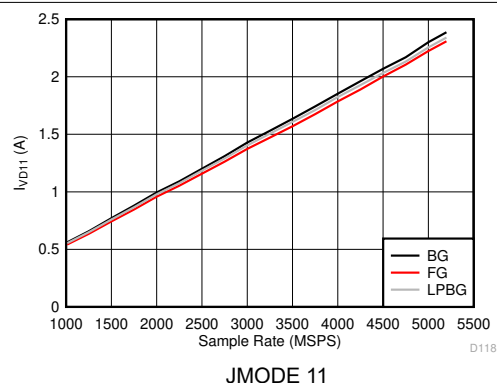
图 6-150. 双通道模式： I_{VD11} 与采样率间的关系 (ADC12DJ5200RF)
