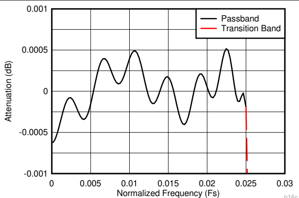
图 7-16. 16 倍抽取复合放大通带响应
