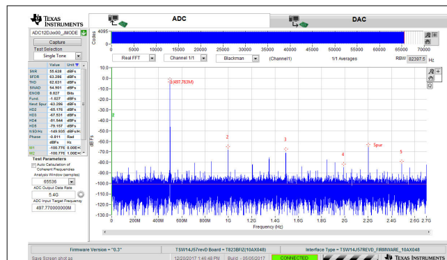
图 8-2. 针对 497.77MHz 输入信号的 FFT，5.4GSPS，JMODE0
