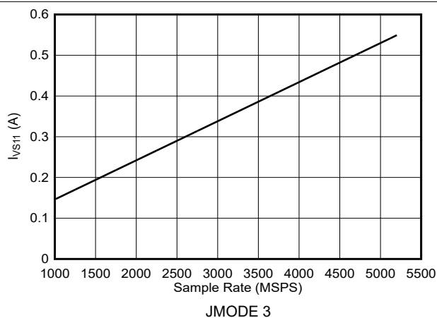
图 6-149. 双通道模式： I_{VS11} 与采样率间的关系 (ADC12DJ5210RF)
