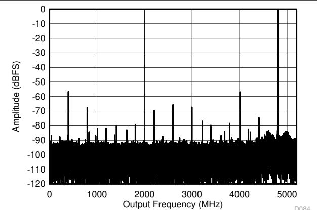
图 6-9. DES 模式：5597MHz 时的单音 FFT
