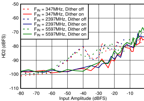
图 6-76. 双通道模式：HD2 与输入振幅和抖动间的关系
