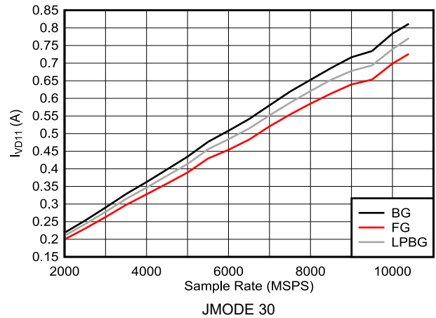
图 6-136. DES 模式： I_{VD11} 与采样率间的关系 (ADC12DJ5210RF)
