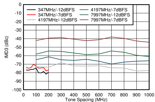
图 6-106. 双通道模式：IMD3 与频音间隔间的关系
