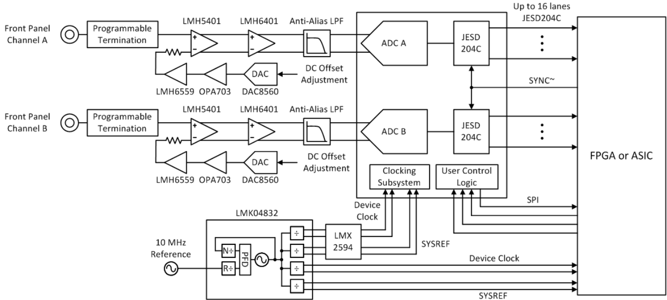
图 8-5. 可重新配置示波器的典型配置
