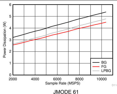
图 6-144. DES 模式：功耗与采样率间的关系
