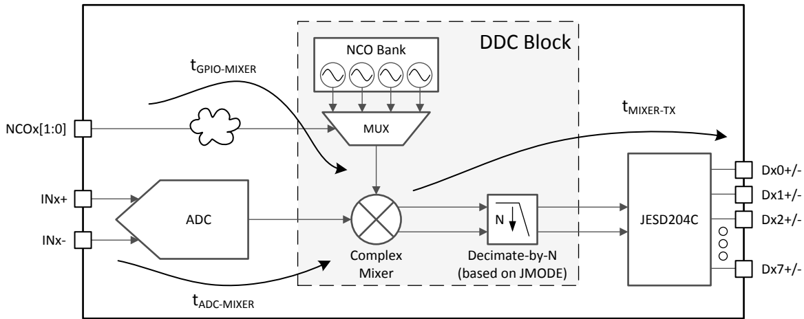
图 7-10. NCO 快速跳频延迟图
