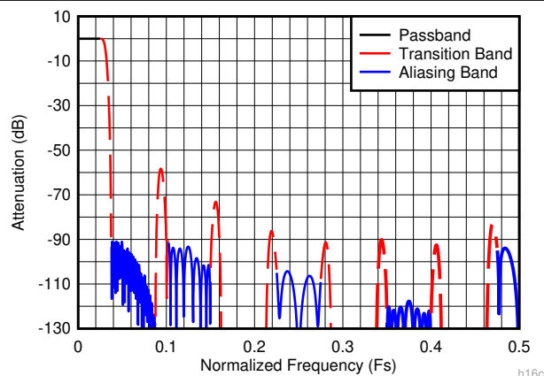
图 7-15. 16 倍抽取复合响应
