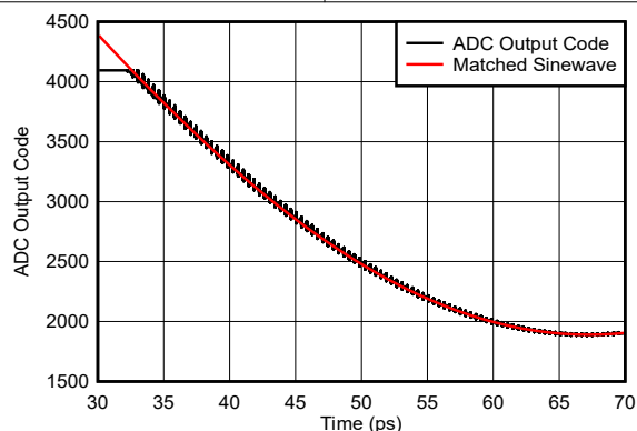
图 6-171. 正弦波过驱恢复
