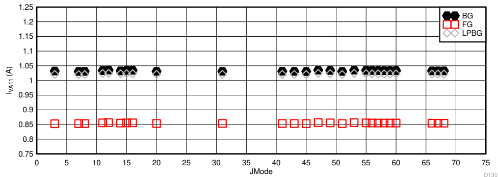
图 6-115. 双通道模式：在 5.2GSPS 时的 I_{VA19} 与 JMODE
