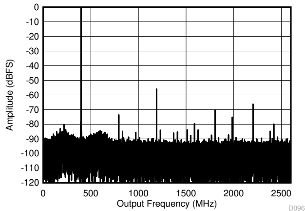
图 6-21. 双通道模式：5597MHz 时的单音 FFT
