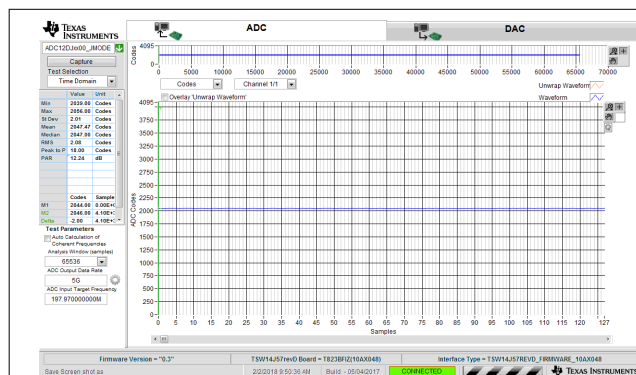
图 8-6. 5GSPS 单通道示波器的空闲通道噪声 ( 无输入 )
