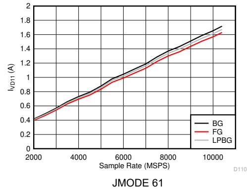
图 6-138. DES 模式： I_{VD11} 与采样率间的关系 (ADC12DJ5200RF)
