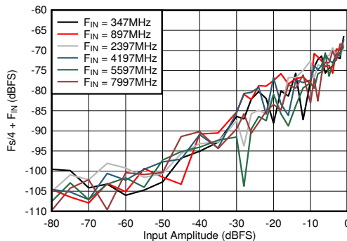
图 6-67. DES 模式： F_s/4 + F_{\text{IN}} 与输入振幅和频率间的关系
