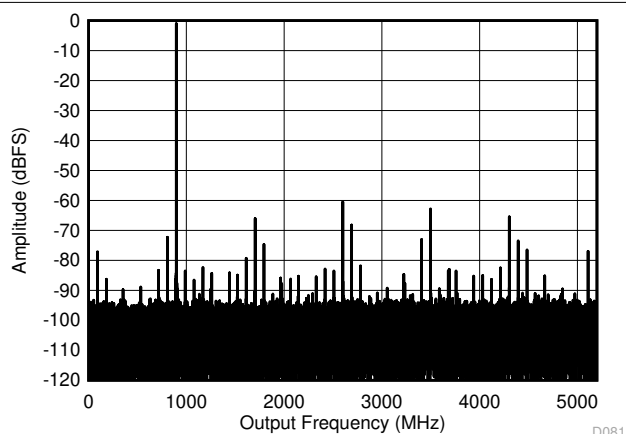
图 6-6. DES 模式：897MHz 时的单音 FFT
