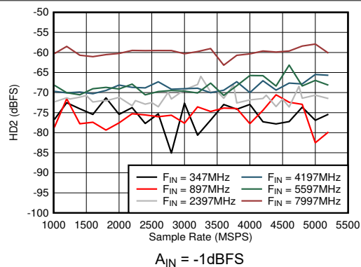
图 6-50. 双通道模式：HD2 与采样率和输入频率间的关系
