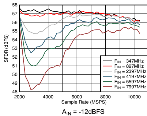
图 6-34. DES 模式：SFDR 与采样率和输入频率间的关系
