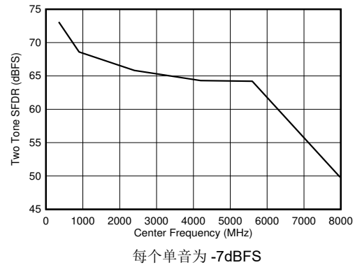
图 6-102. DES 模式：双音 SFDR 与输入频率间的关系
