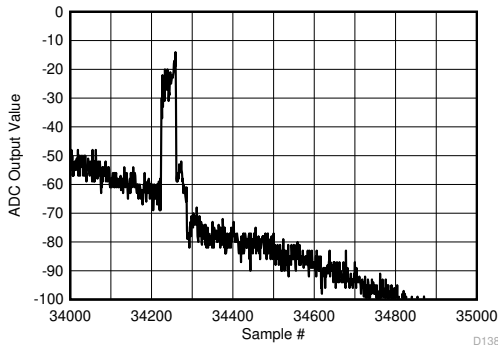
图 6-165. 后台校准内核转换 (放大交流信号)
