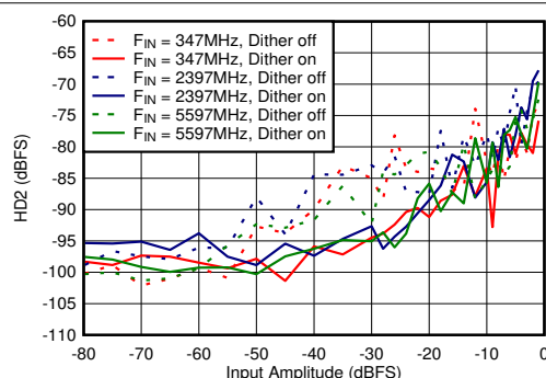
图 6-62. DES 模式：HD2 与输入振幅和抖动间的关系
