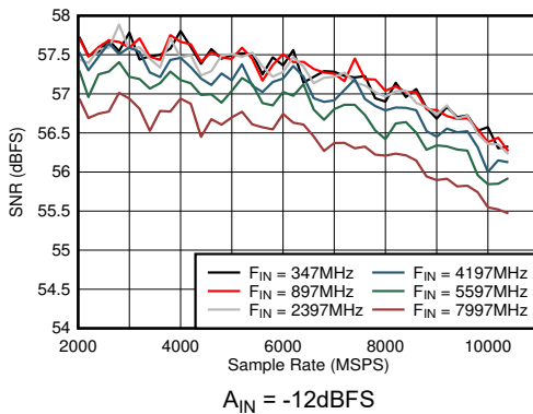
图 6-31. DES 模式：SNR 与采样率和输入频率间的关系
