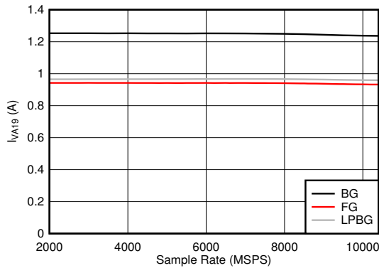
图 6-127. DES 模式: I_{VA19} 与采样率间的关系
