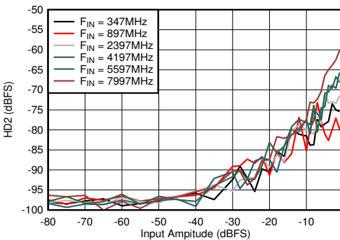
图 6-75. 双通道模式：HD2 与输入振幅和频率间的关系
