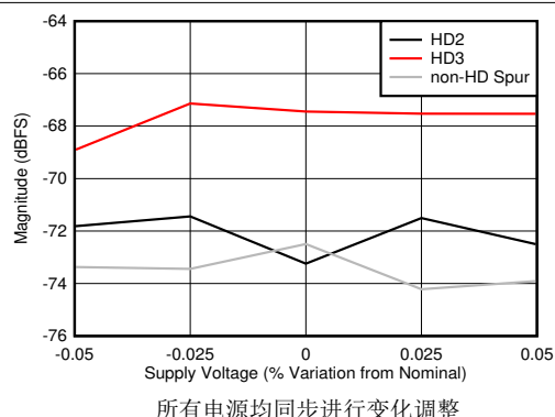
图 6-96. 双通道模式：HD2、HD3 和最差非 HD 杂散与电源电压间的关系
