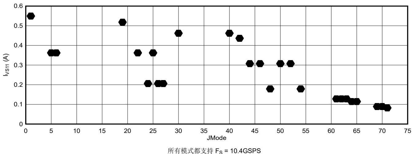
图 6-113. DES 模式：在 10.4GSPS 时的 I_{VS11} 与 JMODE 间的关系(ADC12DJ5210RF)
