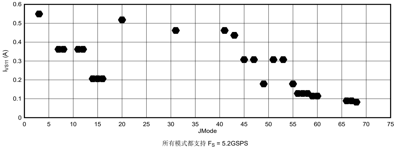
图 6-119. 双通道模式：在 5.2GSPS 时的 I_{VS11} 与 JMODE 间的关系(ADC12DJ5210RF)
