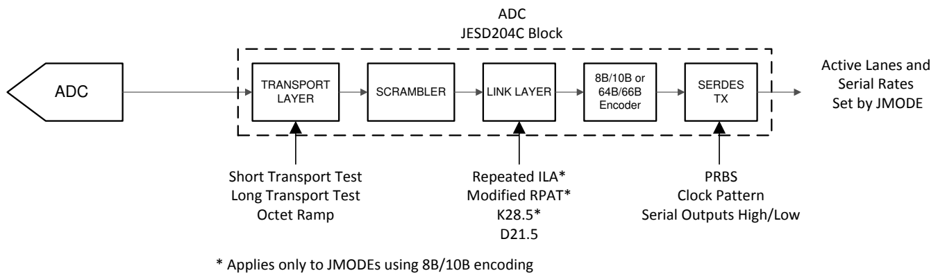
图 7-25. 测试模式插入点
