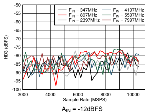
图 6-40. DES 模式：HD3 与采样率和输入频率间的关系
