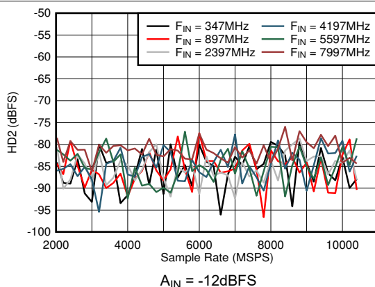
图 6-37. DES 模式：HD2 与采样率和输入频率间的关系
