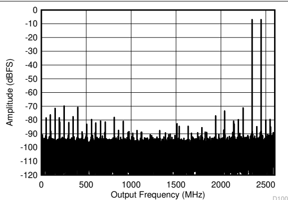
图 6-25. 双通道模式：2397MHz 时的双音 FFT
