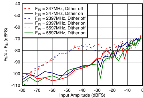
图 6-66. DES 模式： F_s/2 + F_{\text{IN}} 与输入振幅和抖动间的关系
