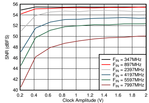
图 6-81. DES 模式：SNR 与时钟振幅间的关系
