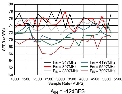
图 6-49. 双通道模式：SFDR 与采样率和输入频率间的关系
