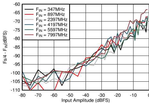
图 6-69. DES 模式： F_s/4 - F_{\text{IN}} 与输入振幅和频率间的关系
