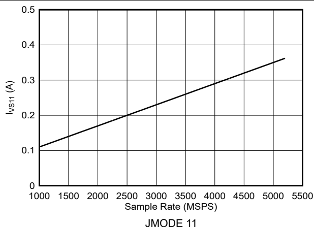
图 6-152. 双通道模式： I_{VD11} 与采样率间的关系 (ADC12DJ5210RF)
