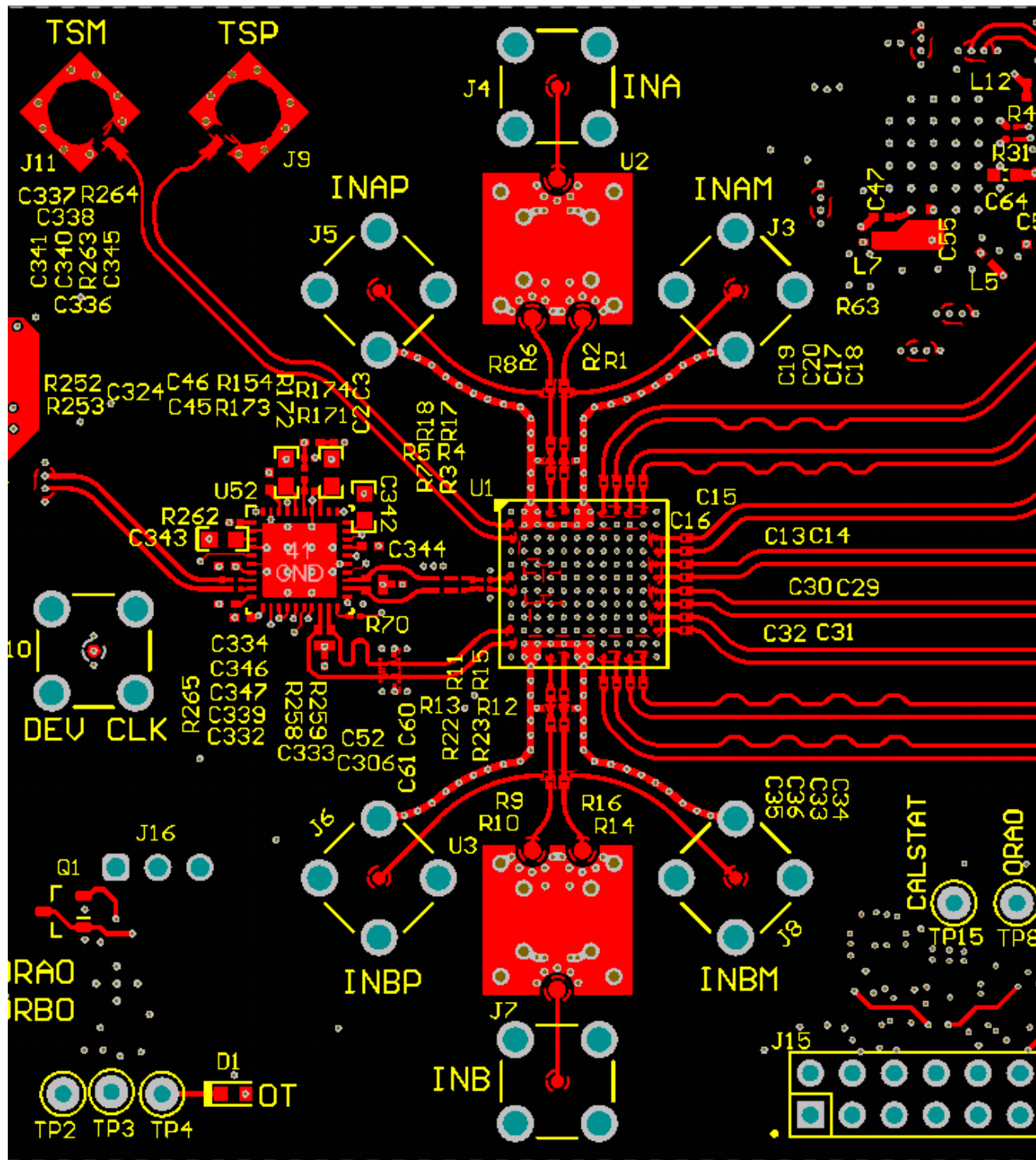
图 8-17. 顶层布线：模拟输入、CLK 和 SYSREF、DA0-3、DB0-3
