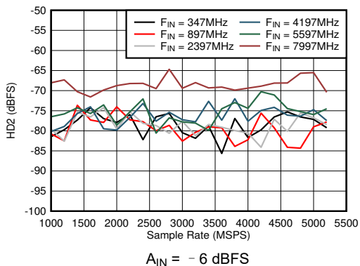
图 6-51. 双通道模式：HD2 与采样率和输入频率间的关系
