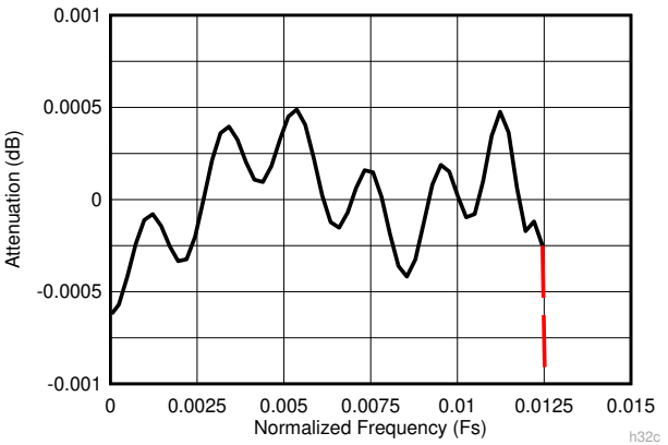
图 7-18. 32 倍抽取复合放大通带响应
