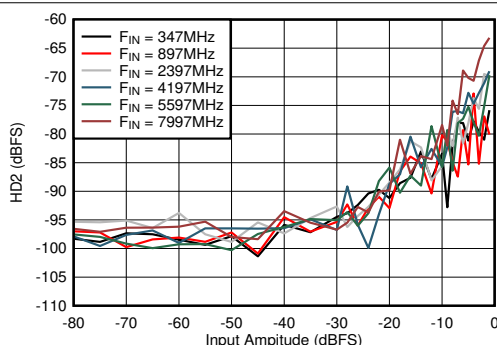
图 6-61. DES 模式：HD2 与输入振幅和频率间的关系
