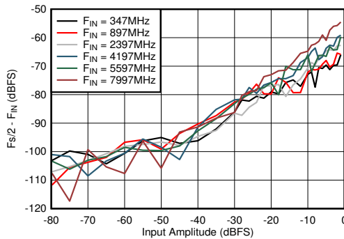
图 6-65. DES 模式： F_s/2 - F_{\text{IN}} 与输入振幅和频率间的关系
