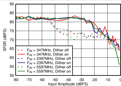
图 6-74. 双通道模式：SFDR 与输入振幅和抖动间的关系
