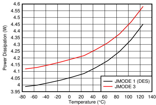
图 6-163. 功耗与温度间的关系
