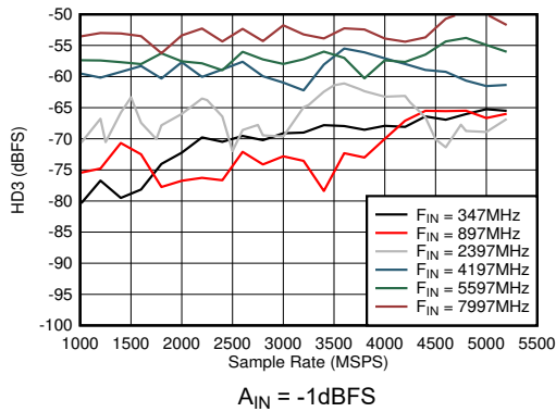
图 6-53. 双通道模式：HD3 与采样率和输入频率间的关系
