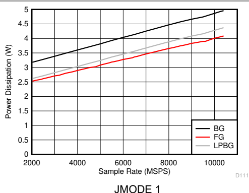
图 6-141. DES 模式：功耗与采样率间的关系
