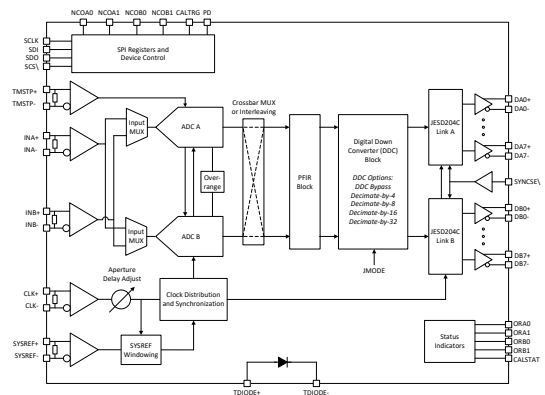
ADC12DJ52x0RF 方框图
