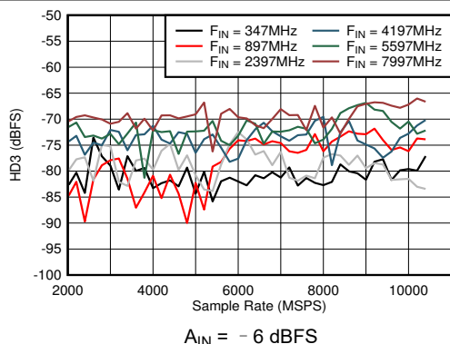
图 6-39. DES 模式：HD3 与采样率和输入频率间的关系
