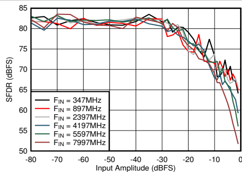
图 6-73. 双通道模式：SFDR 与输入振幅和频率间的关系
