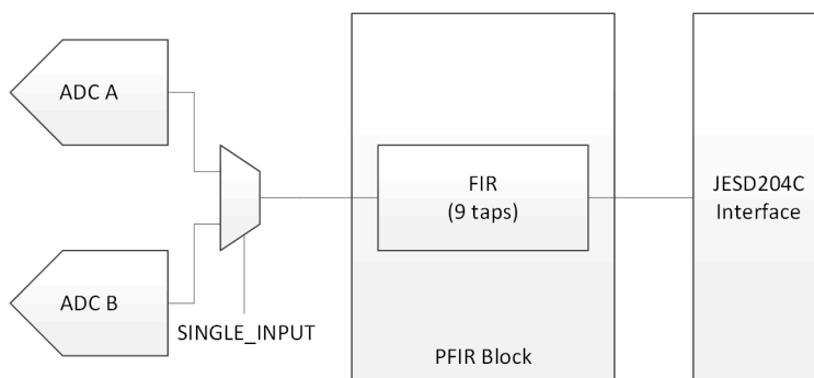
图 7-5. 单通道均衡 PFIR 方框图
