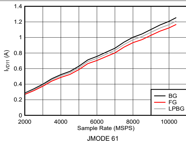
图 6-139. DES 模式： I_{VD11} 与采样率间的关系 (ADC12DJ5210RF)
