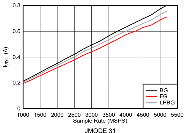
图 6-154. 双通道模式: I_{VD11} 与采样率间的关系 (ADC12DJ5210RF)
