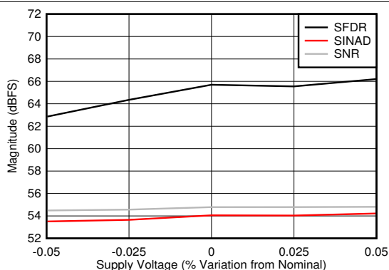
图 6-95. 双通道模式：SNR、SINAD 和 SFDR 与电源电压间的关系
