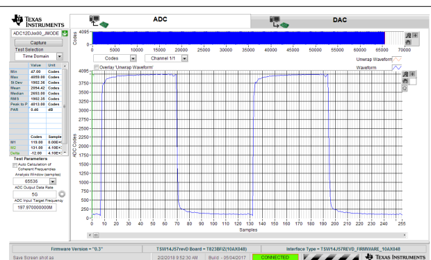
图 8-7. 5GSPS 单通道示波器的 40MHz 方波时域
