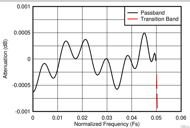
图 7-14. 8 倍抽取复合放大通带响应
