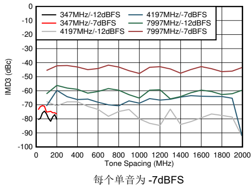
图 6-101. DES 模式：IMD3 与频音间隔间的关系
