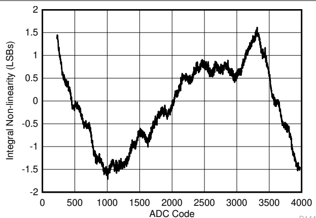
图 6-4. INL 与 ADC 代码间的关系
