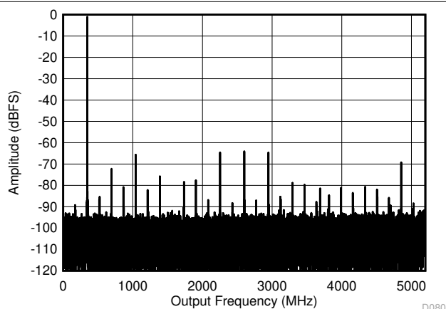
图 6-5. DES 模式：347MHz 时的单音 FFT
