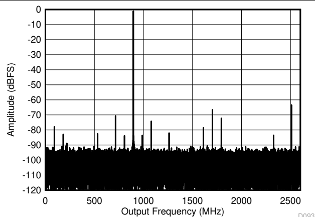
图 6-18. 双通道模式：897MHz 时的单音 FFT
