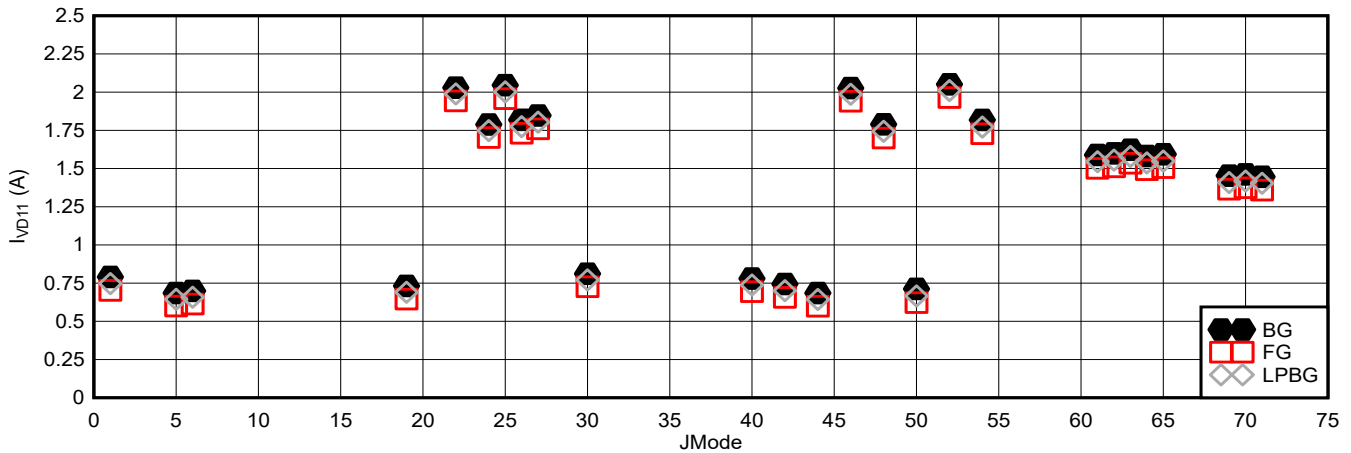
图 6-111. DES 模式：在 10.4GSPS 时的 I_{VD11} 与 JMODE 间的关系 (ADC12DJ5200RF)
