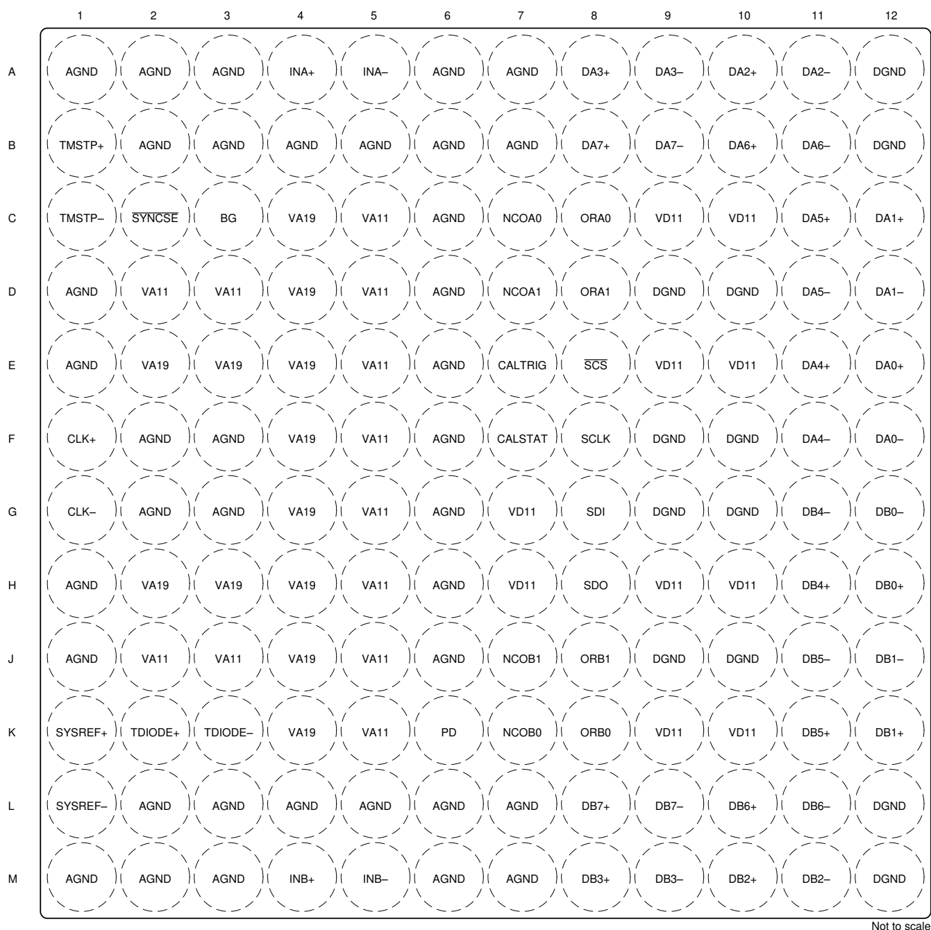
图 5-1. ADC12DJ5200RF AAV 封装、144 焊球倒装芯片 BGA (顶视图)
