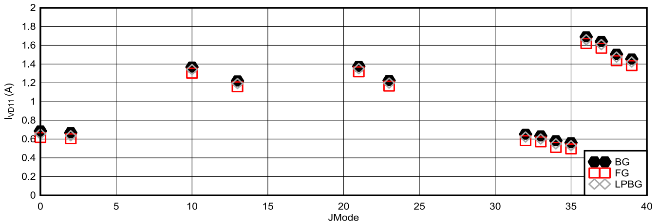
图 6-123. 具有较低最大 F_S 的其他模式： I_{VD11} 与 \text{JMODE} 间的关系 (ADC12DJ5200RF)
