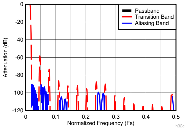
图 7-17. 32 倍抽取复合响应
