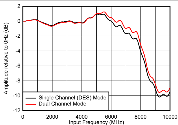
图 6-1. 输入振幅与输入频率间的关系
