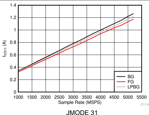
图 6-153. 双通道模式: I_{VD11} 与采样率间的关系 (ADC12DJ5200RF)
