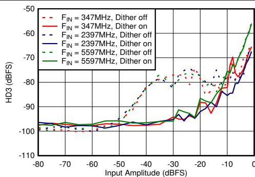
图 6-78. 双通道模式：HD3 与输入振幅和抖动间的关系
