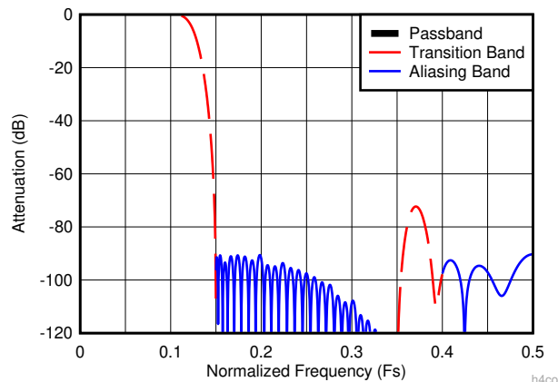
图 7-11. 4 倍抽取复合响应
