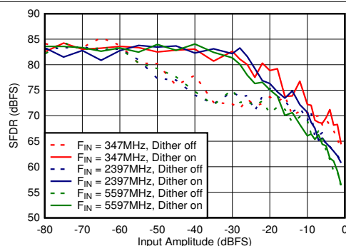
图 6-60. DES 模式：SFDR 与输入振幅和抖动间的关系
