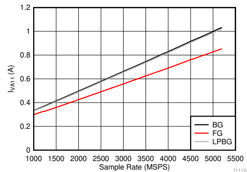
图 6-146. 双通道模式： I_{VA11} 与采样率间的关系
