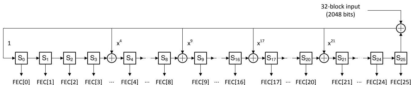
图 7-22. FEC 奇偶校验位发生器
