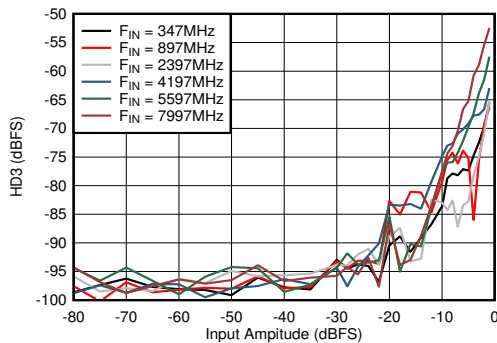
图 6-63. DES 模式：HD3 与输入振幅和频率间的关系
