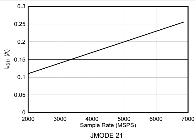
图 6-134. DES 模式： I_{VS11} 与采样率间的关系 (ADC12DJ5210RF)
