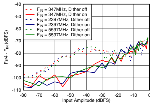
图 6-70. DES 模式： F_s/4 - F_{\text{IN}} 与输入振幅和抖动间的关系
