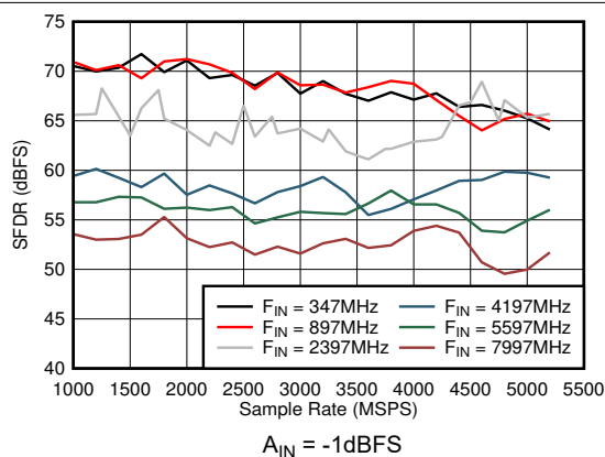
图 6-47. 双通道模式：SFDR 与采样率和输入频率间的关系
