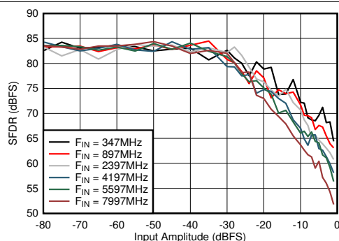
图 6-59. DES 模式：SFDR 与输入振幅和频率间的关系
