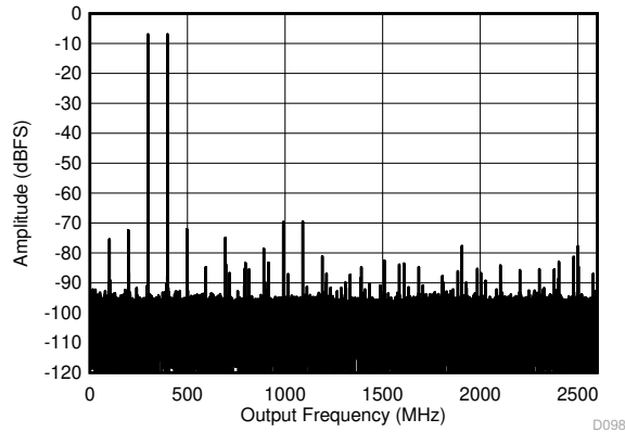
图 6-21. 双通道模式：5597MHz 时的单音 FFT
