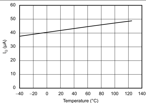
图 6-35. 静态电流与温度间的关系
