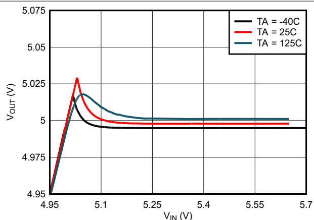
图 6-12. 各种温度下 V_{OUT} 与 V_{IN} 间的关系
