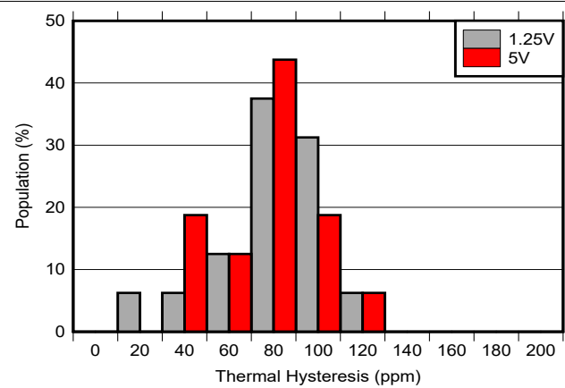
图 6-28. 热迟滞直方图 0°C to 70°C 周期 1
