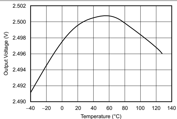
图 6-32. 输出电压与温度间的关系
