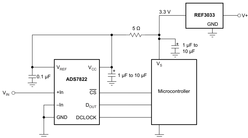
图 7-4. 基本数据采集系统 1
