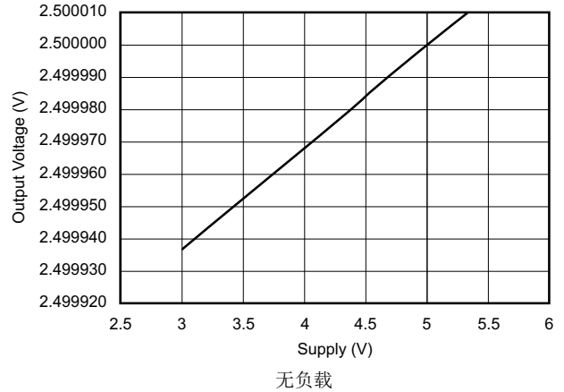
图 6-39. 输出电压与电源电压之间的关系
