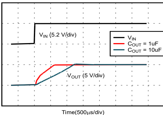
图 6-17. 阶跃响应启动
