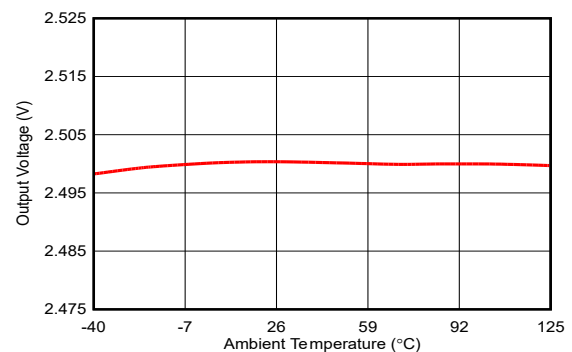
输出电压与温度间的关系 (REF3025E)
