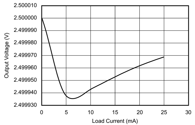
图 6-41. 输出电压与负载电流间的关系
