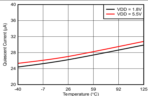
图 6-8. 静态电流与温度间的关系 V_{OUT} = 1.25\text{V}
