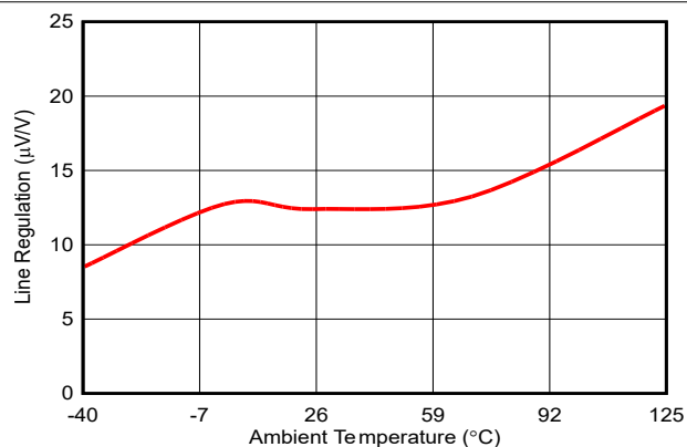
图 6-10. 线路调整率与温度间的关系 V_{OUT} = 2.5\text{V}
