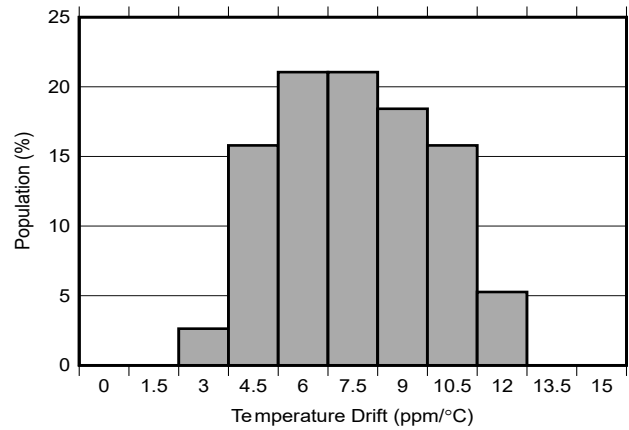
图 6-2. 温漂直方图 ( -40°C 至 +85°C )
