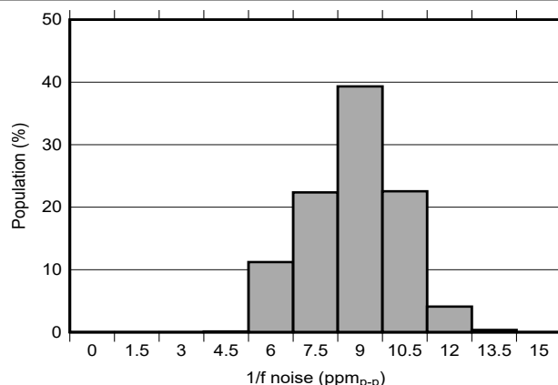
图 6-21. 闪烁噪声直方图
