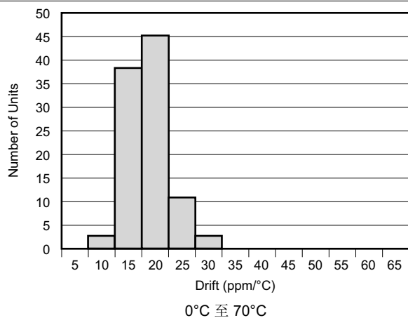
图 6-30. 温漂
