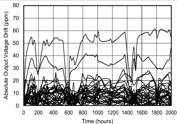
图 6-52. 长期稳定性：0 到 2000 小时
