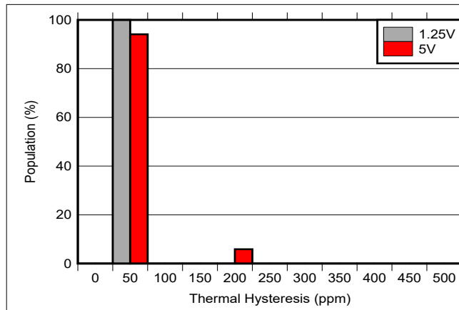
图 6-25. 热迟滞直方图 -40°C to 125°C 周期 2
