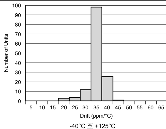
图 6-31. 温漂
