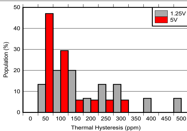
图 6-24. 热迟滞直方图 -40°C to 125°C 周期 1
