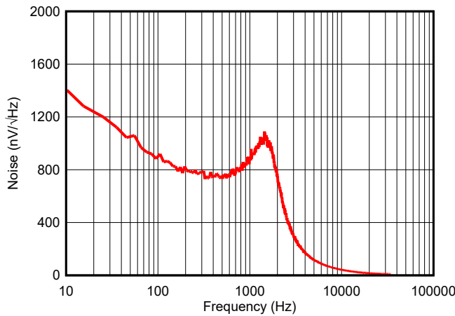
图 6-13. 噪声频谱密度与频率间的关系
