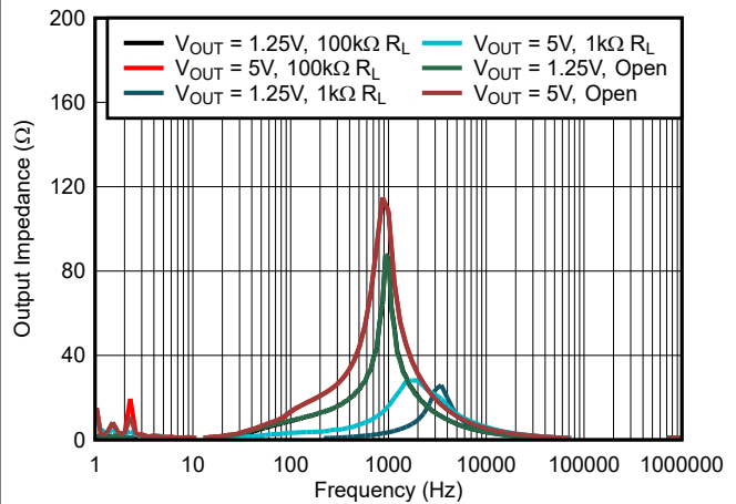
图 6-14. 输出阻抗与频率间的关系
