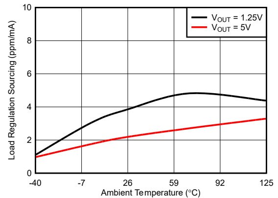
图 6-6. 负载调整率 ( 拉电流 ) 与温度间的关系
