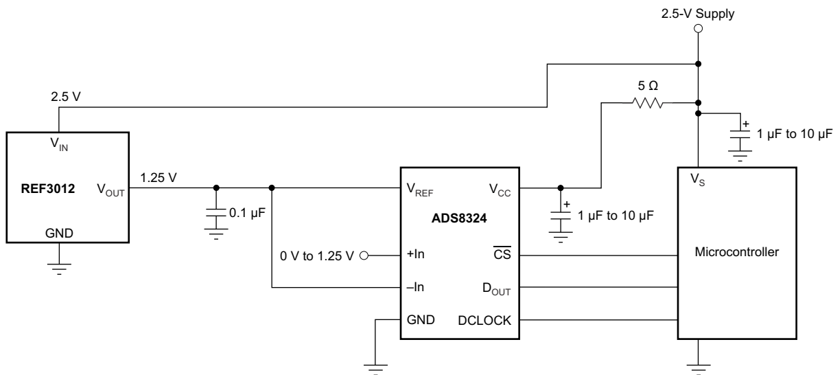
图 7-5. 基本数据采集系统 2
