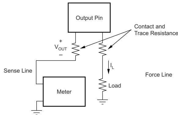
图 7-2. REF30 的准确负载调节
