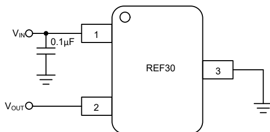
图 8-1. 运行 REF30 的典型连接
