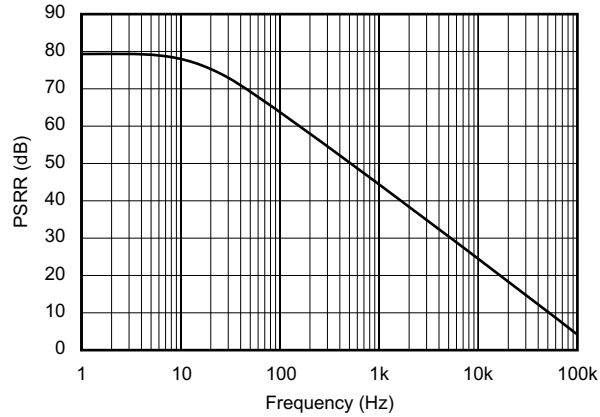
图 6-38. 电源抑制比与频率间的关系
