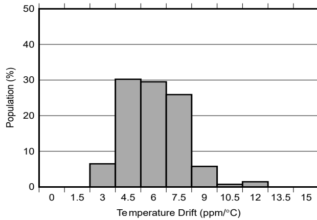
图 6-1. 温漂直方图 ( -40°C 至 +125°C )
