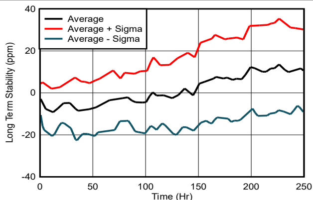
图 6-22. 长期稳定性: 0 到 250 小时
