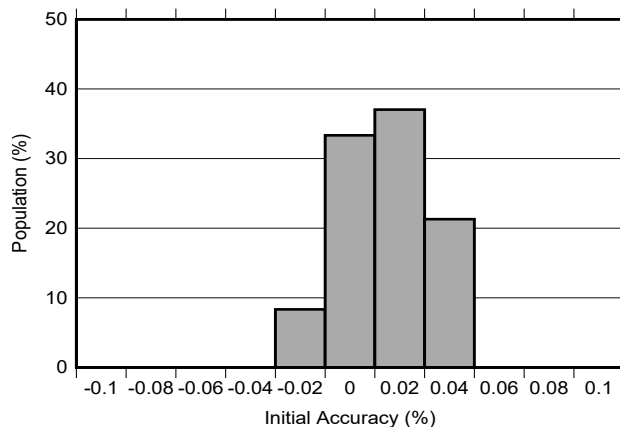
图 6-5. 初始精度
