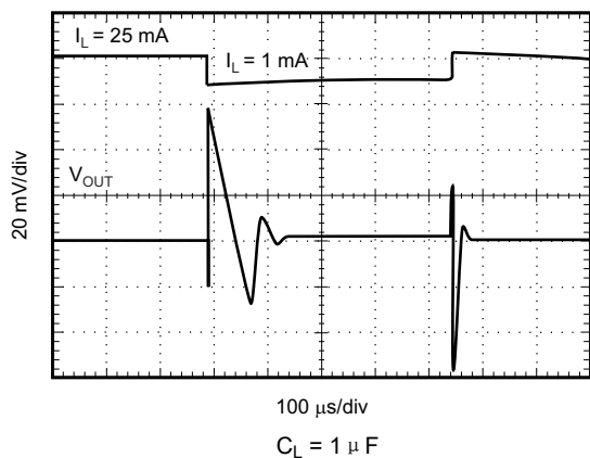
图 6-48. 1mA 至 25mA 负载瞬态
