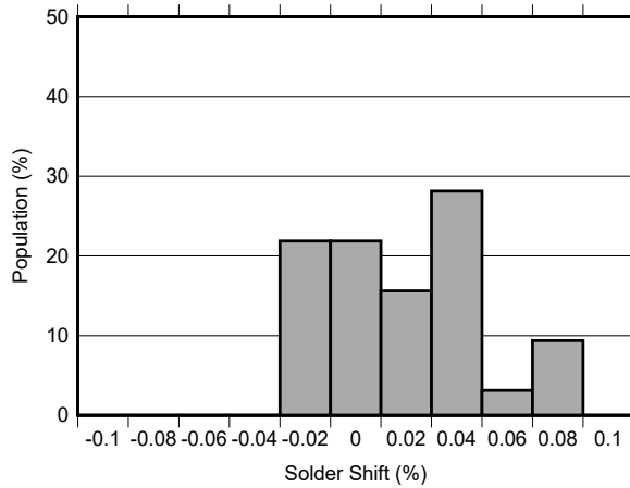
图 6-15. 焊接漂移直方图
