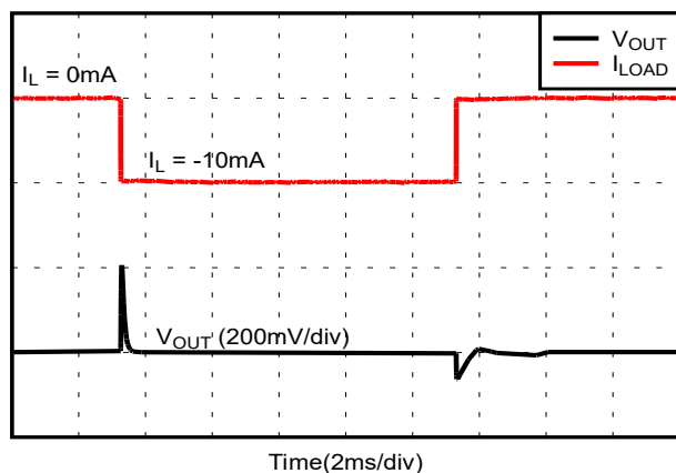
图 6-19. 负载瞬态响应 (灌电流)
