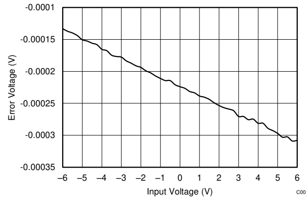
图 8-4. OPA317 输出电压误差与输入电压之间的关系
