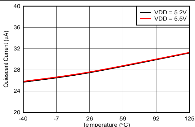
图 6-9. 静态电流与温度间的关系 V_{OUT} = 5\text{V}
