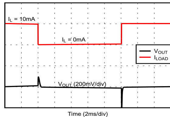
图 6-18. 负载瞬态响应 (拉电流)
