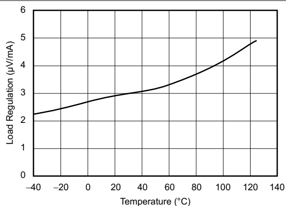
图 6-34. 负载调节与温度之间的关系
