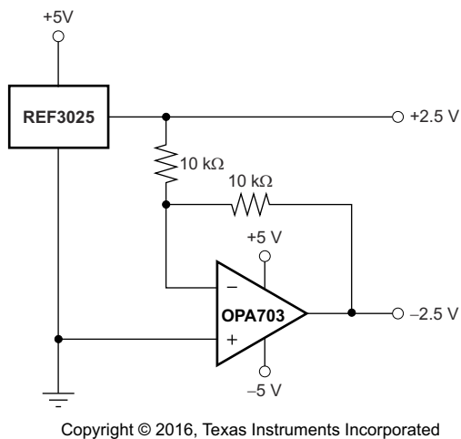
图 7-3. REF3025 与 OPA703 结合使用可产生正和负基准电压。
