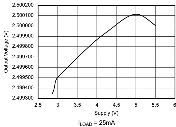
图 6-40. 输出电压与电源电压之间的关系
