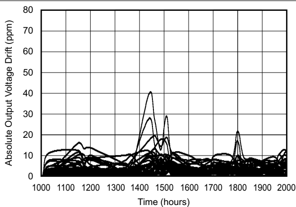
图 6-51. 长期稳定性：1000 到 2000 小时
