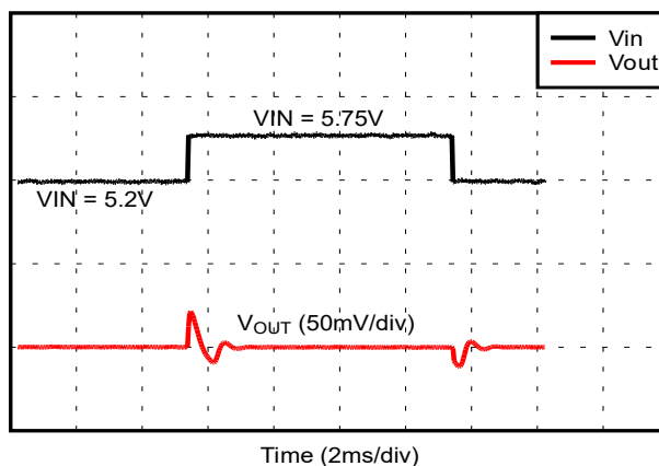
图 6-20. 线路瞬态响应
