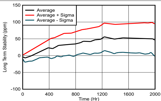
图 6-23. 长期稳定性: 0 到 2000 小时
