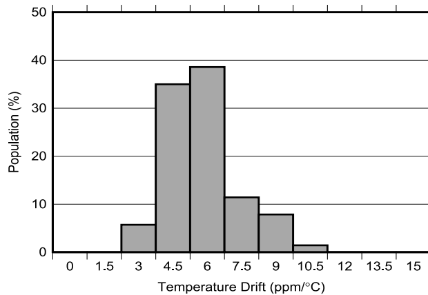
图 6-3. 温漂直方图 ( 0°C 至 +70°C )
