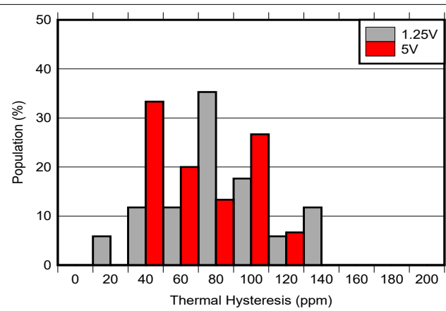
图 6-26. 热迟滞直方图 -40°C to 85°C 周期 1
