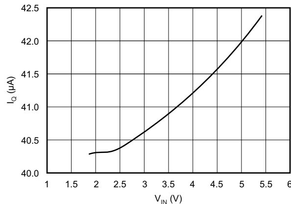
图 7-1. 电源电流与电源电压间的关系
