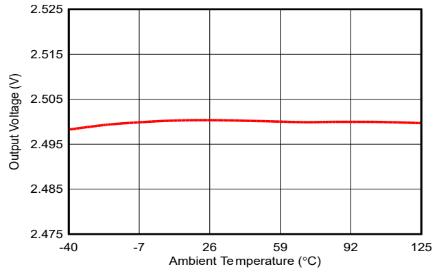
图 6-4. 输出电压与温度间的关系 V_{OUT} = 2.5\text{V}
