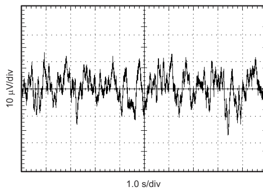
图 6-49. 0.1Hz 至 10Hz 噪声
