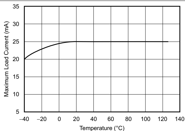
图 6-33. 最大负载电流与温度之间的关系
