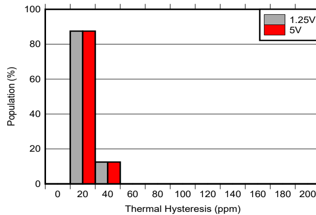
图 6-29. 热迟滞直方图 0°C to 70°C 周期 2
