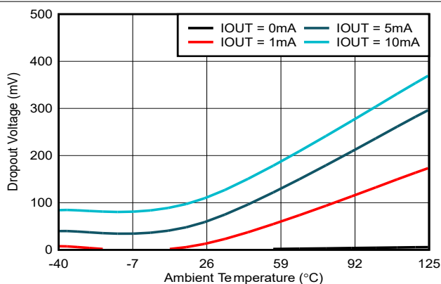
图 6-11. 压降电压与温度间的关系
