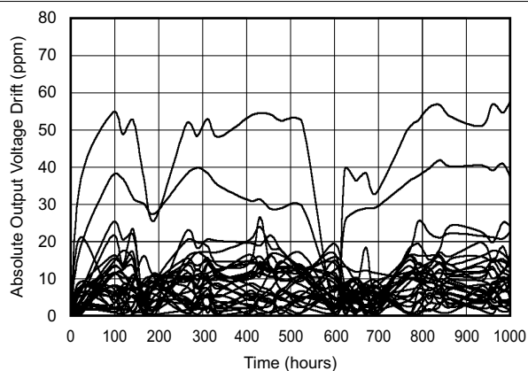
图 6-50. 长期稳定性：0 到 1000 小时
