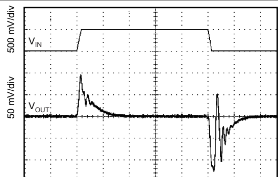
10 \mu\text{s}/\text{div} 图 6-44. 线路瞬态响应
