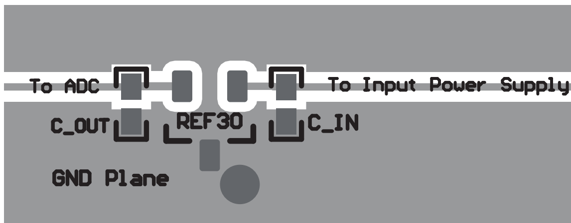
图 8-6. 布局示例
