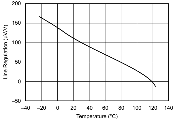
图 6-36. 线路调整率与温度间的关系
