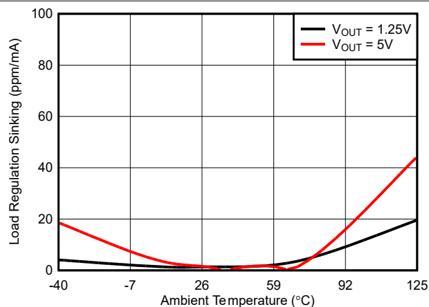
图 6-7. 负载调整率 (灌电流) 与温度间的关系
