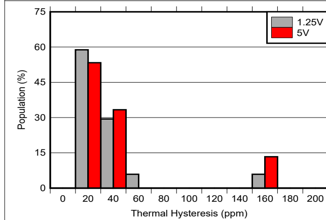
图 6-27. 热迟滞直方图 -40°C to 85°C 周期 2
