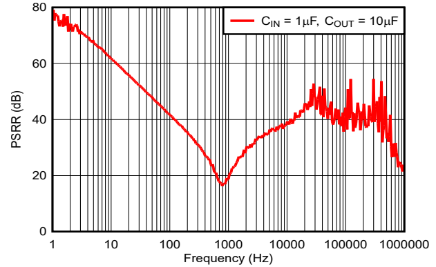
图 6-16. 电源抑制比与频率间的关系
