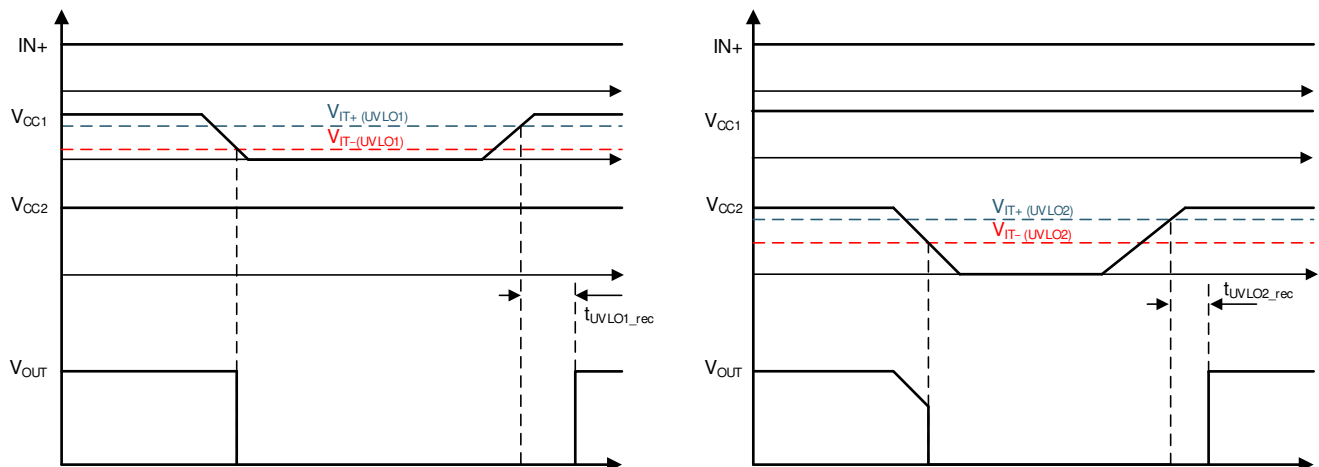
图 8-9. UVLO 功能
