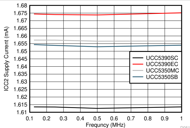
图 6-21. I_{CC2} 电源电流与输入频率间的关系
