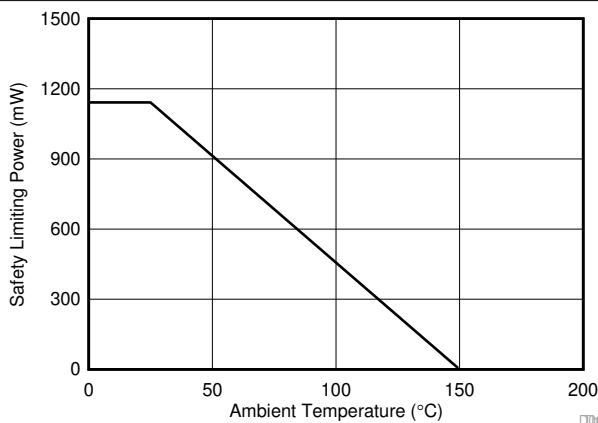
图 6-3. D 封装根据 VDE 标准限制功率的热降额曲线
