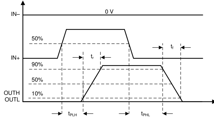
图 7-1. t_{PLH} 和 t_{PLH} 传播延迟，同相配置
