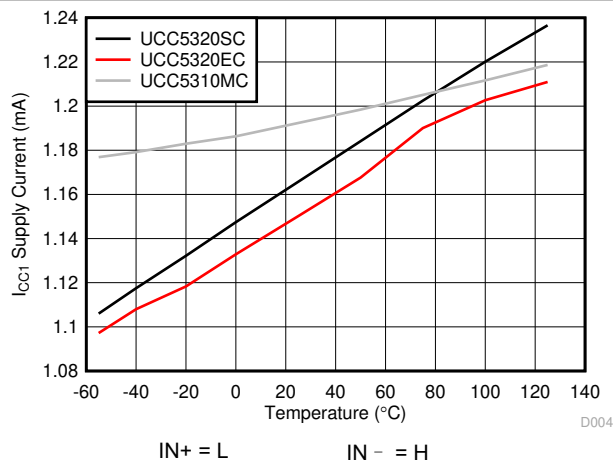
图 6-10. I_{CC1} 电源电流与温度间的关系
