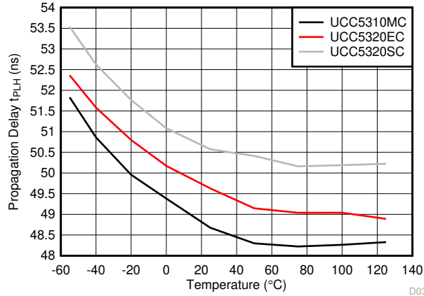
图 6-31. 传播延迟时间 t_{PLH} 与温度间的关系
