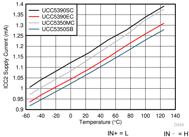
图 6-17. I_{CC2} 电源电流与温度间的关系
