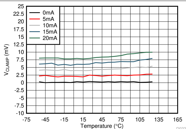
图 6-25. UCC5350M V_{Clamp} 与温度间的关系
