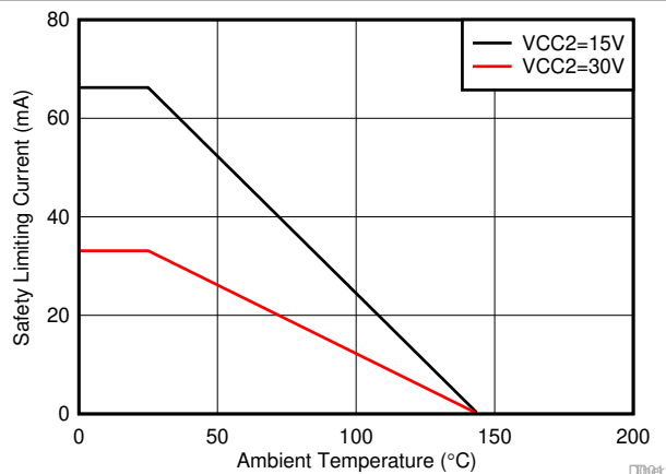
图 6-2. DWV 封装根据 VDE 标准限制电流的热降额曲线
