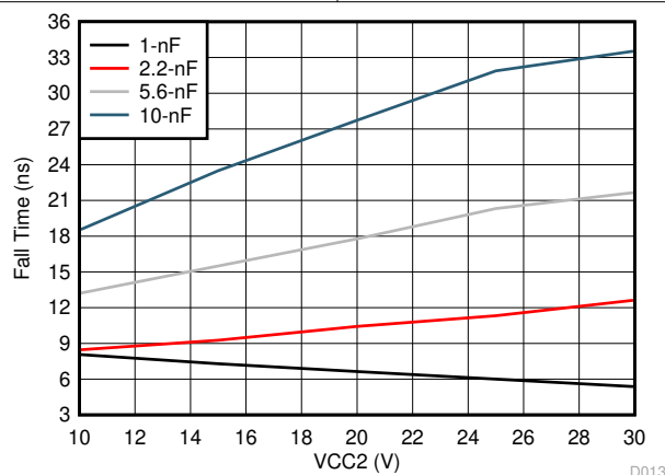
图 6-41. UCC5350SBD 下降时间与 C_L 和 V_{CC2} 间的关系
