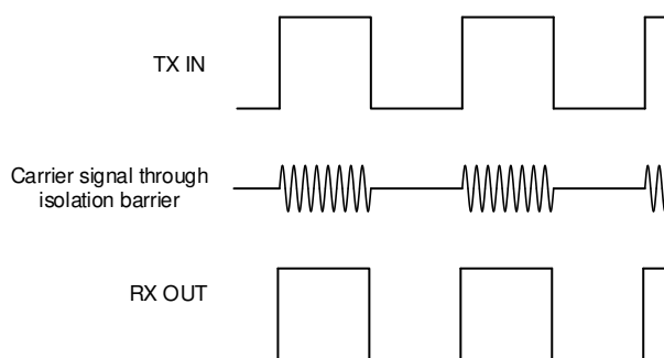
图 8-2. 基于开关键控 (OOK) 的调制方案
