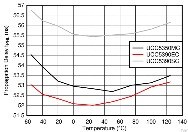
图 6-35. 传播延迟时间 t_{PLH} 与温度间的关系
