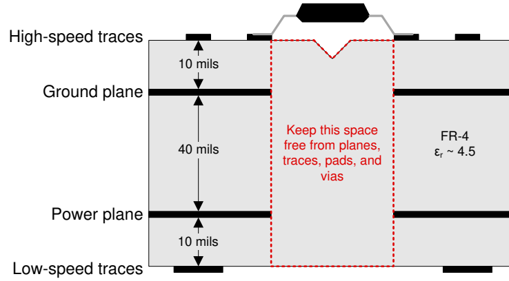
图 11-5. 建议的层堆叠
