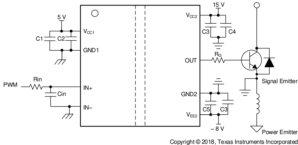
图 9-3. UCC5320E 和 UCC5390E 用于驱动 IGBT 的典型应用电路
