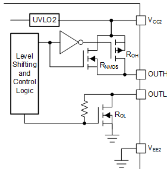
图 8-6. 输出级 — S 版本
