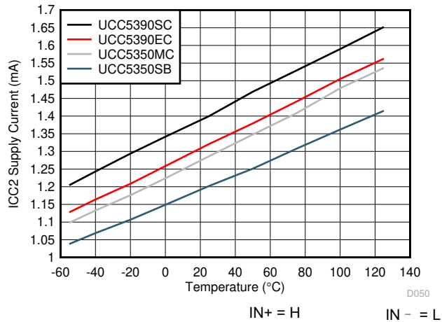
图 6-19. I_{CC2} 电源电流与温度间的关系
