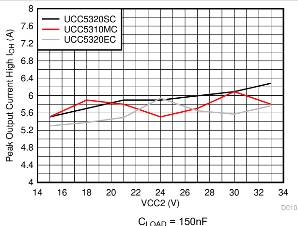
图 6-5. 输出高驱动电流与输出电压间的关系
