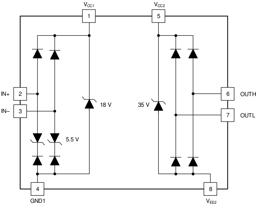
图 8-10. ESD 结构
