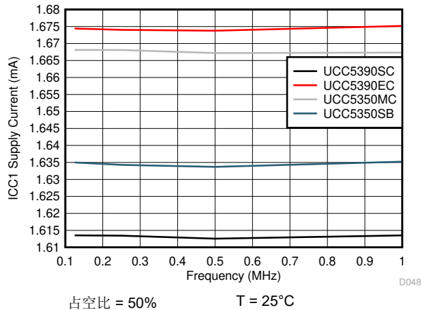
图 6-15. I_{CC1} 电源电流与输入频率间的关系
