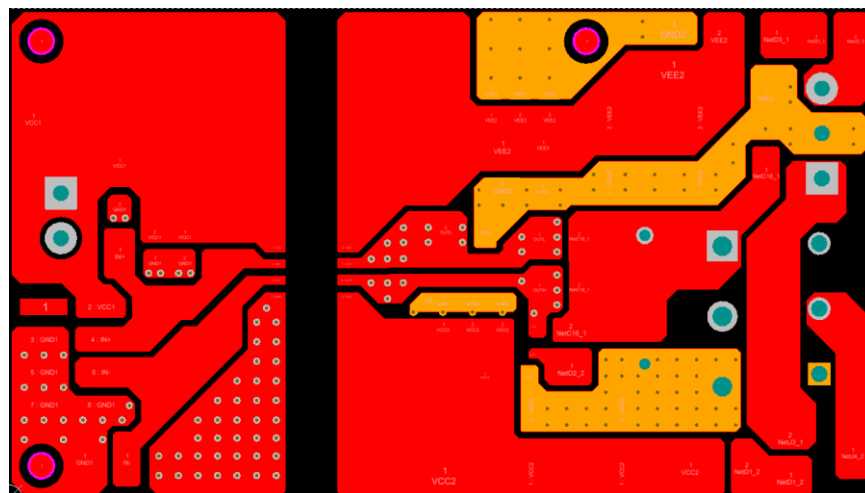
图 11-2. 顶层布线和覆铜
