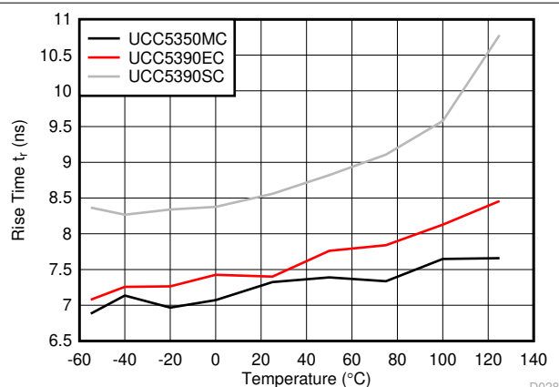
图 6-28. 上升时间与温度间的关系
