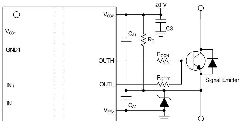
图 9-4. 利用 Iso 偏置电源输出上的齐纳二极管生成负偏置
