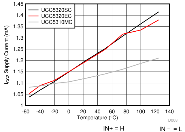
图 6-18. I_{CC2} 电源电流与温度间的关系
