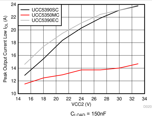
图 6-9. 输出低驱动电流与输出电压间的关系
