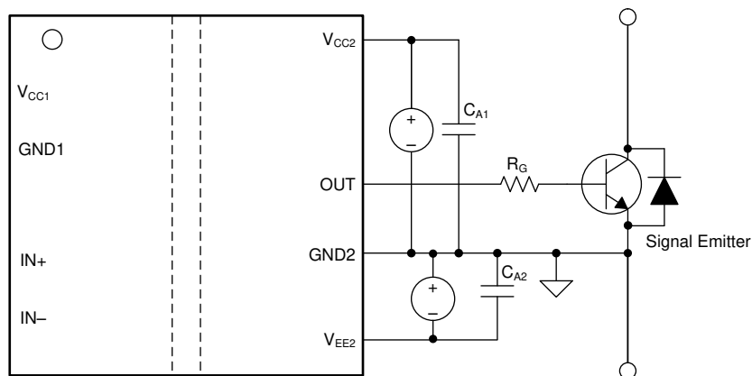
图 9-5. 利用两个 Iso 偏置电源 (UCC5320E 和 UCC5390E) 生成负偏置
