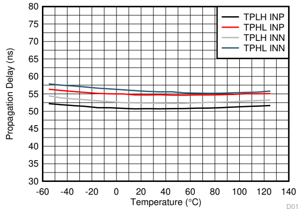
图 6-33. UCC5350SBD 传播延迟与温度间的关系
