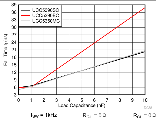
图 6-40. 下降时间与负载电容间的关系
