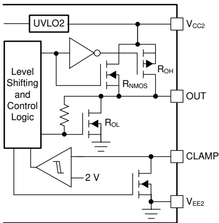
图 8-8. 输出级 — M 版本
