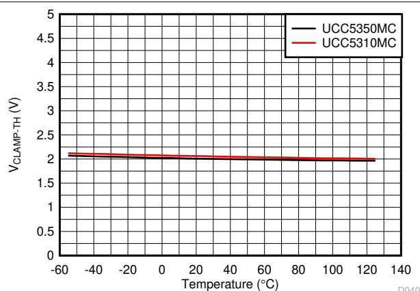
图 6-26. V_{Clamp-TH} 与温度间的关系
