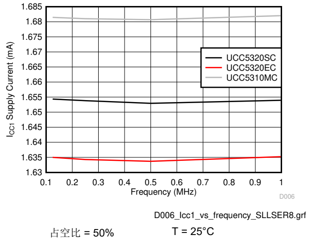
图 6-14. I_{CC1} 电源电流与输入频率间的关系
