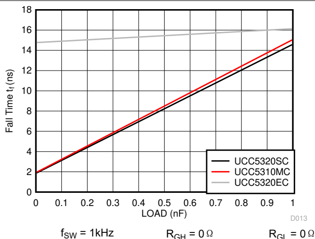
图 6-39. 下降时间与负载电容间的关系
