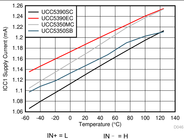
图 6-11. I_{CC1} 电源电流与温度间的关系
