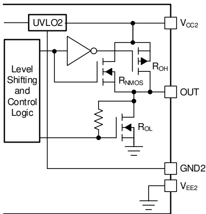
图 8-7. 输出级 — E 版本
