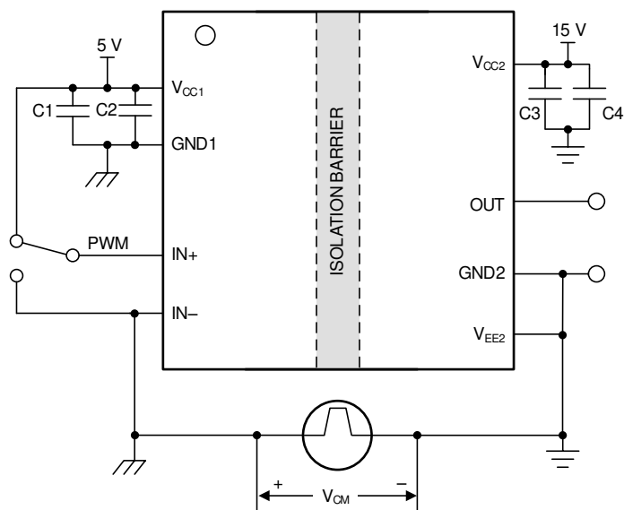
图 7-5. 相对于 GND2 的 UVLO2 的 CMTI 测试电路 (UCC53x0E)
