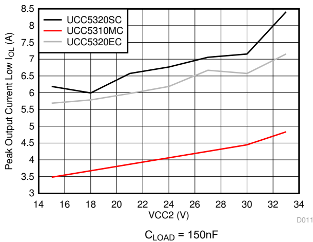
图 6-8. 输出低驱动电流与输出电压间的关系
