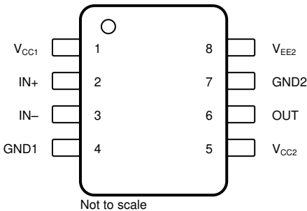
图 5-3. UCC5320E 和 UCC5390E 8 引脚 SOIC 顶视图
