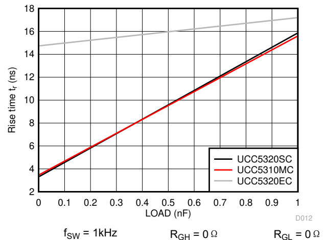
图 6-36. 上升时间与负载电容间的关系
