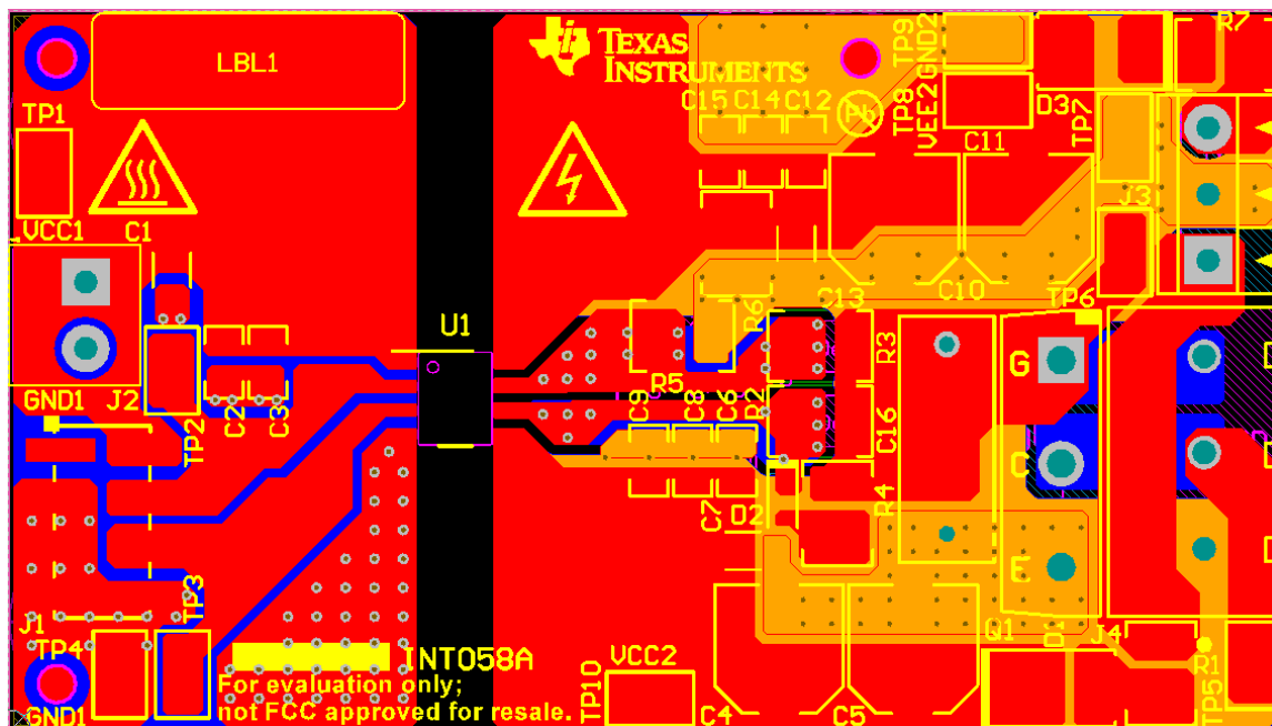
图 11-1. 布局示例
