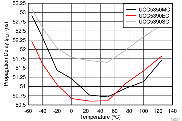
图 6-32. 传播延迟时间 t_{PLH} 与温度间的关系
