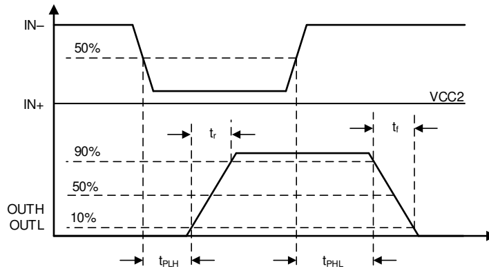
图 7-2. t_{PLH} 和 t_{PLH} 传播延迟，反相配置
