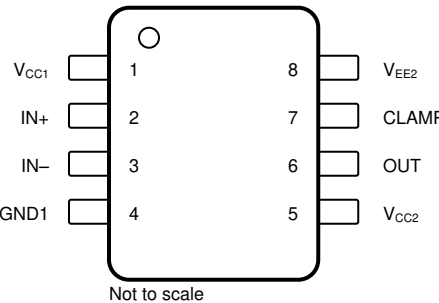
图 5-2. UCC5310M 和 UCC5350M 8 引脚 SOIC 顶视图
