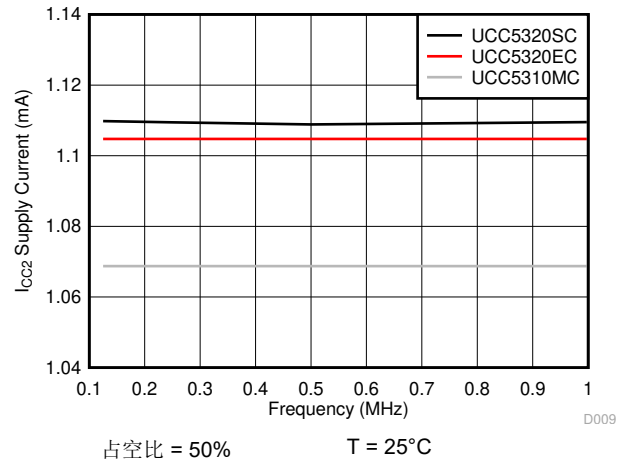
图 6-20. I_{CC2} 电源电流与输入频率间的关系
