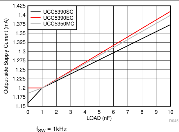
图 6-23. I_{CC2} 电源电流与负载电容间的关系
