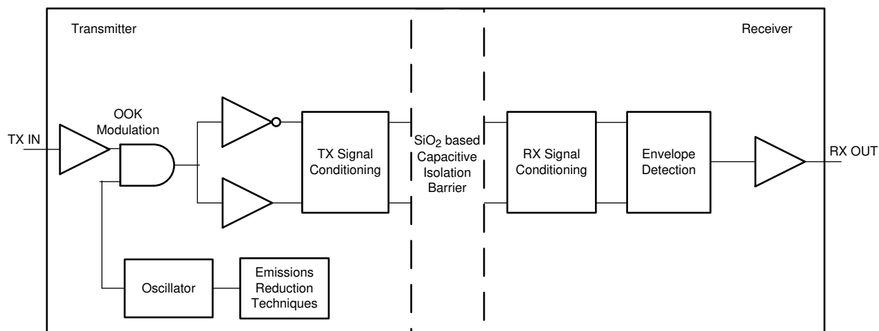
图 8-1. 电容数据通道的概念方框图
