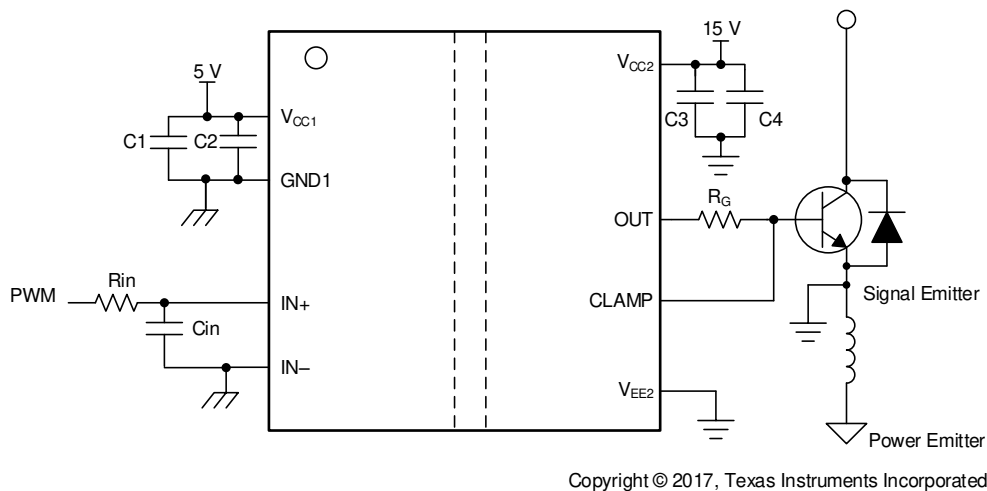
图 9-2. UCC5310M 和 UCC5350M 用于驱动 IGBT 的典型应用电路
