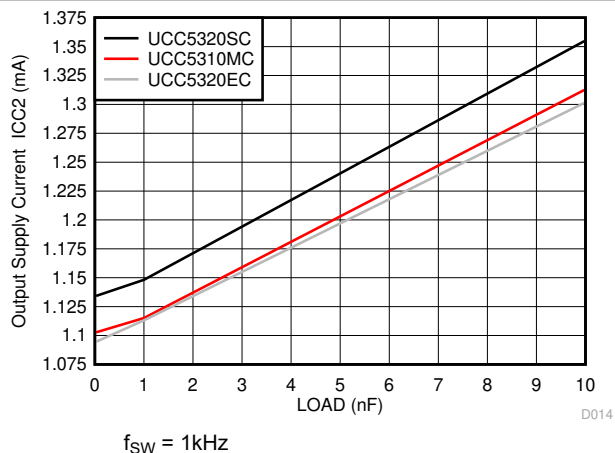
图 6-22. I_{CC2} 电源电流与负载电容间的关系
