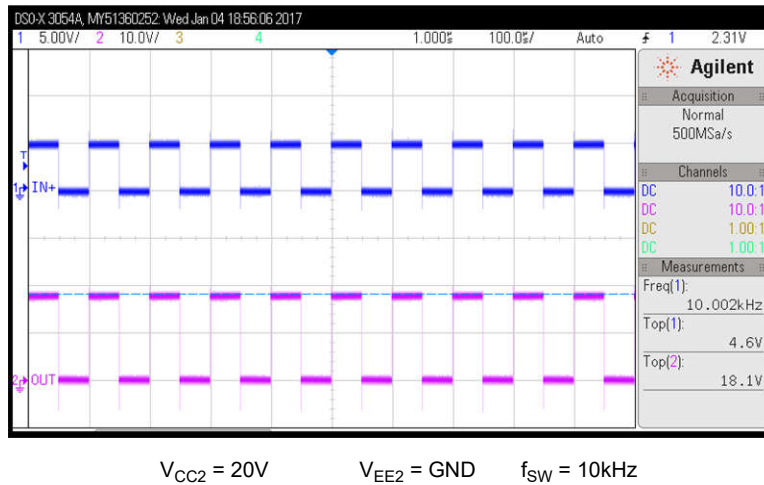
图 9-6. PWM 输入 和栅极电压波形
