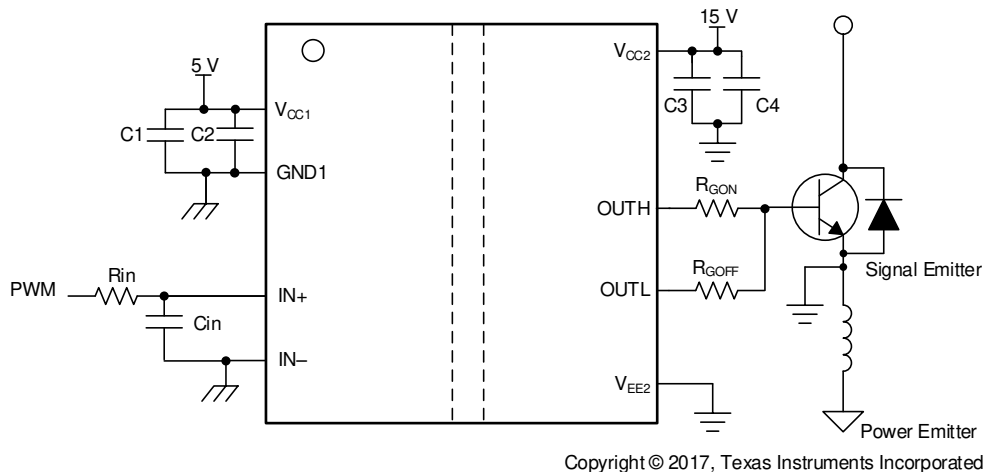
图 9-1. UCC53x0S 用于驱动 IGBT 的典型应用电路
