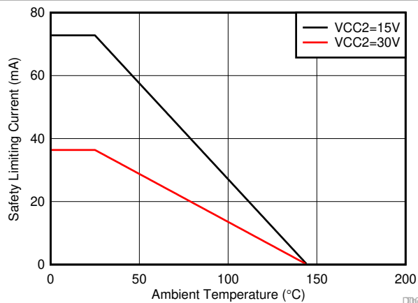
图 6-1. D 封装根据 VDE 标准限制电流的热降额曲线
