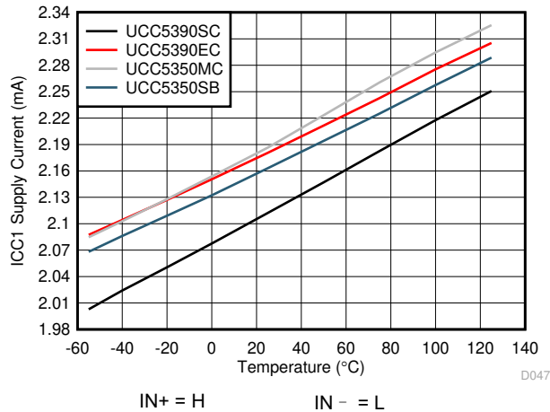
图 6-13. I_{CC1} 电源电流与温度间的关系
