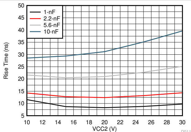
图 6-38. UCC5350SBD 上升时间与 C_L 和 V_{CC2} 间的关系
