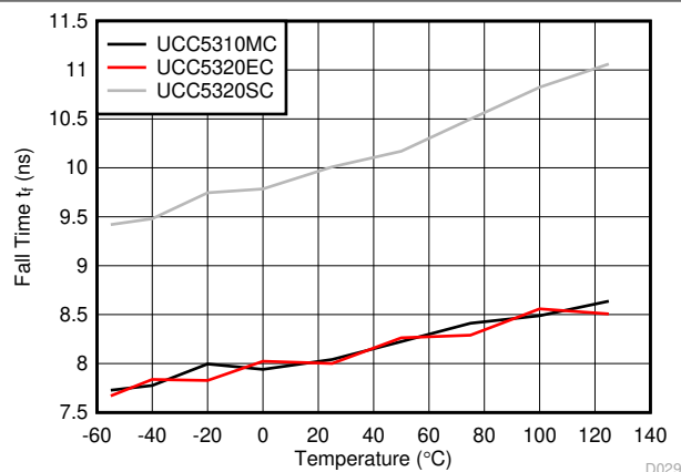
图 6-29. 下降时间与温度间的关系
