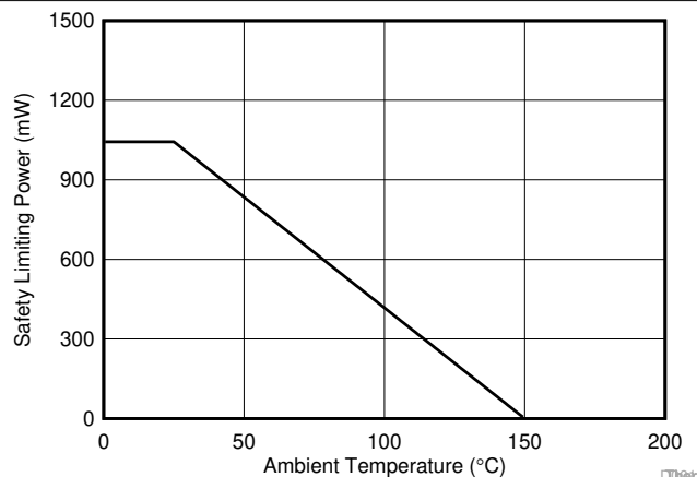
图 6-4. DWV 封装根据 VDE 标准限制功率的热降额曲线
