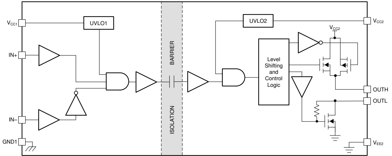
图 8-3. 功能方框图 — 分离输出 (UCC53x0S)
