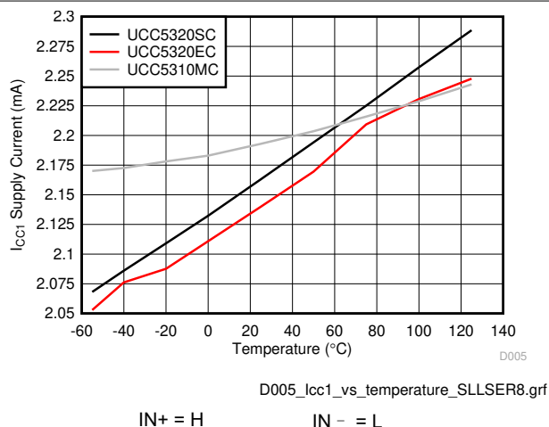
图 6-12. I_{CC1} 电源电流与温度间的关系
