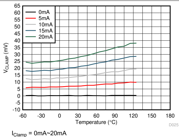
图 6-24. UCC5310M V_{CLAMP} 与温度间的关系
