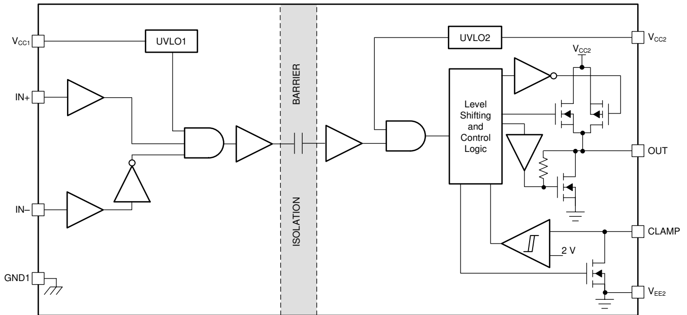
图 8-4. 功能方框图 — 米勒钳位 (UCC53x0M)
