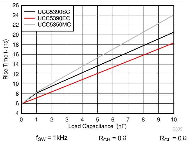
图 6-37. 上升时间与负载电容间的关系
