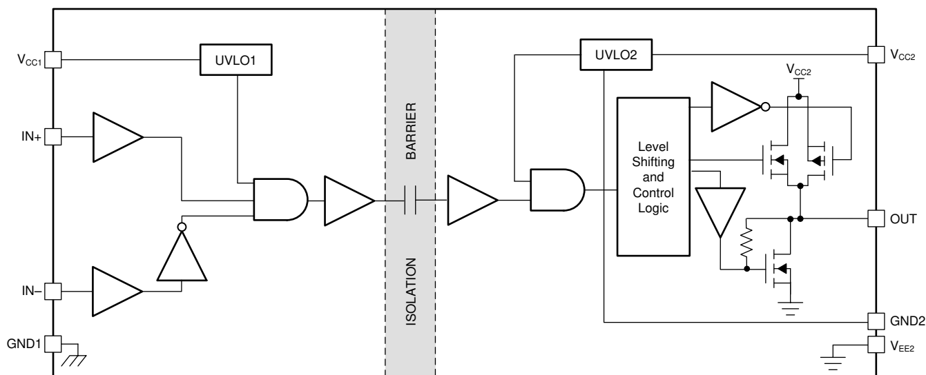
图 8-5. 功能方框图 — 以 GND2 为基准的 UVLO (UCC53x0E)
