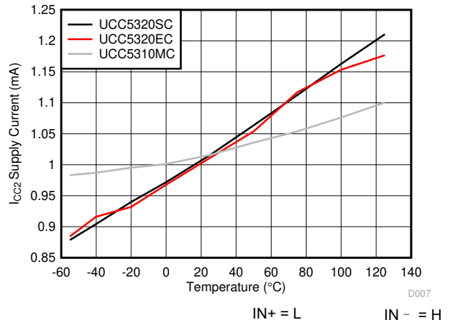
图 6-16. I_{CC2} 电源电流与温度间的关系
