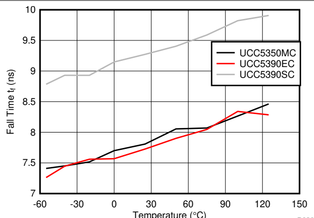
图 6-30. 下降时间与温度间的关系
