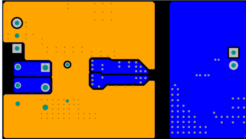
图 11-3. 底层布线和覆铜 (翻转)
