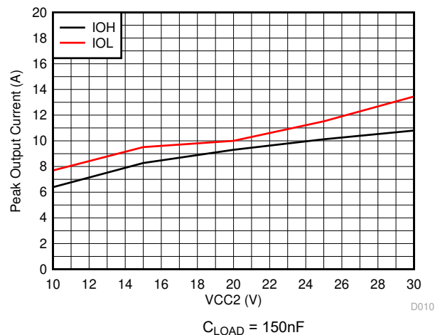
图 6-7. UCC5350SBD 输出高驱动电流与输出电压间的关系
