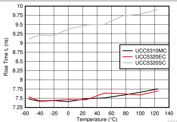
图 6-27. 上升时间与温度间的关系
