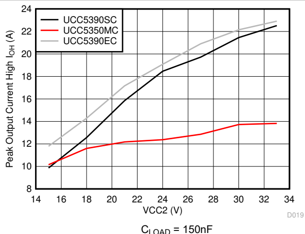
图 6-6. 输出高驱动电流与输出电压间的关系
