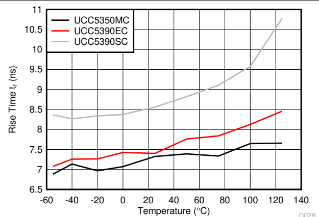
图 6-28. Rise Time vs Temperature
