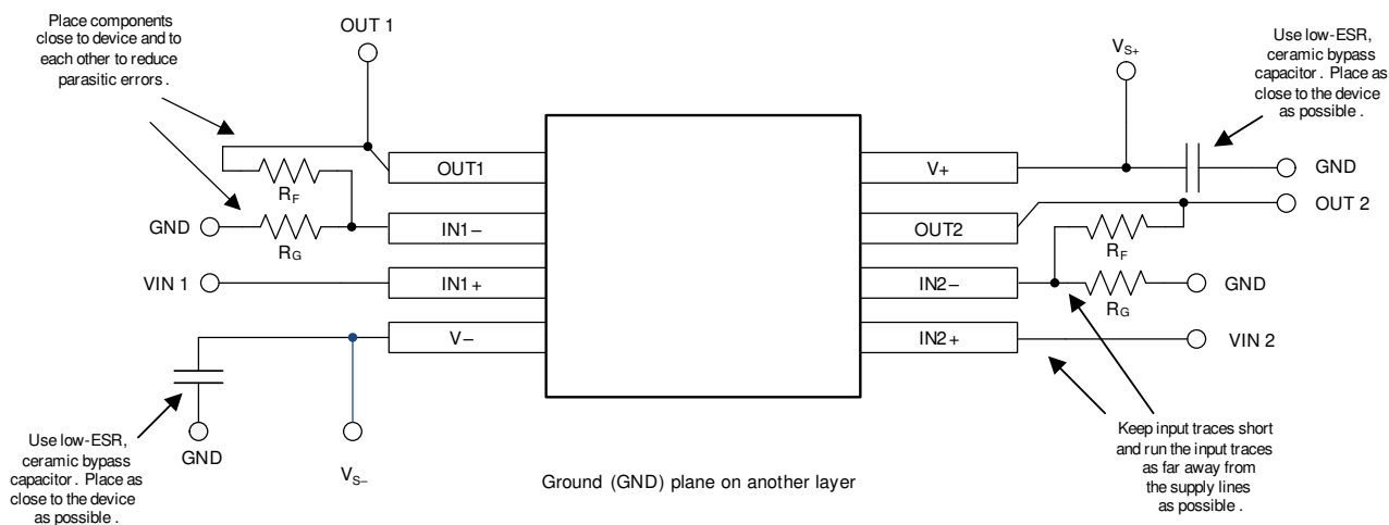
图 8-5. 布局示例
