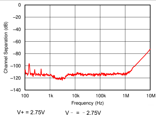
图 6-32. 通道隔离与频率间的关系
