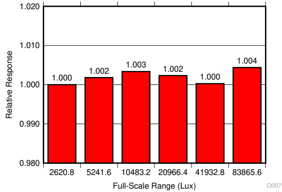
图 5-8. 满标量程匹配 (最高的 6 个量程)
