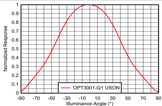
图 5-15. 归一化响应与照明角度间的关系
