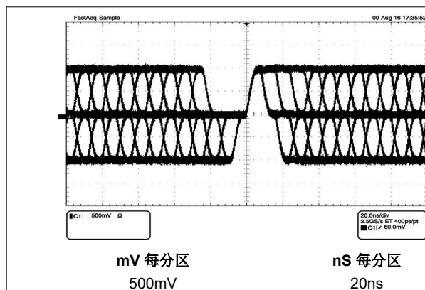
图 6-18. 100BASE-TX PMD 眼图波形
