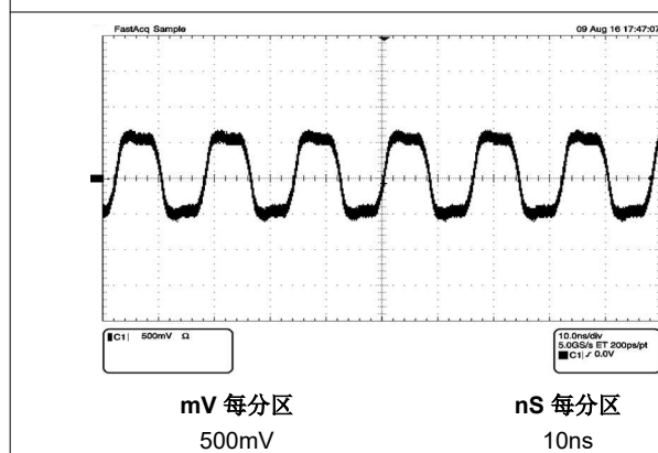
图 6-20. 100BASE-FX 波形
