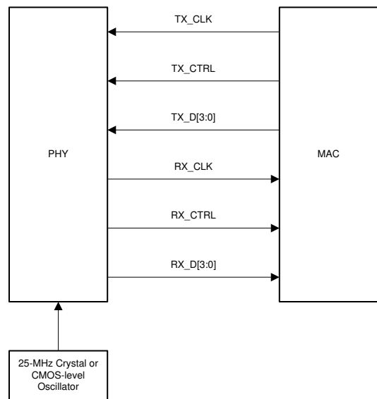
图 7-9. RGMII 信号
