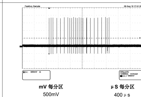
图 6-21. 自动协商快速链路脉冲波形
