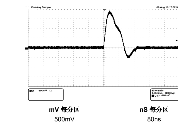
图 6-19. 10BASE-Te 链路脉冲波形
