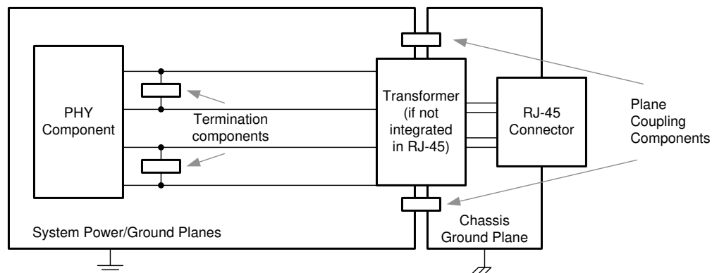
图 9-9. 布局示例
