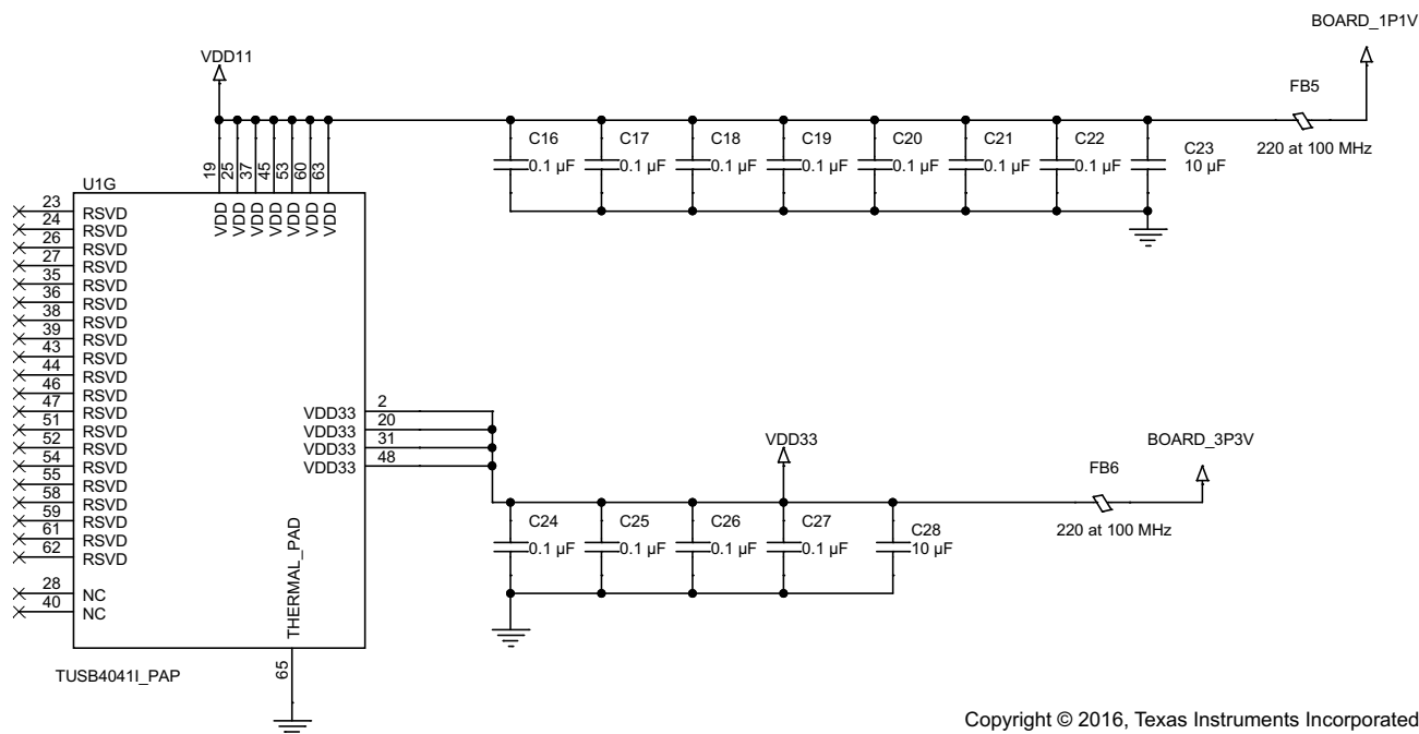
图 7-9. TUSB4041I-Q1 电源实现
