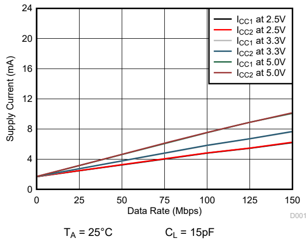
图 5-3. 电源电流与数据速率之间的关系 (15pF 负载)
