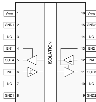
图 4-2. DWW 封装 16 引脚 (SOIC)顶视图
