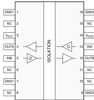
图 4-1. DW 封装 16 引脚 (SOIC)顶视图
