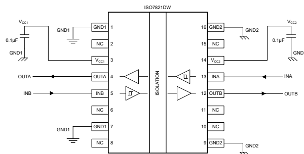
图 8-2. 典型 ISO7821 电路组装
