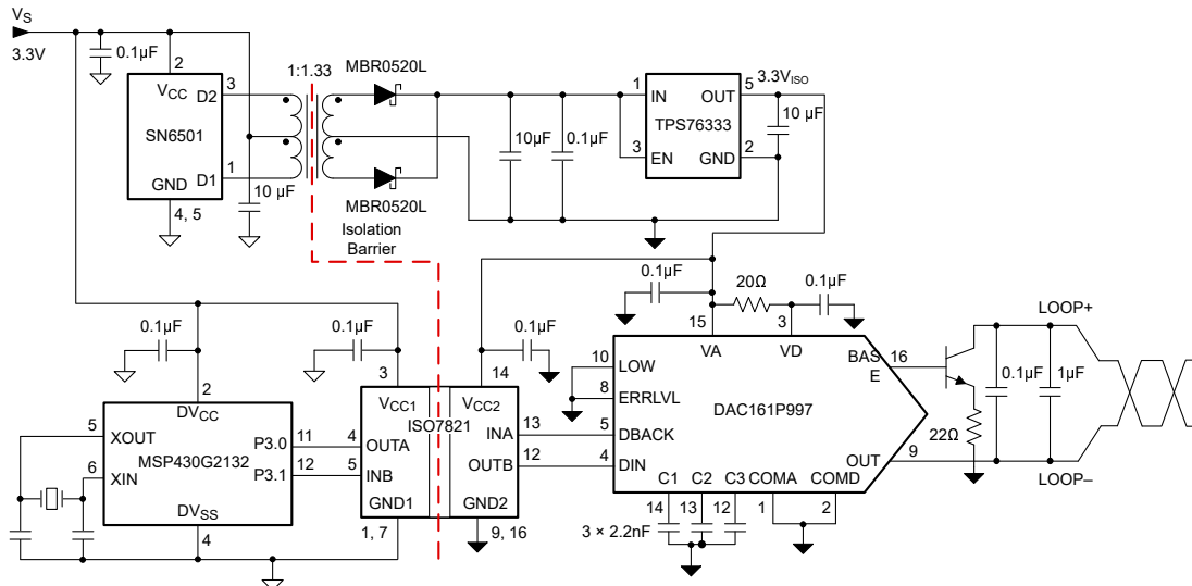
图 8-1. 隔离式 4mA 至 20mA 电流环路
