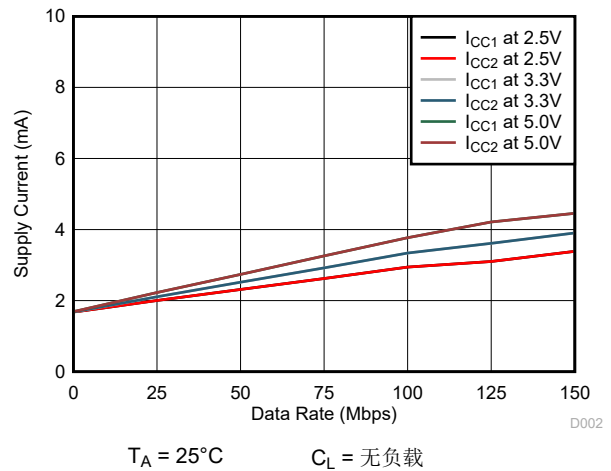
图 5-4. 电源电流与数据速率之间的关系 (无负载)
