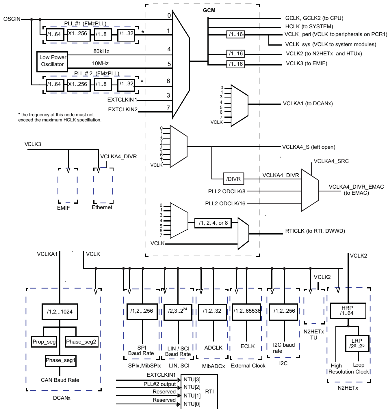
图 5-7. 器件时钟域
