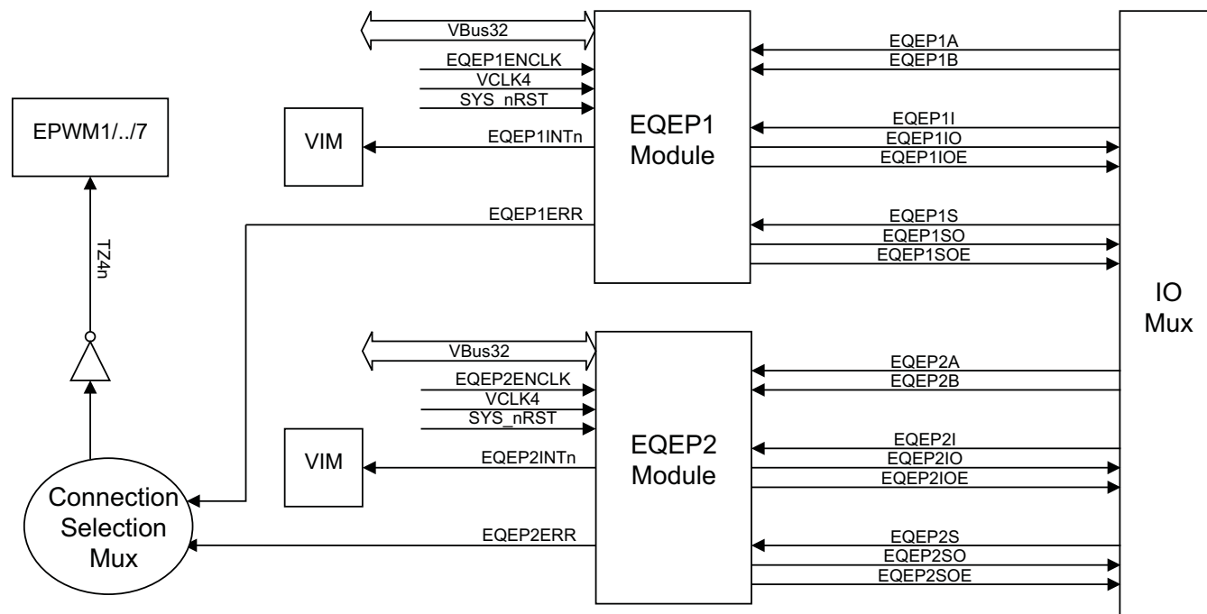
图 6-4. eOEP 模块互连
