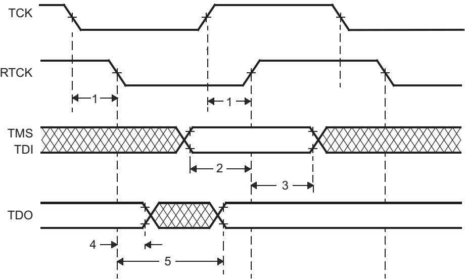
图 5-20. JTAG 时序
