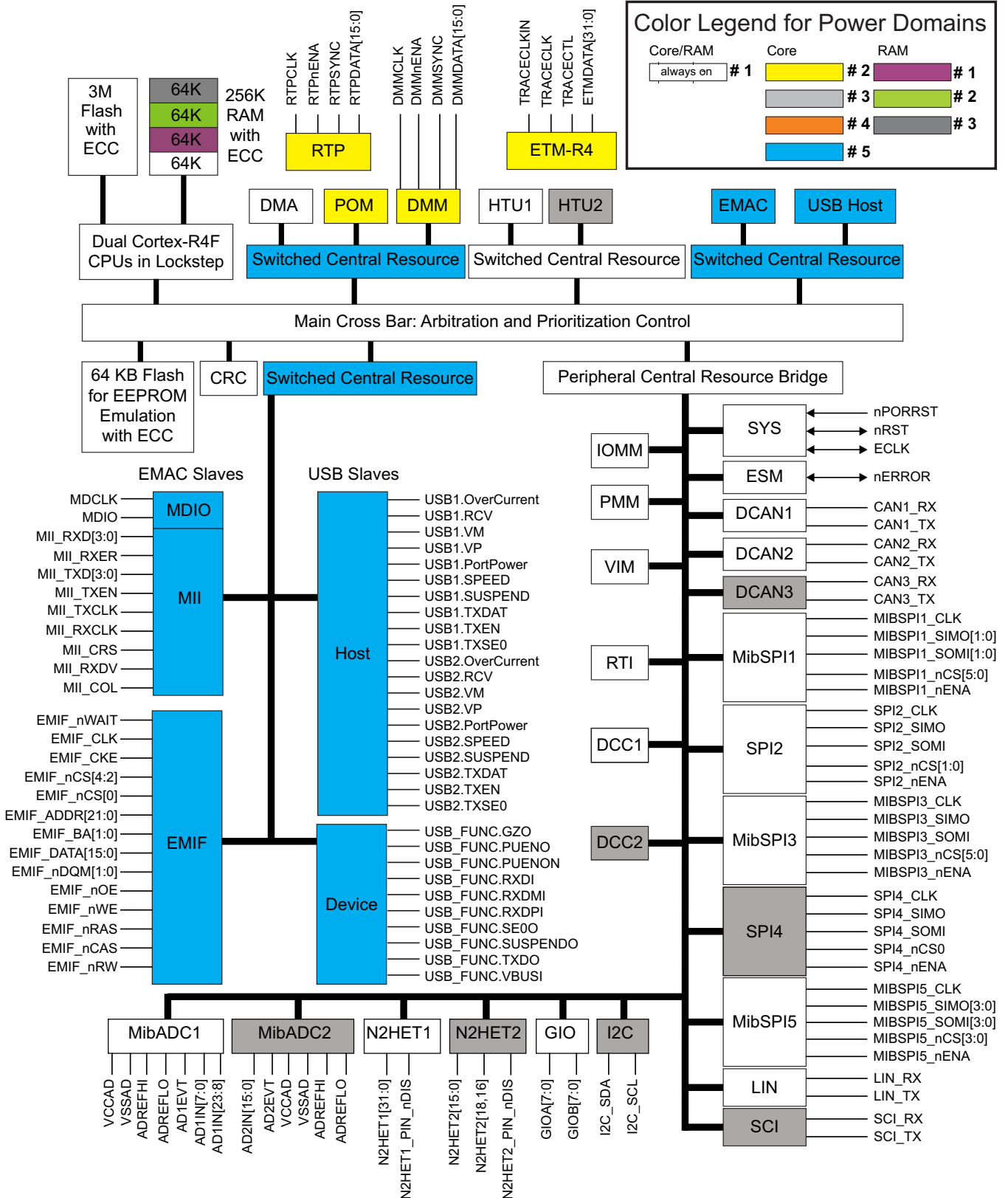
图 1-1. 功能方框图
