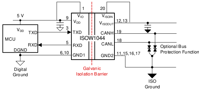
图 3-2. 采用小型 ISOW1044 的隔离信号和电源
