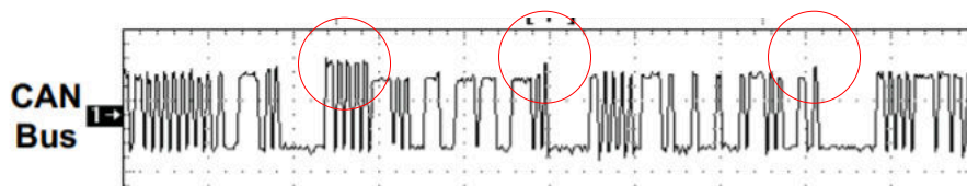
图 14-1. 差分 CAN 总线电压在某些位上显示更高的电压
