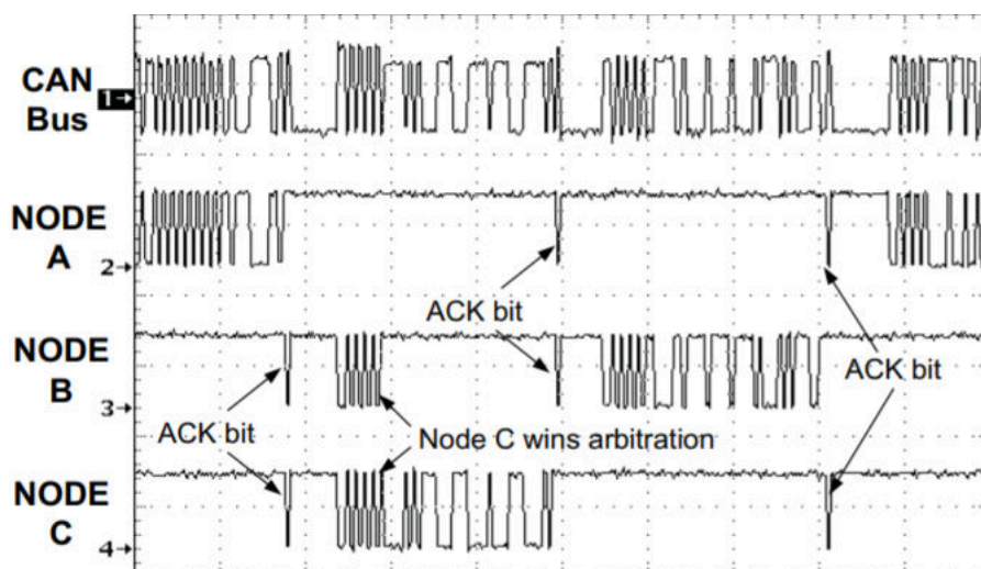
图 14-3. CAN 总线波形描述了为什么有些位的幅度更大
