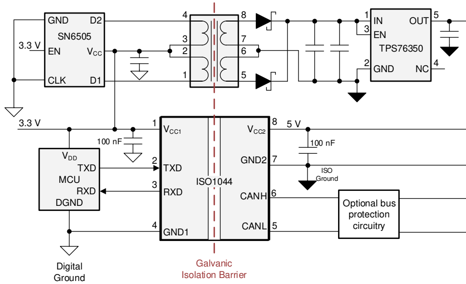
图 3-1. 采用推挽式拓扑的隔离式电源产生
