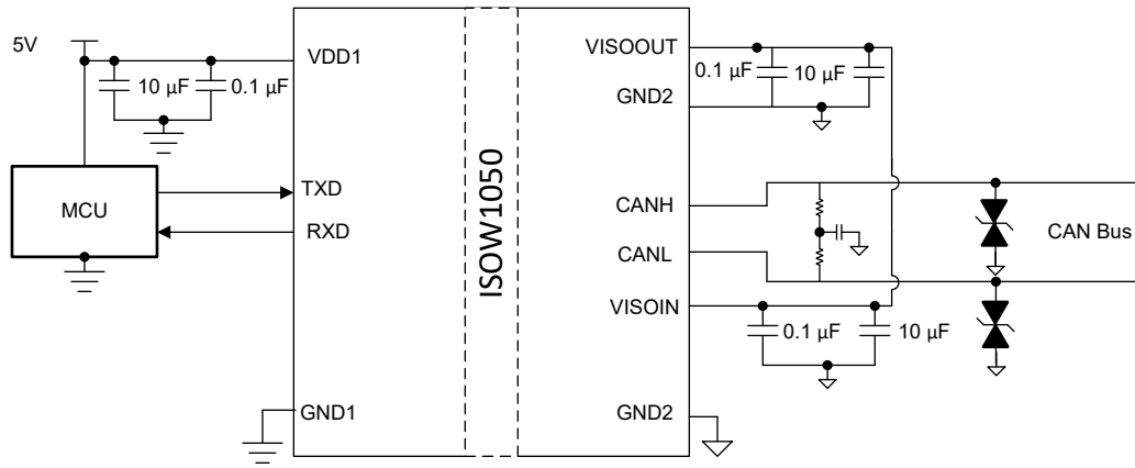
图 3-3. 采用 ISOW1050 进行信号与电源隔离以实现出色的 EMC
