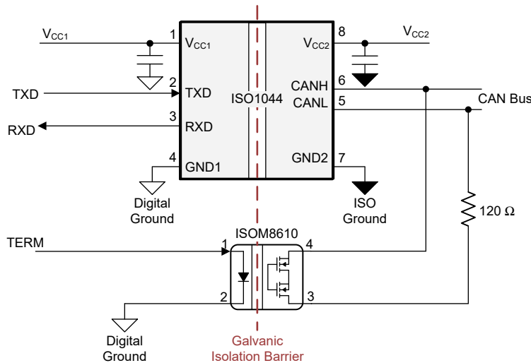
图 4-2. 使用 ISOM8610 的软件控制端接
