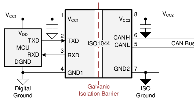
图 2-1. 集成式超小型封装隔离式 CAN 器件 ISO1044
