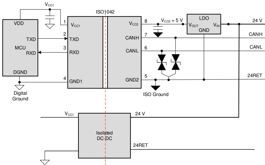
图 3-4. DeviceNet 应用原理图
