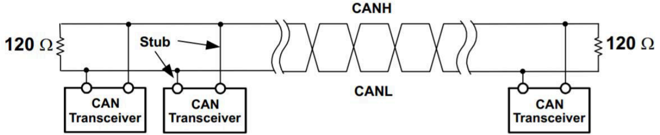
图 13-1. 显示残桩的 CAN 网络
