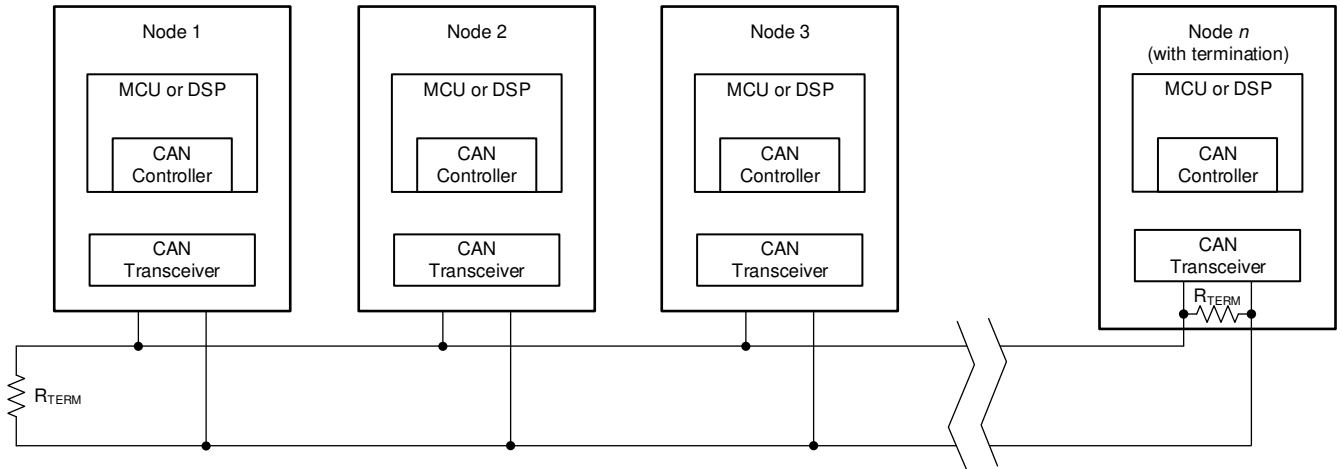
图 4-1. 典型 CAN 总线网络
