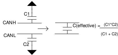
图 11-1. CAN 总线电容
