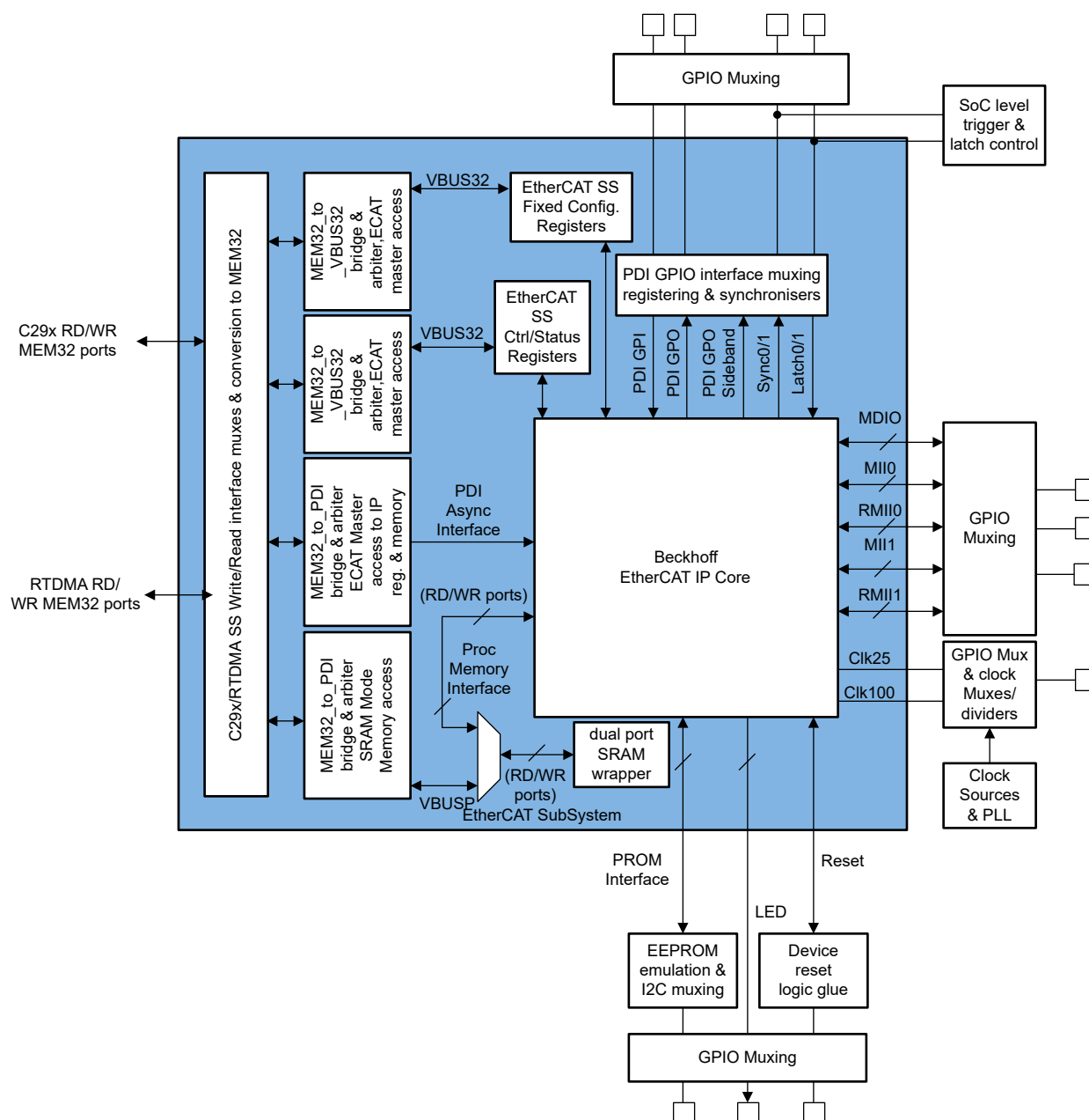
Figure 31-9. ESCSS Wrapper
