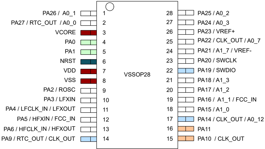
图 6-6. 28 引脚 DGS28 (VSSOP) (顶视图)
