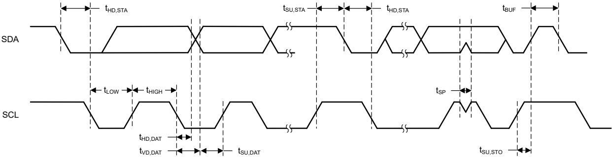
图 7-3. I2C 时序图
