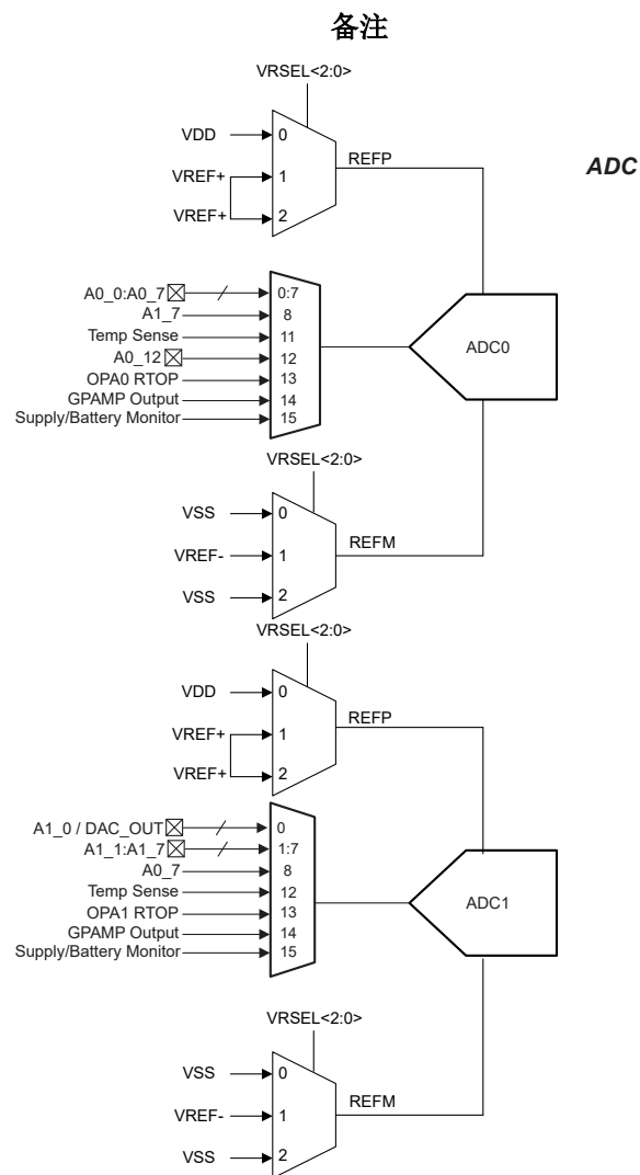
图 8-3. 器件模拟连接 ( ADC0 和 ADC1 )
