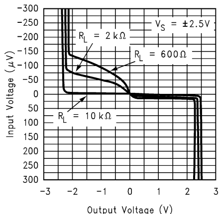
图 7-19. 输入电压与输出电压之间的关系
