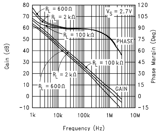
图 7-20. 开环频率响应
