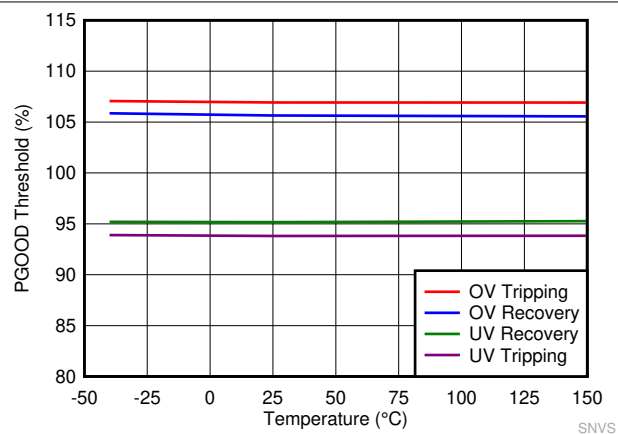
图 7-7. PGOOD 阈值
