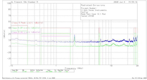
图 9-36. 辐射 EMI Red 与 CISPR25 限值
