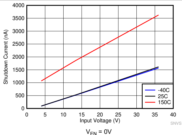
图 7-2. 关断电源电流
