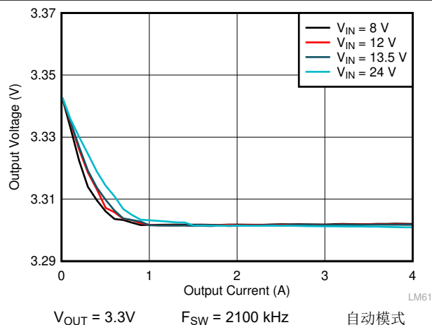
图 9-9. LMQ62440-Q1 负载和线性调整率
