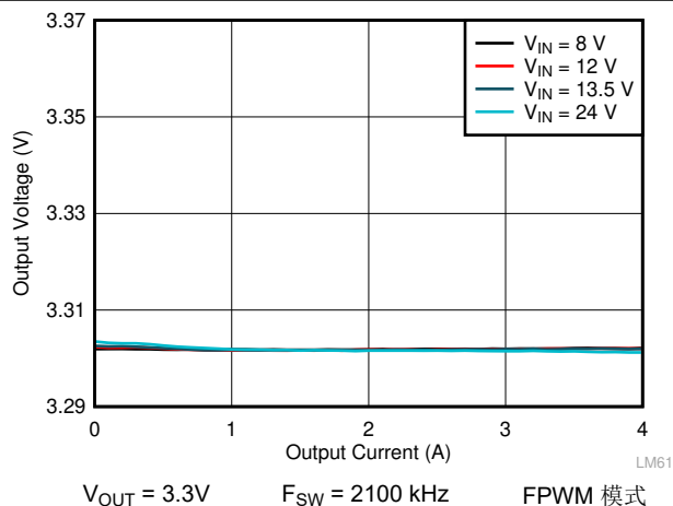
图 9-10. LMQ62440-Q1 负载和线性调整率
