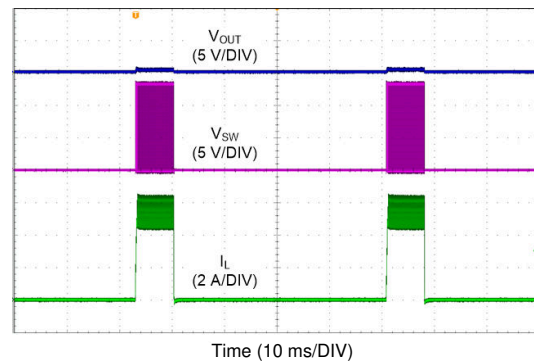
图 9-22. LMQ62440-Q1 短路性能
