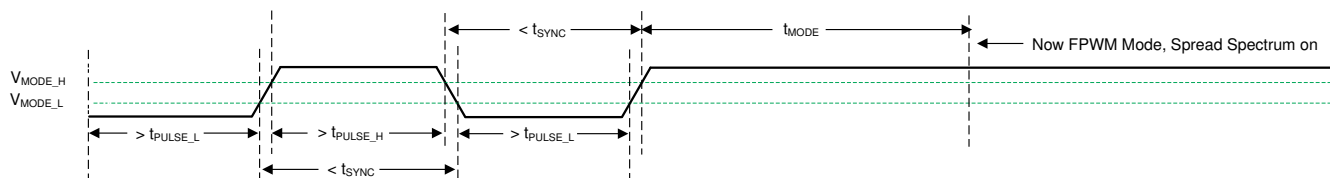
图 8-11. 从 SYNC 模式转换到 FPWM 模式
