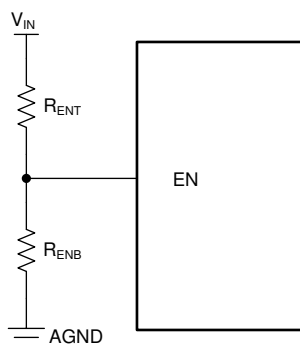
图 9-4. 使用 EN 的 UVLO
