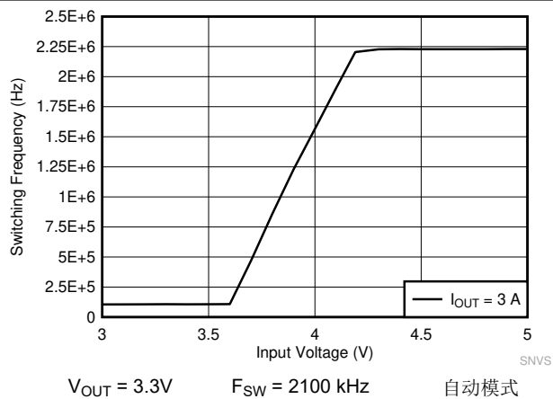
图 9-15. LMQ62440-Q1 频率压降曲线
