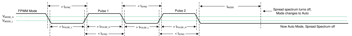
图 8-8. 从 FPWM 模式转换到自动模式时禁用展频
