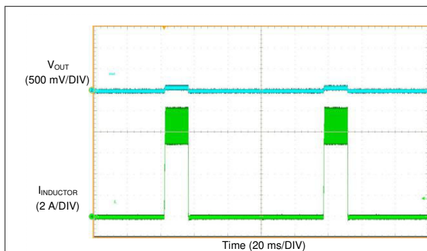
图 8-20. 断续期间的电感器电流突发
