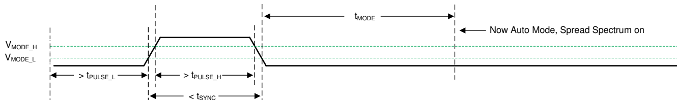
图 8-10. 从 SYNC 模式转换到自动模式
