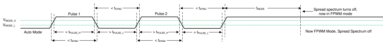
图 8-9. 从自动模式转换到 FPWM 模式时禁用展频
