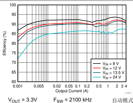
图 9-5. LMQ62440-Q1 效率
