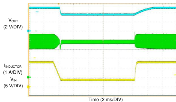
图 8-17. 从压降中恢复 ( V_{OUT} = 5V , I_{OUT} = 4A , V_{IN} = 13.5V 至 4V 至 13.5V )
