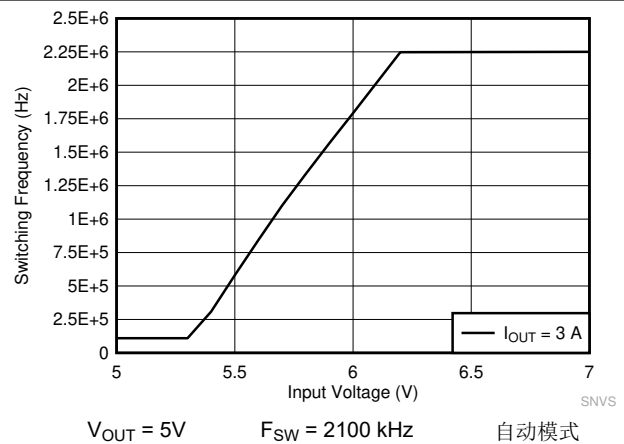
图 9-16. LMQ62440-Q1 频率压降曲线
