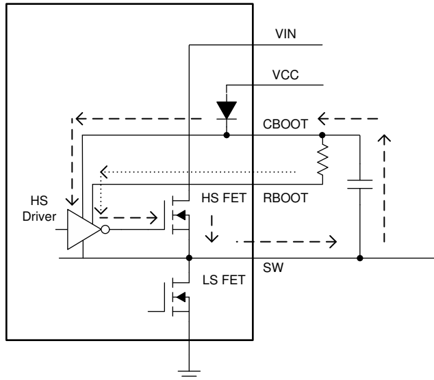
图 8-14. 显示 RBOOT 功能的简化电路
