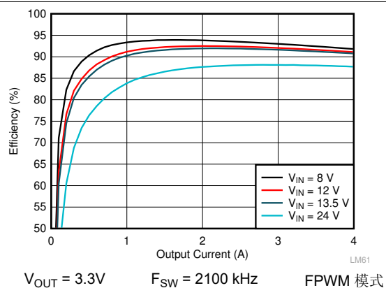
图 9-6. LMQ62440-Q1 效率
