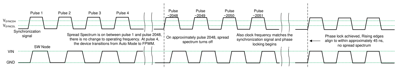
图 8-12. 同步过程
