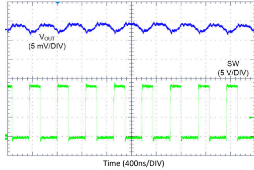
图 9-18. LMQ62440-Q1 开关波形和 V_{OUT} 纹波
