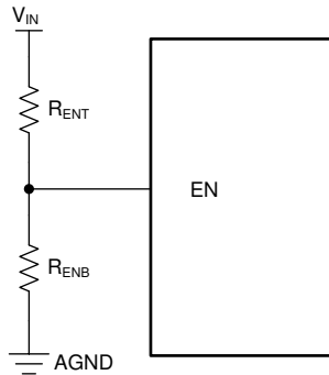
图 8-1. V_{IN} /UVLO 使用 EN 引脚
