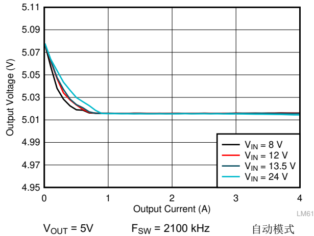
图 9-11. LMQ62440-Q1 负载和线性调整率
