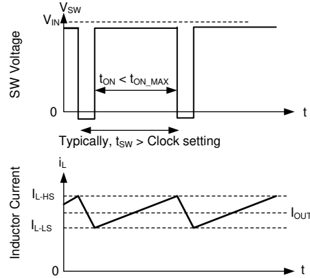
图 8-19. 电流限值波形
