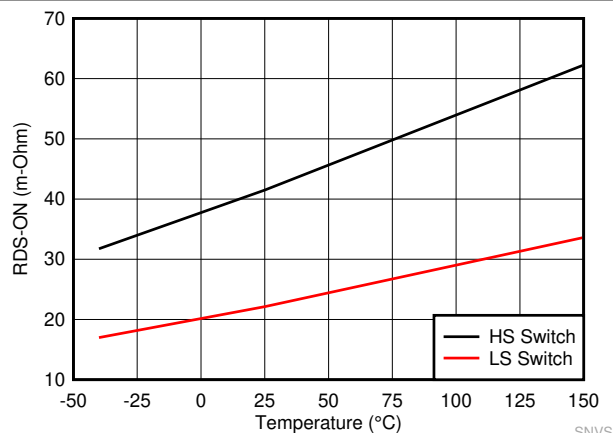
图 7-5. 高侧和低侧开关 R_{DS-ON}
