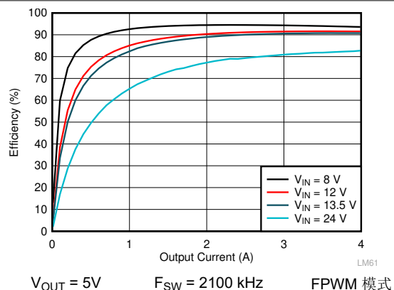
图 9-8. LMQ62440-Q1 效率
