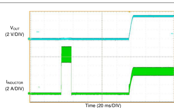
图 8-21. 短路恢复
