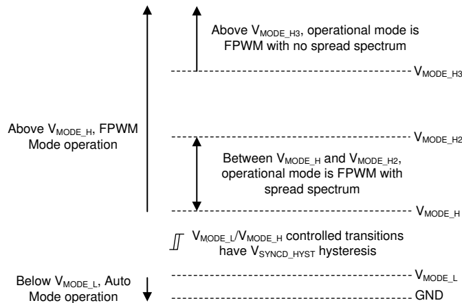
图 8-2. 电平相关模式选择设置
