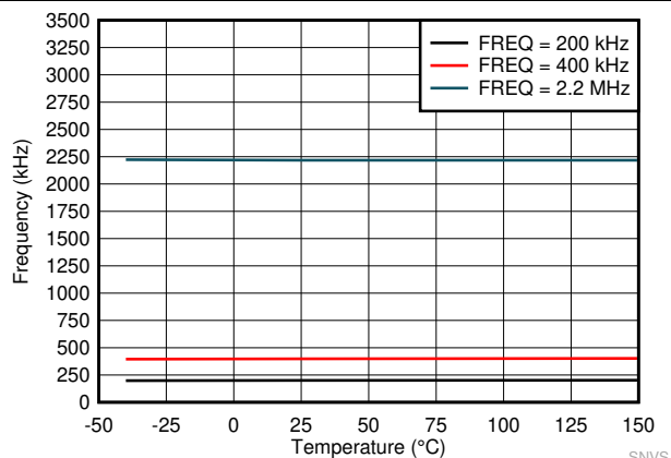
图 7-4. 开关频率
