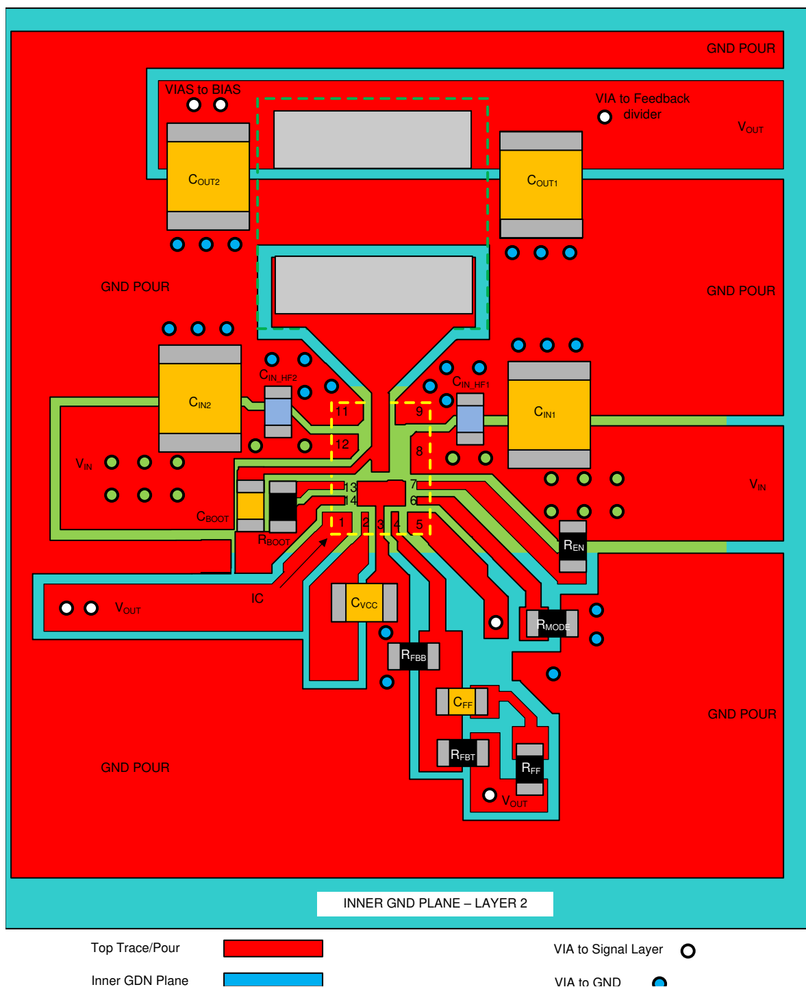
图 11-2. 布局示例
