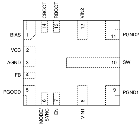
图 6-1. RJR 封装 14 引脚 VQFN-HR 顶视图
