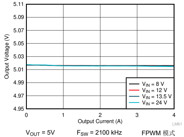
图 9-12. LMQ62440-Q1 负载和线性调整率
