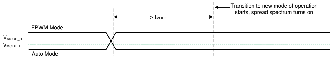
图 8-5. 自动模式和 FPWM 模式之间的转换
