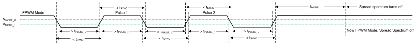
图 8-6. 在 FPWM 模式下禁用展频
