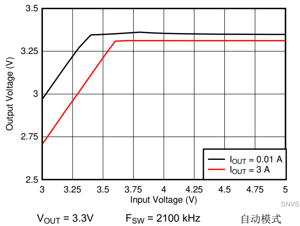
图 9-13. LMQ62440-Q1 压降曲线
