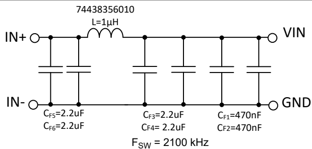
图 9-41. 推荐的输入 EMI 滤波器
