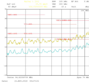
图 9-35. 传导 EMI 与 CISPR25 限值 (黄色：峰值信号，蓝色：平均信号)
