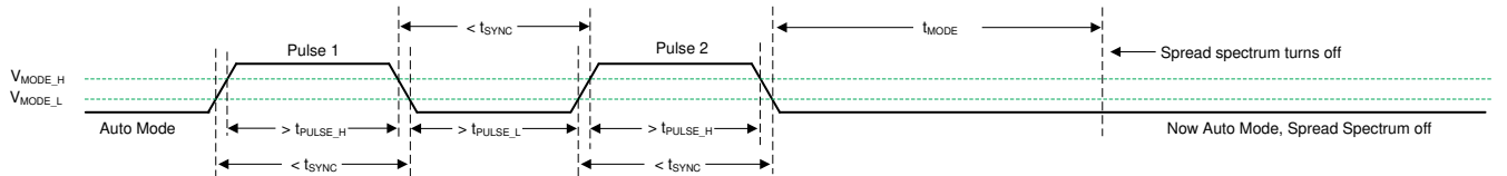
图 8-7. 在自动模式下禁用展频
