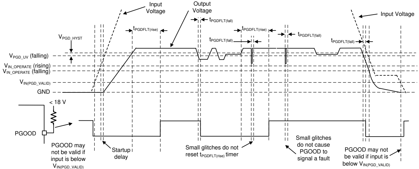
图 8-13. PGOOD 时序图 (不包括 OV 事件)
