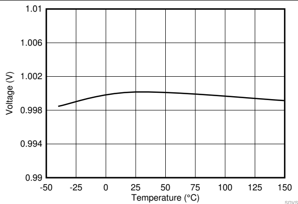
图 7-3. 反馈电压
