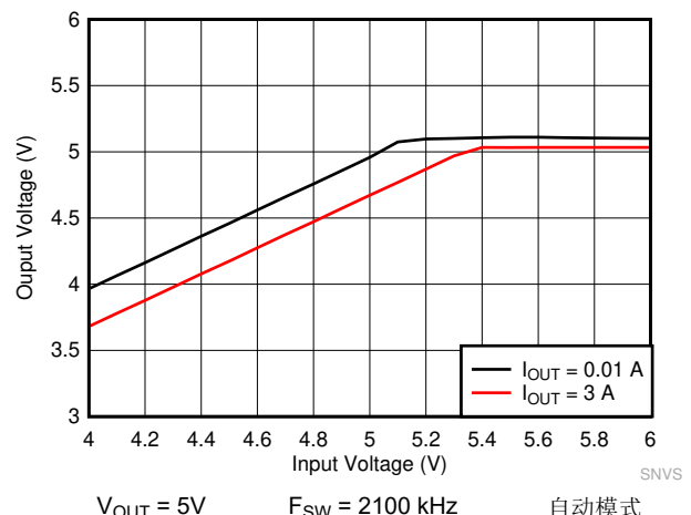
图 9-14. LMQ62440-Q1 压降曲线
