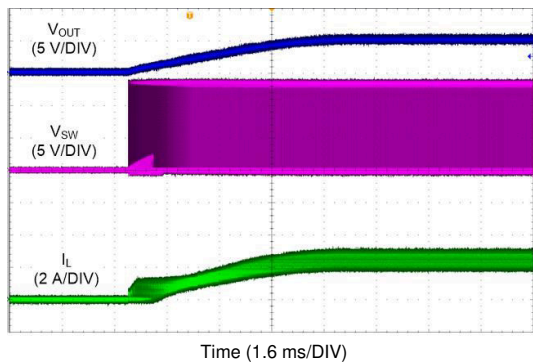
图 9-19. LMQ62440-Q1 在 3.25A 时启动
