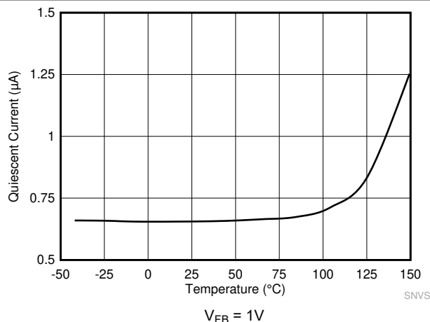
图 7-1. 非开关输入电源电流
