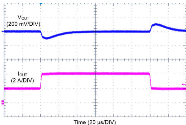
图 9-23. LMQ62440-Q1 负载瞬态
