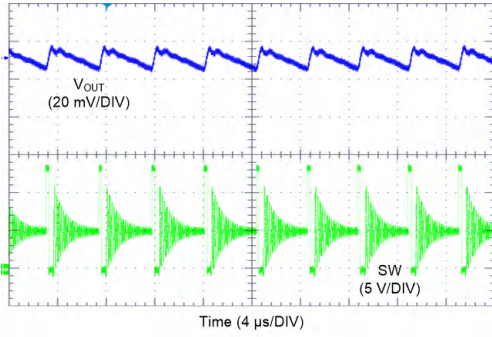
图 9-17. LMQ62440-Q1 开关波形和 V_{OUT} 纹波
