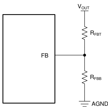
图 8-18. 设置可调版本的输出电压
