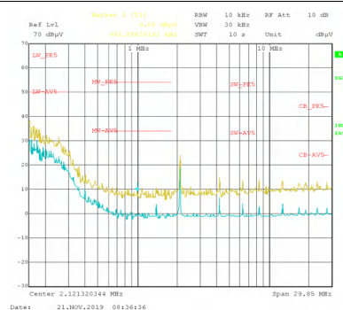
图 9-32. 辐射 EMI 对数水平与 CISPR25 限值
