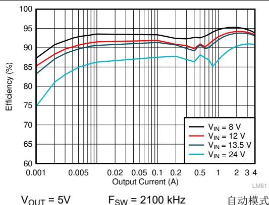
图 9-7. LMQ62440-Q1 效率
