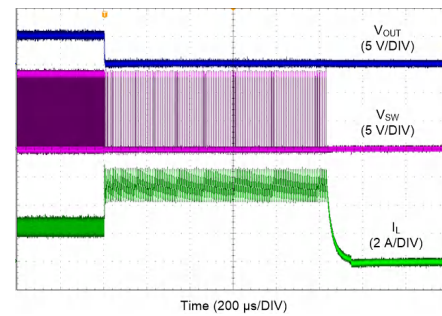
图 9-18. LMQ62440-Q1 开关波形和 V_{OUT} 纹波
