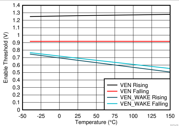
图 7-6. 使能阈值
