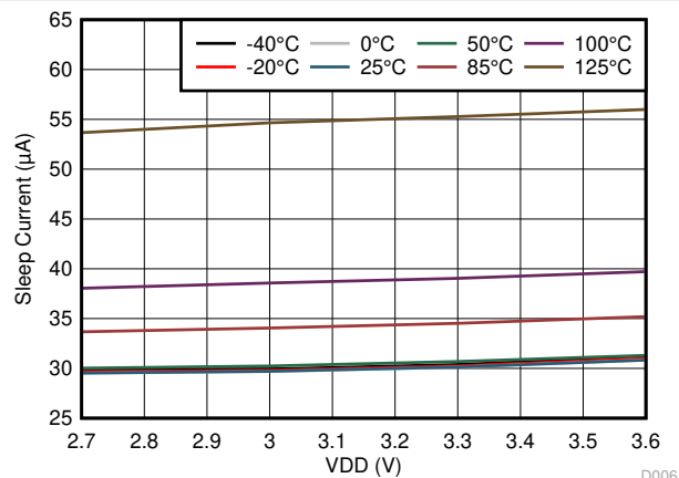
图 6-5. 睡眠模式 IDD 与 VDD 间的关系
