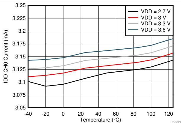
图 6-2. 活动模式 IDD 与温度间的关系
