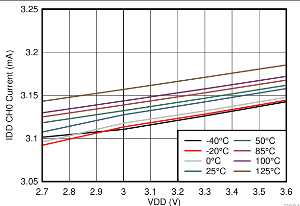
图 6-3. 活动模式 IDD 与 VDD 间的关系
