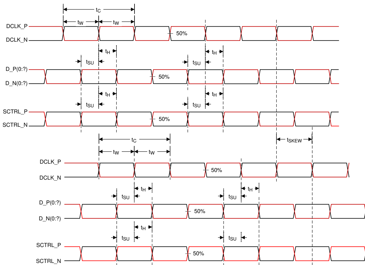
图 5-6. Timing Requirements
