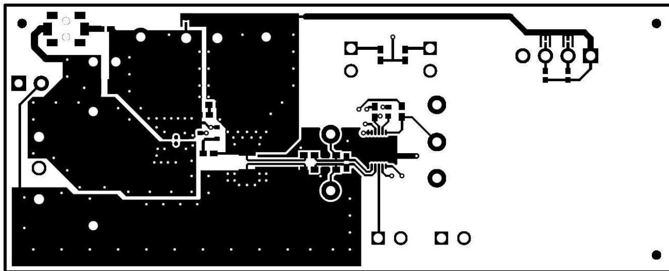
Figure 19. Top Layer
