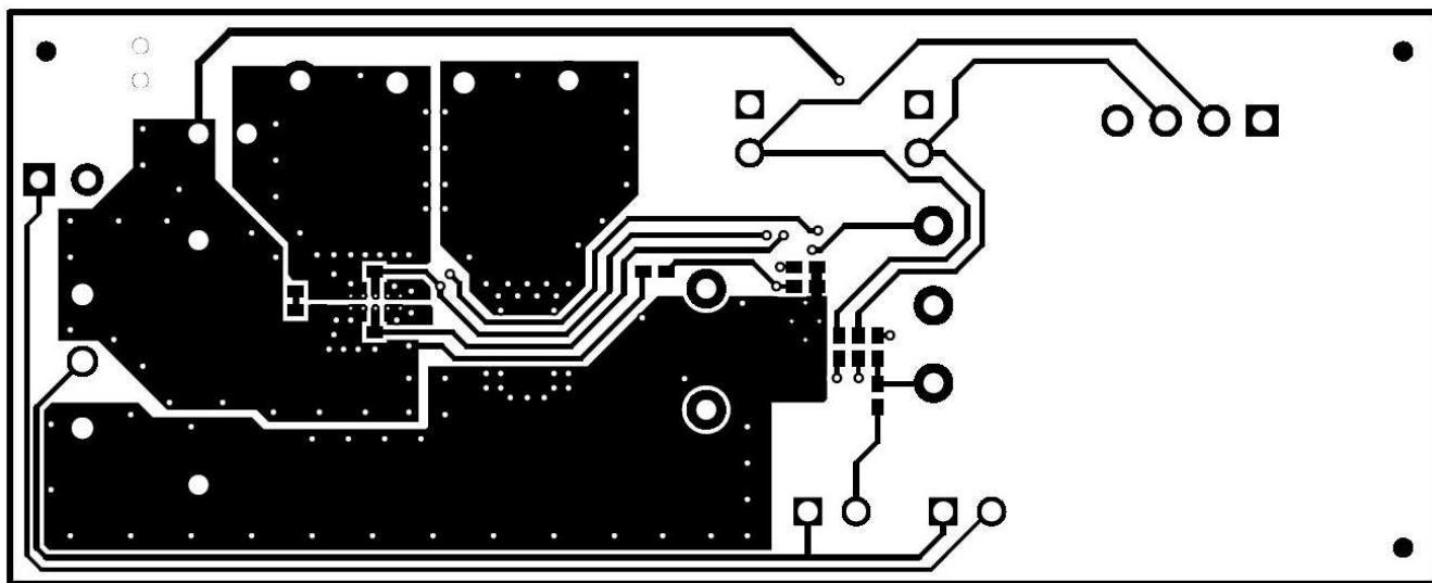
Figure 20. Bottom Layer
