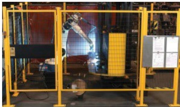
图 6. 带有物理安全笼的机械臂。
