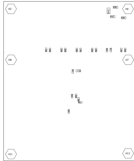
图 4-3. TPS1685EVM 电路板：底层装配图
