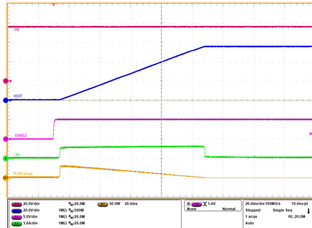
图 3-3. 使用 ENABLE 的 TPS1685 电子保险丝启动曲线 ( V_{IN} = 54\text{V} , EN 从 0V 升高至 5V, C_{OUT} = 1\text{mF} , C_{DVRT} = 82\text{nF} )
