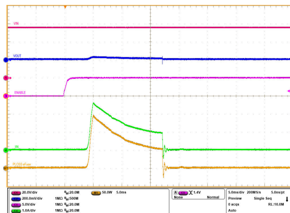
图 3-4. TPS1685 电子保险丝的上电至输出短路响应 ( V_{IN} = 54V , EN 从 0V 升高至 5V , OUT 短接至 PGND )
