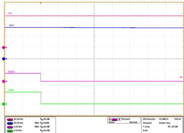
图 3-12. 在 TPS1685 电子保险丝上禁用 QOD ( V_{IN} = 54V , C_{OUT} = 1mF , EN 下拉至 0V)
