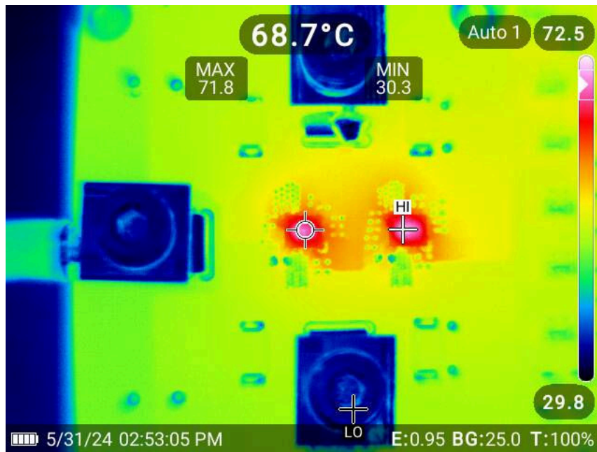
图 3-13. TPS1685EVM 的热性能 ( V_{IN} = 54V ， I_{OUT} = 40A ， T_A = 30^{\circ}C ，无外部气流)
