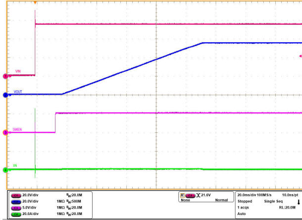
图 3-2. TPS1685 电子保险丝热插拔曲线 ( V_{IN} 从 0V 升高至 54V, C_{OUT} = 1\text{mF} , C_{DVRT} = 82\text{nF} )
