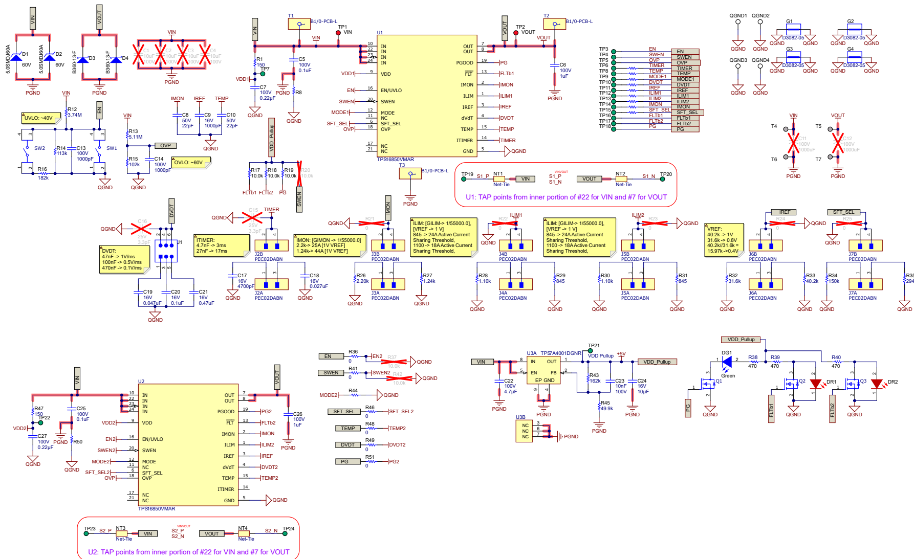
图 4-1. TPS1685EVM 保险丝评估板原理图
