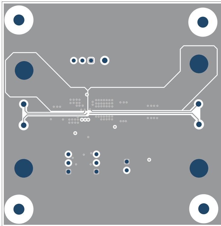
图 3-3. 底面布局
