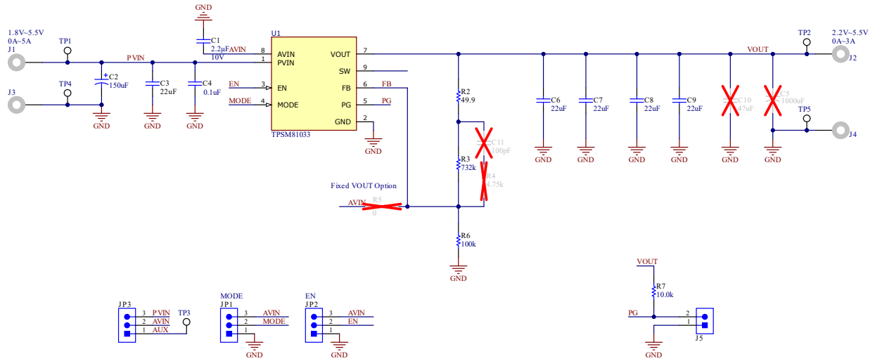
图 3-1. 原理图
