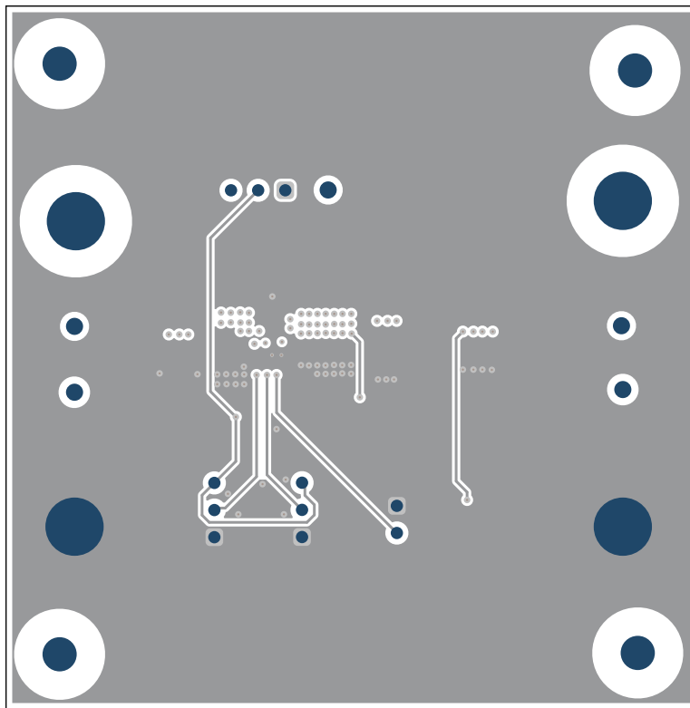
图 3-5. 内层 2 布局
