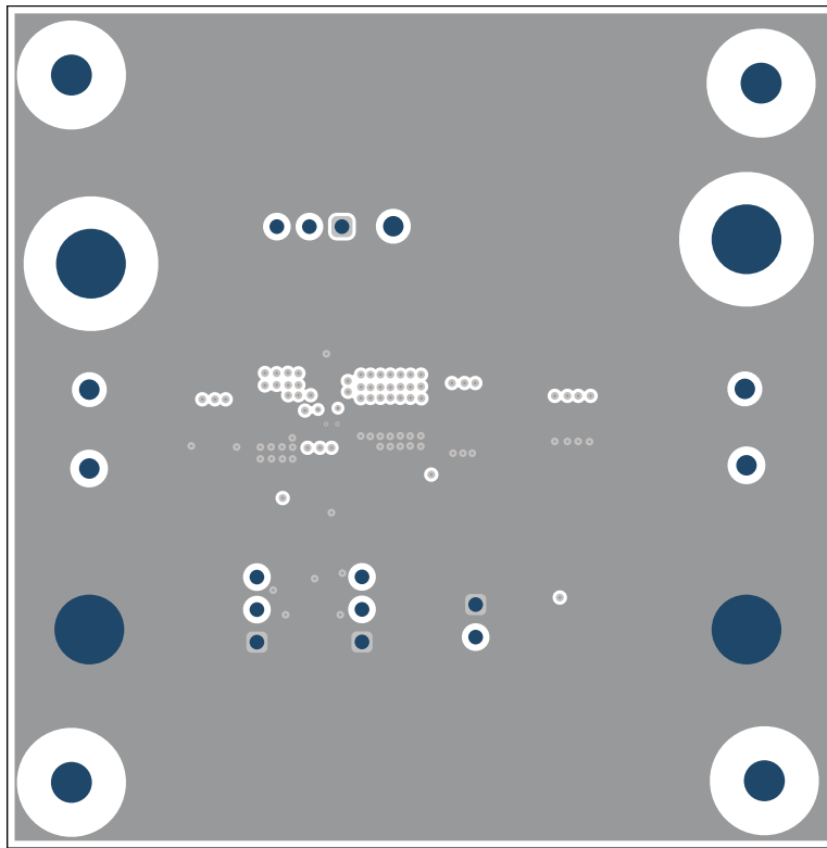
图 3-4. 内层 1 布局
