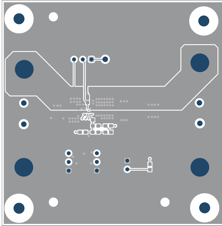
图 3-2. 顶面布局
