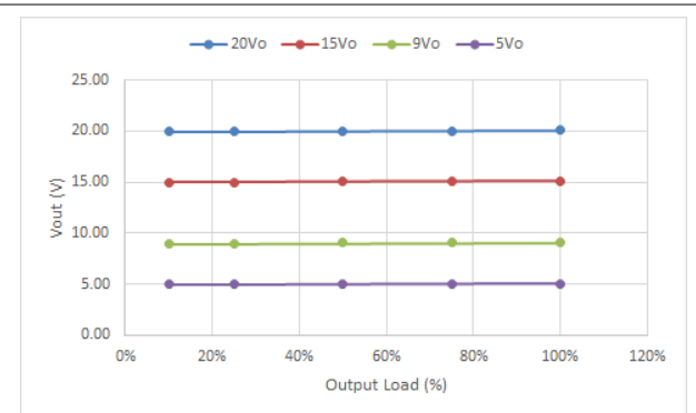
图 3-7. V_{OUT} 与输出电流间的关系
