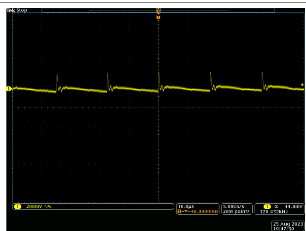
图 3-28. V_{OUT} = 5V 时的典型纹波电压
