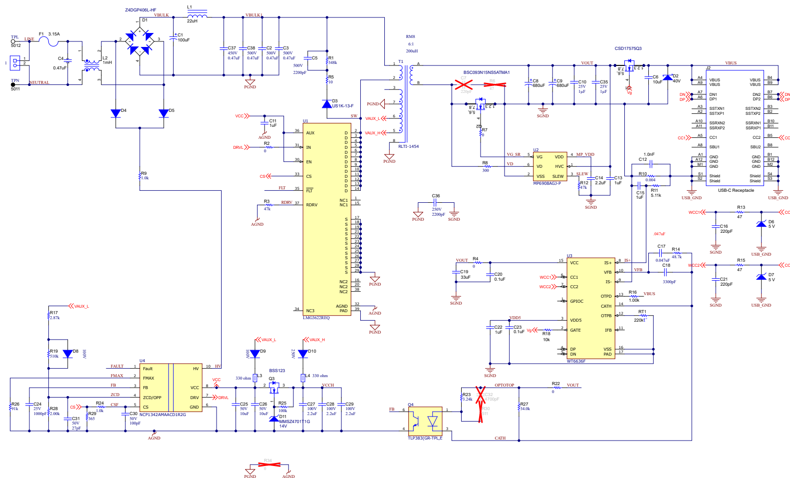
图 4-1. LMG3622EVM-082 原理图
