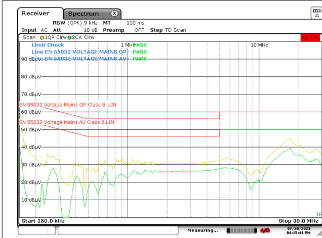
图 3-34. V_{IN} = 115V_{RMS} , V_{OUT} = 20V , 负载 = 3.25A (输出未接地至 LISN 地)
