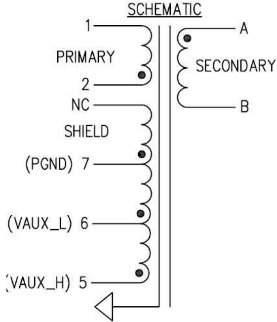
图 4-4. 变压器原理图
