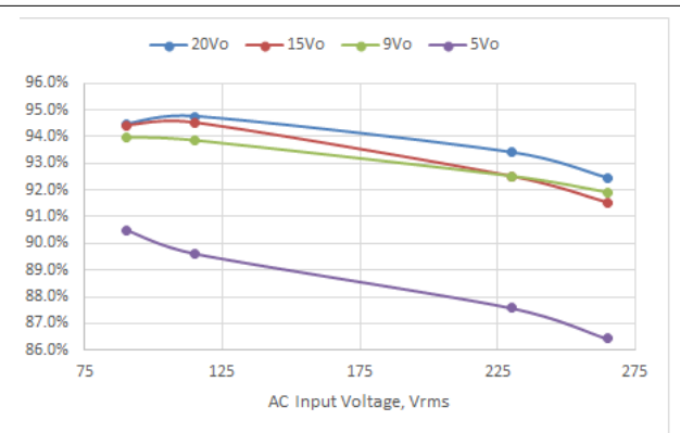
图 3-5. 50% 负载效率与输入电压
