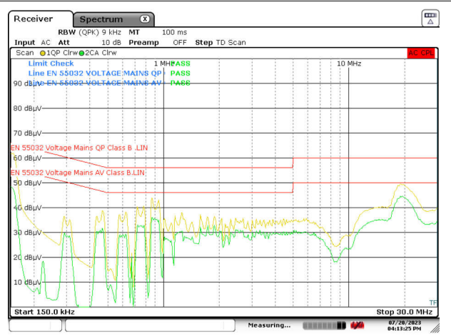
图 3-35. V_{IN} = 230V_{RMS} , V_{OUT} = 20V , 负载 = 3.25A (输出未接地至 LISN 地)
