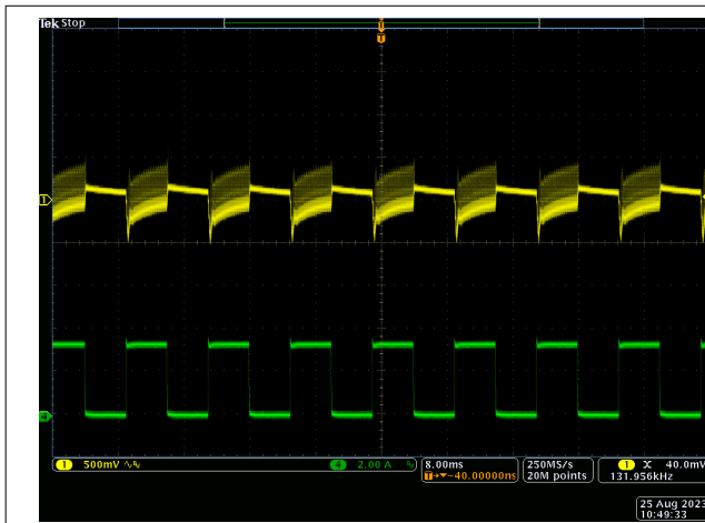
图 3-30. V_{OUT} = 20V 过冲/下冲 = 357mV/-619mV 条件下的负载瞬态响应
