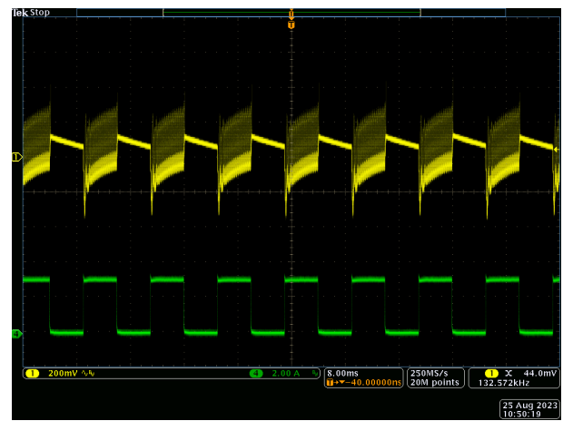
图 3-31. V_{OUT} = 15V 过冲/下冲 = 366mV/-562mV 条件下的瞬态响应
