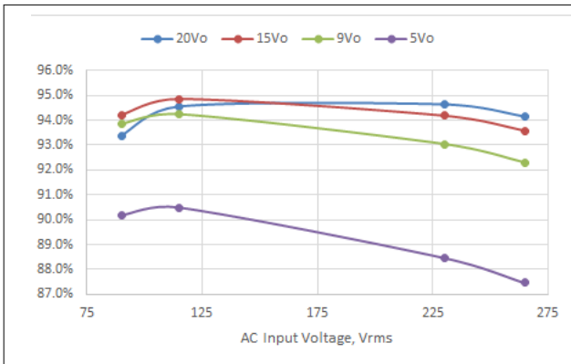
图 3-4. 满负载效率与输入电压
