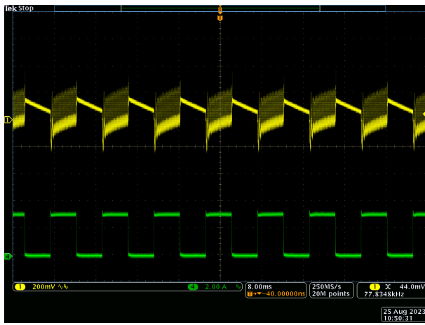
图 3-32. V_{OUT} = 9V 过冲/下冲= 326mV/-426mV 条件下的瞬态响应
