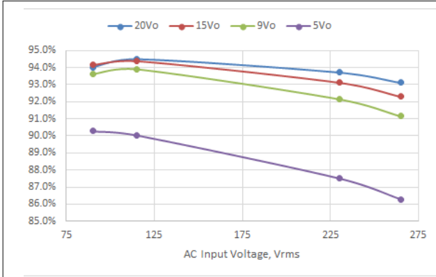
图 3-2. 4 点平均效率与输入电压
