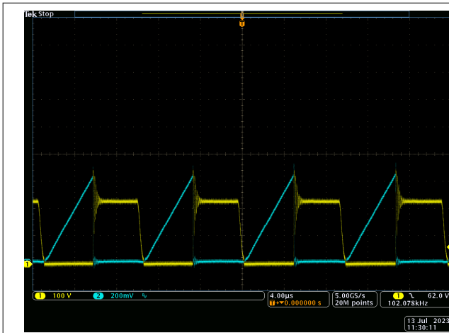
图 3-9. Vin = 90Vac , Vout = 20V
