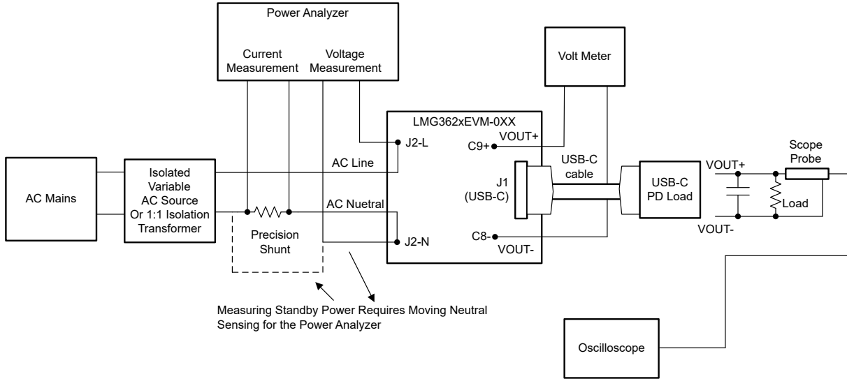
图 3-1. LMG3622EVM-082 测试设置图
