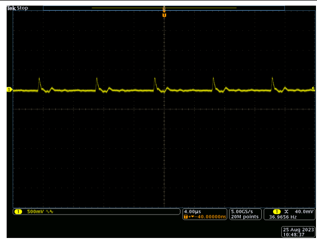
图 3-26. V_{OUT} = 15V 时的典型纹波电压
