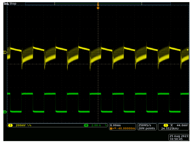
图 3-33. V_{OUT} = 5V 过冲/下冲= 326mV/-426mV 条件下的瞬态响应
