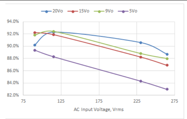
图 3-3. 10% 负载效率与输入电压
