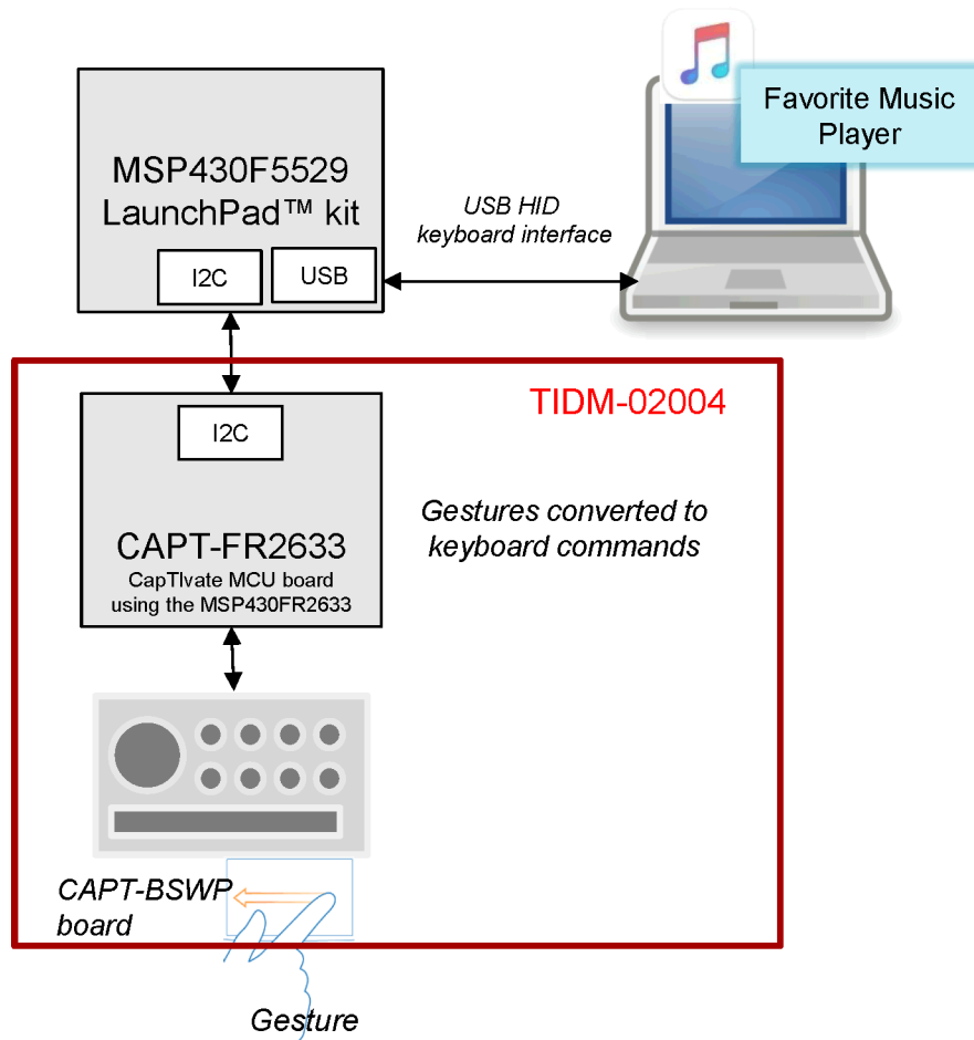
图 1. TIDM-02004 Block Diagram
